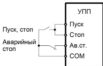
Рисунок 5 – Трехпроводная и двухпроводная схема управления
