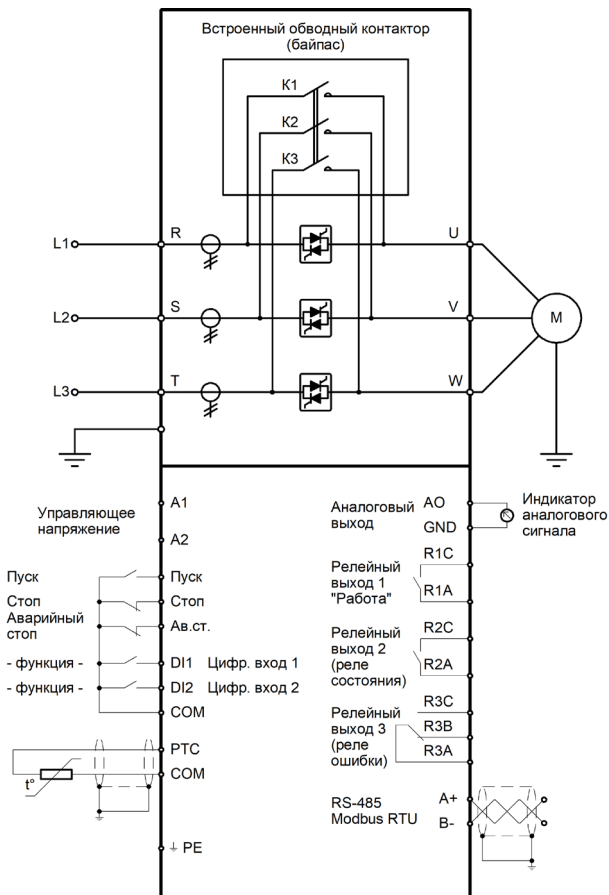
Рисунок 4 – Схема подключения клемм устройства плавного пуска серии SBIP
