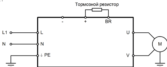
Рисунок 2 – Схема силовых подключений для моделей NCI-GY/PY-1B
