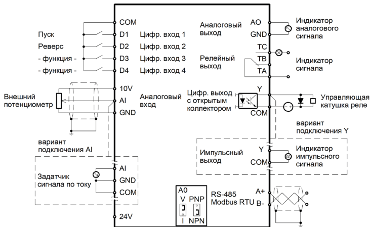
Рисунок 5 – Подключение управляющих клемм NC1
