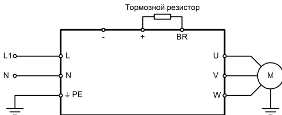
Рисунок 3 – Схема силовых подключений для моделей NCI-GY/PY-2B
