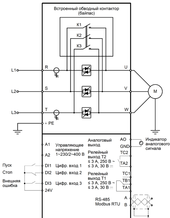
Рисунок 26 – Схема подключения клемм устройства плавного пуска серии SBIM мощностью от 18.5 кВт
