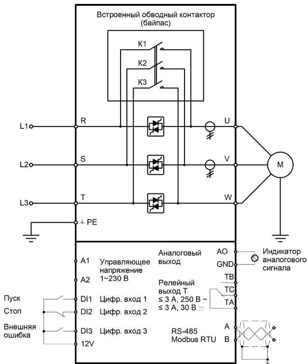
Рисунок 2а – Схема подключения клемм устройства плавного пуска серии SBIM мощностью до 15 кВт
