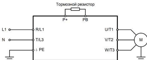
Рисунок 2б – Подключение силовых клемм для моделей LCI-GY/PY-2(B)
