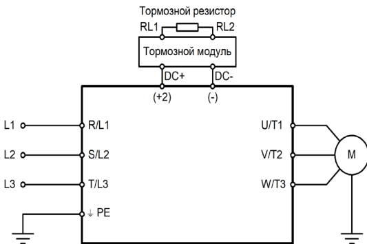
Рисунок 2б – Подключение силовых клемм для моделей LCI-GY/PY-6
