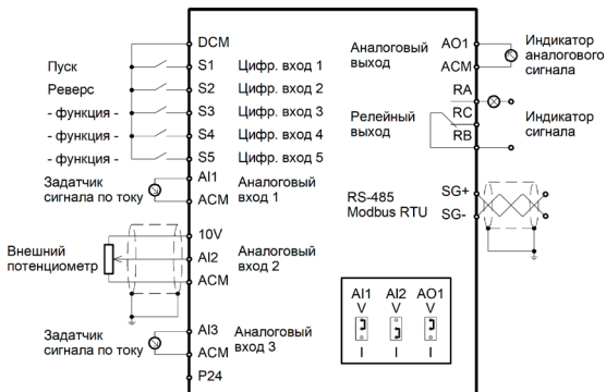
Рисунок 3 – Подключение управляющих клемм для преобразователя частоты серии LCI(S) и LCI-GY/PY-1
