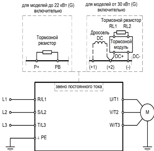
Рисунок 2а – Подключение силовых клемм для моделей LCI-GY/PY-4(B)
