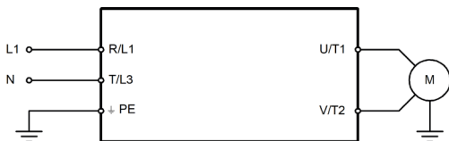
Рисунок 2а – Подключение силовых клемм для моделей LCI-GY/PY-1
