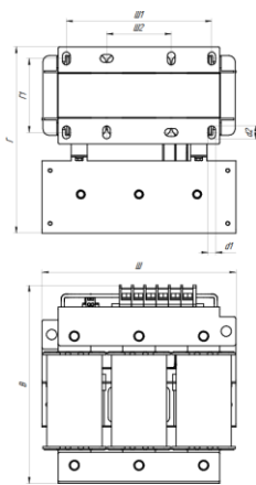
Рисунок 9 - Типоисполнение Б серии ISINOF-6
