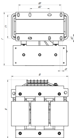
Рисунок 10 - Типоисполнение В серии ISINOF-6
