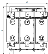
Рисунок 16 - Типоисполнение К серии ISINOF-6
