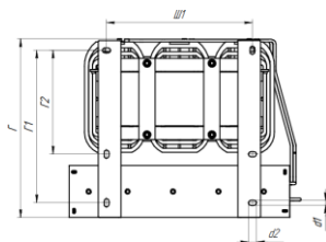
Рисунок 15 - Типоисполнение И серии ISINOF-6
