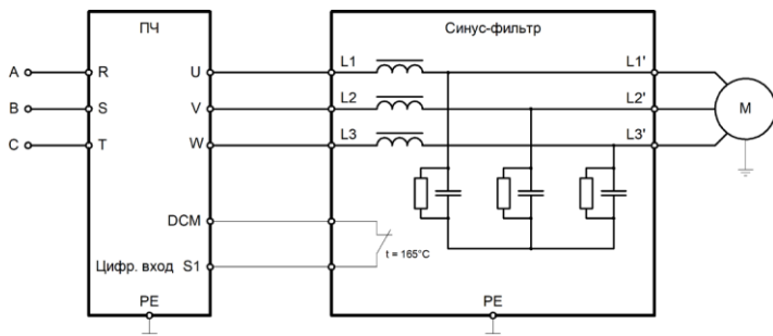
Рисунок 20 — Схема подключения на примере преобразователя частоты серии LCI и синусного фильтра серии ISINOF-4 мощностью до 18,5 кВт (включительно)
