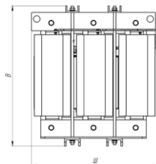
Рисунок 6 – Типоисполнение Е серии ISINOF-4
