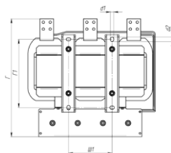
Рисунок 5 – Типоисполнение Д серии ISINOF-4
