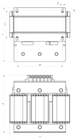
Рисунок 2 – Типоразмер Б серии ISINOF-4
