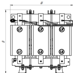
Рисунок 15 - Типоисполнение И серии ISINOF-6
