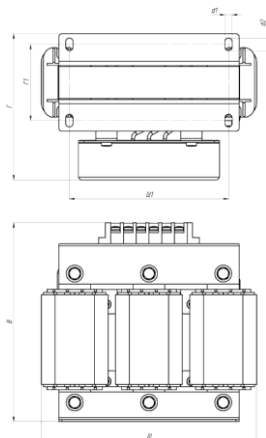
Рисунок 1 – Типоразмер А серии ISINOF-4
