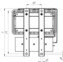
Рисунок 11 - Типоисполнение Г серии ISINOF-6
