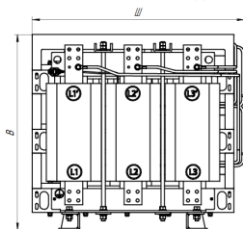
Рисунок 17 - Типоисполнение Л серии ISINOF-6
