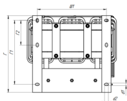
Рисунок 14 - Типоисполнение Ж серии ISINOF-6
