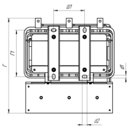
Рисунок 10 - Типоисполнение В серии ISINOF-6
