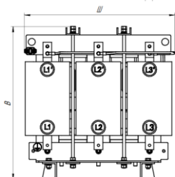
Рисунок 14 - Типоисполнение Ж серии ISINOF-6
