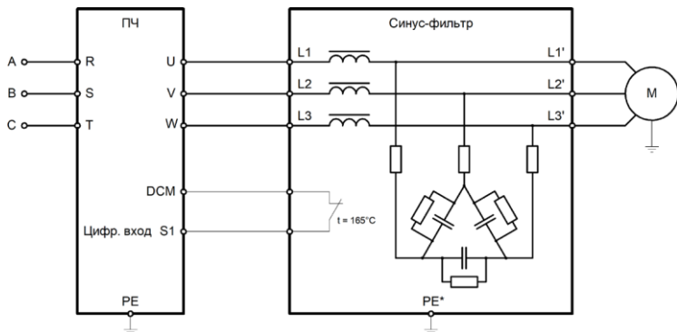
Рисунок 21 — Схема подключения на примере преобразователя частоты серии LCI и синусного фильтра серии ISINOF-4 мощностью от 22 кВт (включительно)
