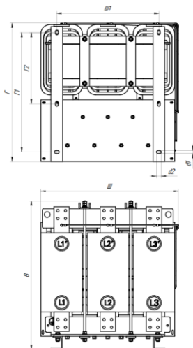
Рисунок 19 - Типоисполнение Н серии ISINOF-6
