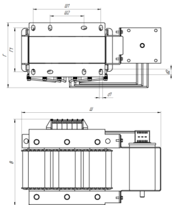
Рисунок 3 – Типоразмер В серии ISINOF-4
