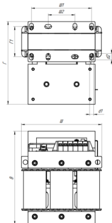
Рисунок 8 - Типоисполнение А серии ISINOF-6
