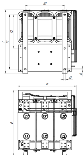
Рисунок 18 - Типоисполнение М серии ISINOF-6
