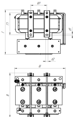
Рисунок 11 - Типоисполнение Г серии ISINOF-6
