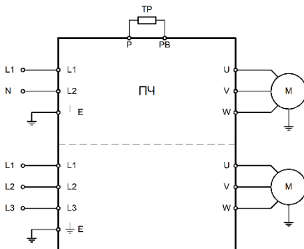
Рис. 3.2 - Схема силовых подключений
