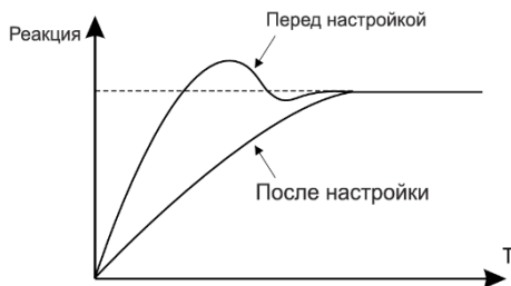
Рис. 6.19 - Управление перерегулированием
