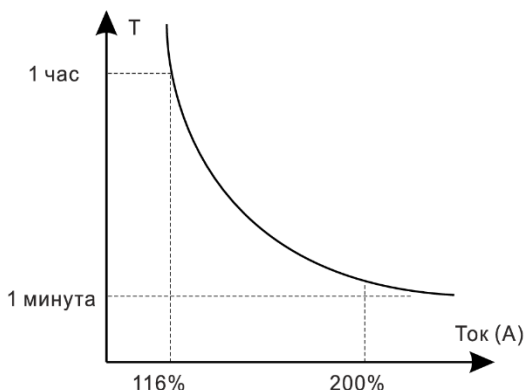
Рис. 6.5 - Кривая зависимости тока перегрузки от времени
