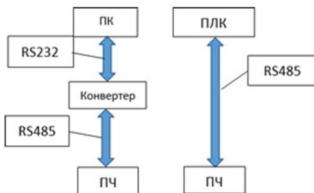
Рус. 7.1 - Сетевой режим Master/Slave
