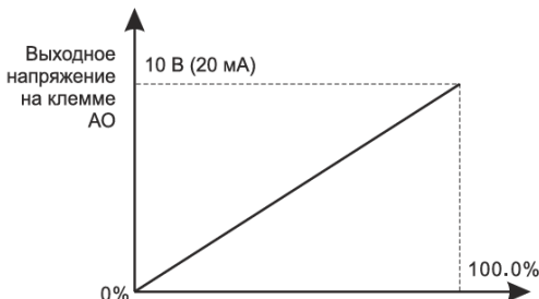
Рис. 6.12 - Выходное напряжение на клемме АО
