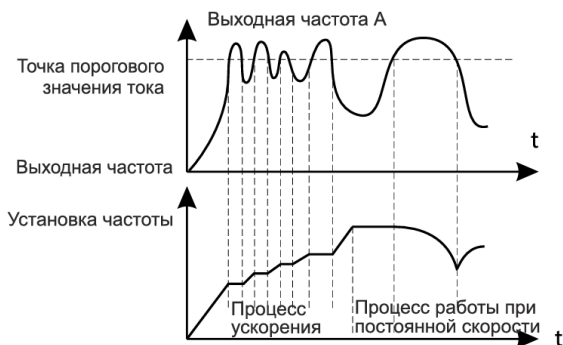
Группа параметров SdB.05 – SdB.07
