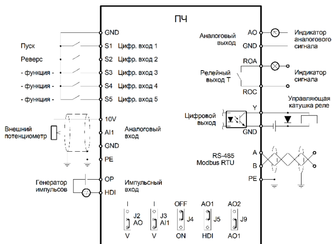
Рис. 3.4 – Схема подключения управляющих клемм
