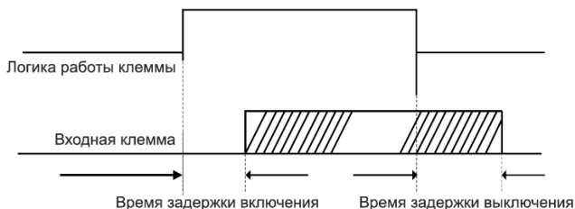
Рис. 6.11 - Время задержки включения и выключения клемм
