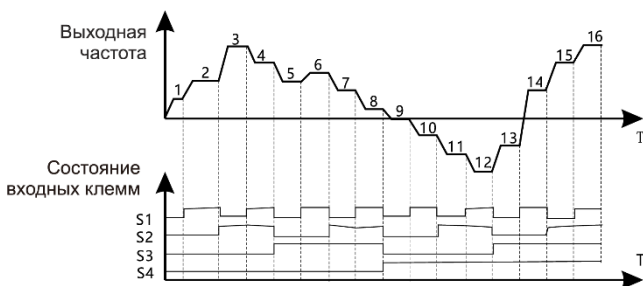
Рис. 6.24 - Многоступенчатое управление
