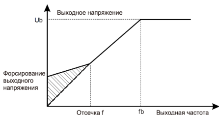
Рис. 6.7 - Повышение крутящего момента электродвигателя
