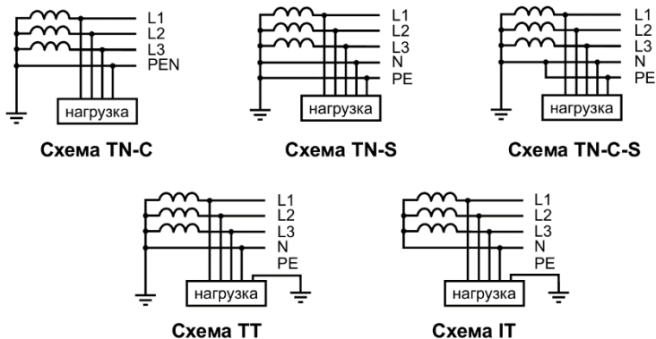
Рис. 3.6 - Типы систем заземления
