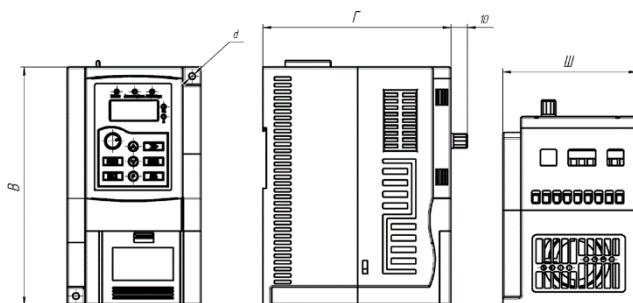
Рис. 2.5 Массогабаритные характеристики ПЧ серии SDI
