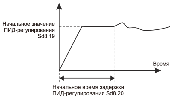
Рис. 6.17 - Принцип работы начального значения ПИД-регулирования
