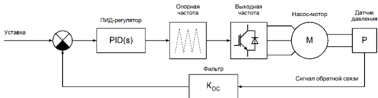
Рис. 6.15 - Схема ПИД-регулирования
