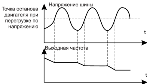
Рис. 6.25 - Защита при превышении напряжения
