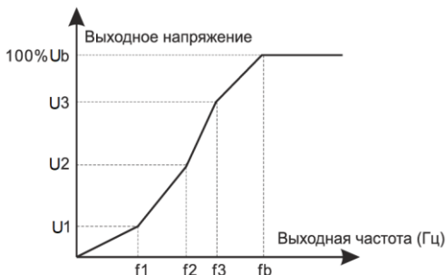
Рис. 6.8 - Ломаная характеристика U/f
