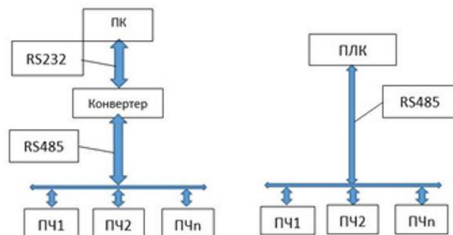
Рус. 7.2 - Сетевой режим Master/Slaves
