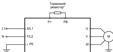
Рисунок 3.2 – Схема силовых подключений для моделей INVENT-GY-2
