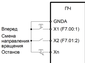
Рисунок 6.15 – Схема трехпроводного подключения 2
