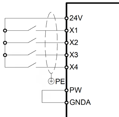
Рисунок 3.16 – Схема подключения, при которой внешний источник питания не используется, цифровые входы в режиме PNP
