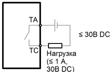
Рисунок 3.13 – Схема подключения нагрузки постоянного тока к релейному выходу
