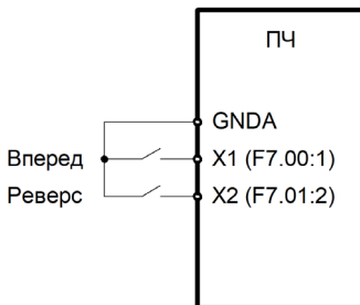
Рисунок 6.12 – Схема двухпроводного подключения 1
