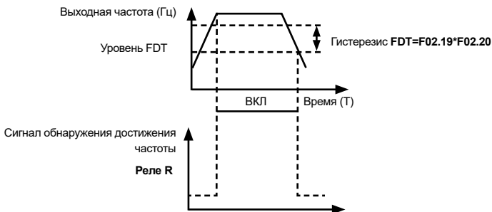
Рисунок 6.7 – Значение обнаружения выходной частоты
