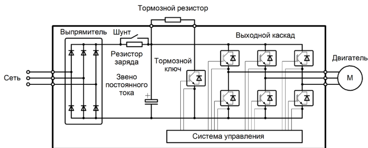
Рисунок 2.1 – Принципиальная электрическая схема устройства трехфазных моделей INVENT со встроенным тормозным модулем
