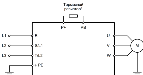
Рисунок 3.3 – Схема силовых подключений для моделей INVENT-GY-2
