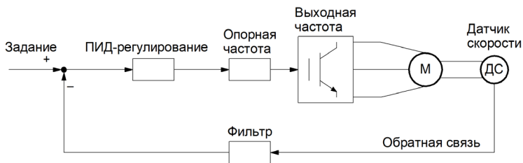
Рисунок 6.16 – Схема ПИД-регулирования
