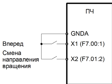
Рисунок 6.13 – Схема двухпроводного подключения 2
