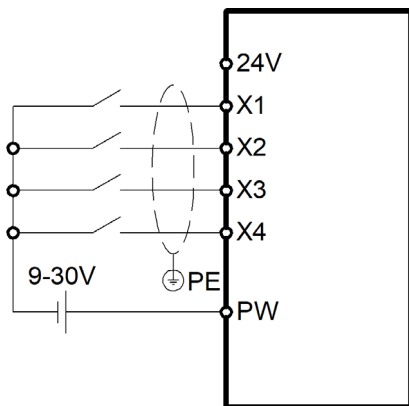
Рисунок 3.15 – Схема подключения, при которой используется внешний источник питания, цифровые входы в режиме NPN
