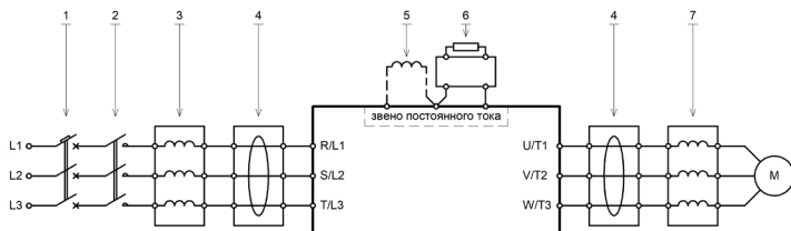
Рисунок 3.4 – Схема подключения дополнительного оборудования
