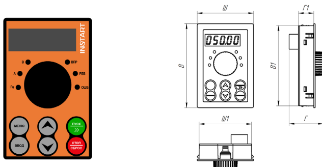
Рисунок 5.2 – Выносная панель управления INVENT-KP
