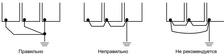
Рисунок 3.7 – Схематичное изображение образования петли с заземляющим проводом
