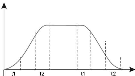
Рисунок 6.3 – S-образная кривая ускорения и замедления
