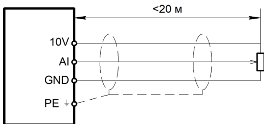
Рисунок 3.10 – Схема подключения проводов к аналоговому входу (общий случай)
