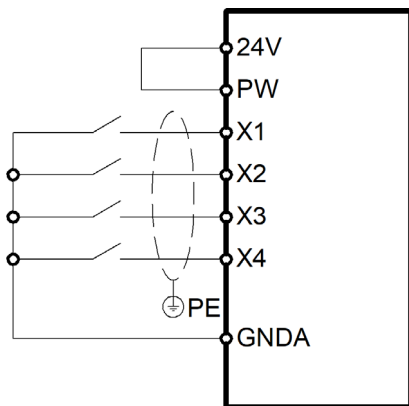
Рисунок 3.14 – Схема подключения, при которой внешний источник питания не используется, цифровые входы в режиме NPN (по умолчанию)
