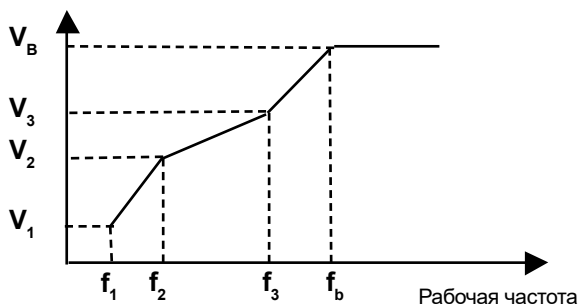
Рисунок 6.11 – Ломаная характеристика V/f
