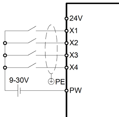
Рисунок 3.17 – Схема подключения, при которой используется внешний источник питания, цифровые входы в режиме PNP
