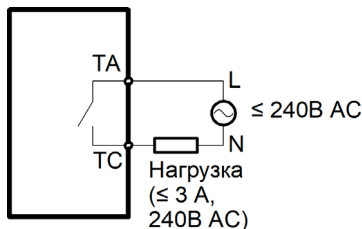
Рисунок 3.12 – Схема подключения нагрузки переменного тока к релейному выходу
