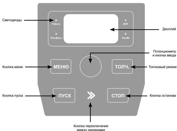
Рисунок 5.1 – Функции кнопок и светодиодов панели управления INVENT
