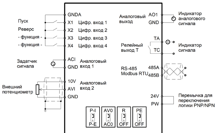
Рисунок 3.6 – Схема подключения управляющих клемм серии INVENT
