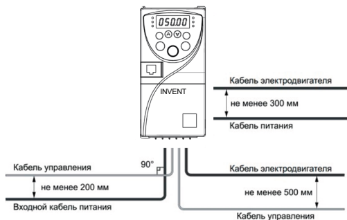
Рисунок 3.8 – Графическое представление расстояний между кабелями
