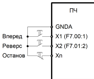
Рисунок 6.14 – Схема трехпроводного подключения 1
