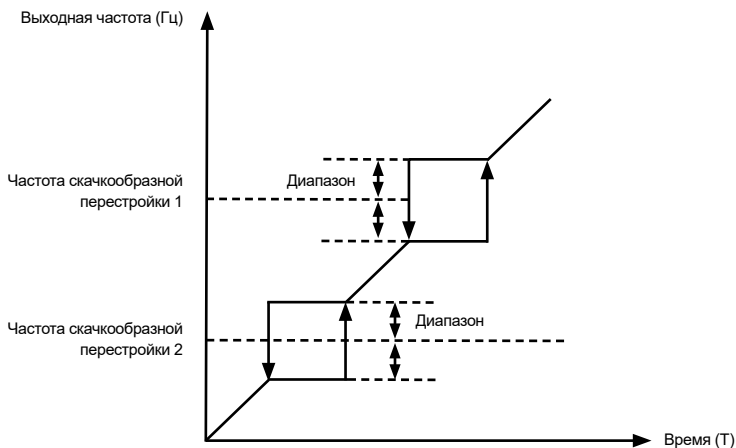
Рисунок 6.5 – Принцип работы функции скачкообразной перестройки
