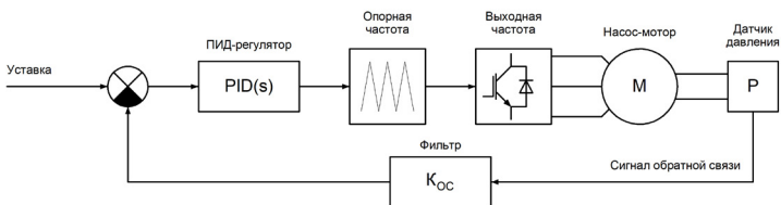
Рис. 6.15 - Схема ПИД-регулирования
