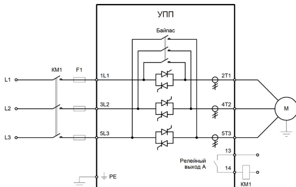
Схема подключения двигателя «в линию»
