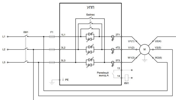
Схема подключения двигателя «внутри треугольника»
