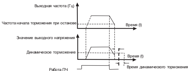
Рисунок 6.5 – Процесс торможения постоянным током
