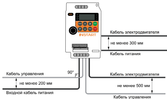
Рис. 3.7 Графическое представление расстояний между кабелями
