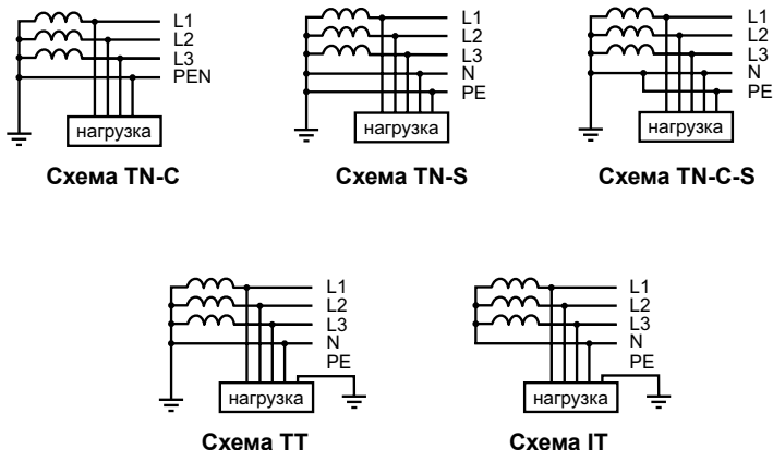
Рис. 3.6 – Типы систем заземления
