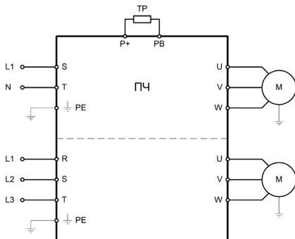
Рис 3.2 Схема силовых подключений
