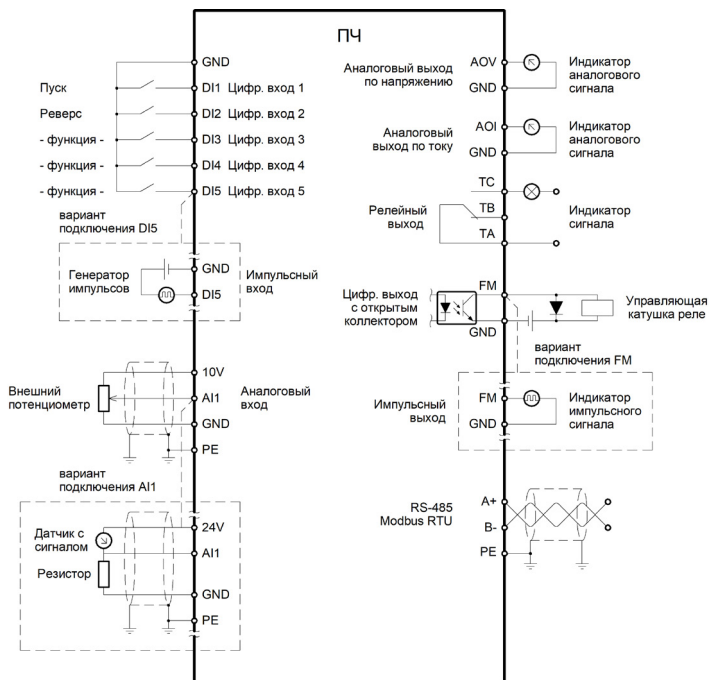
Рис. 3.4 – Схема подключения управляющих клемм
