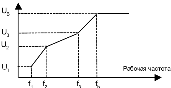
Рисунок 6.7 – Ломаная характеристика U/f
