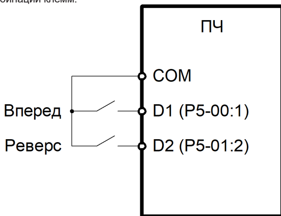
Рисунок 6.9 – Схема двухпроводного подключения 1
