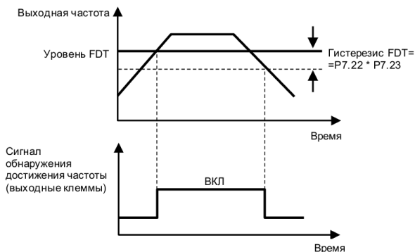
Рисунок 6.16 – Значение обнаружения выходной частоты
