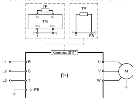
Рисунок 3.5 – Схема силовых подключений для моделей NCI-GY/PY-4B от 37 кВт
