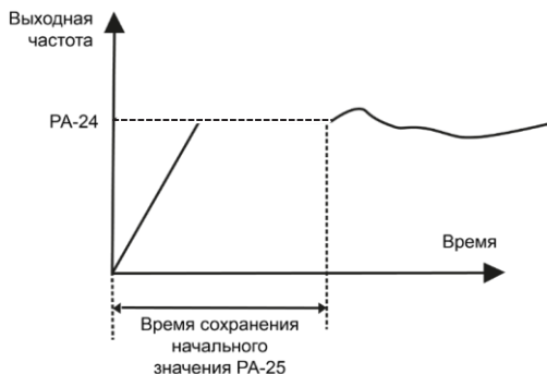
Рисунок 6.22 – Время сохранения опорного значения
