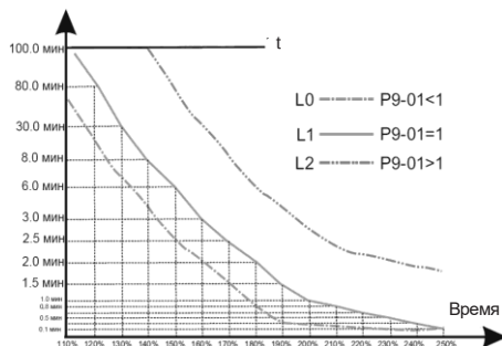
Рисунок 6.18 – Обратнозависимая времятоковая характеристика
