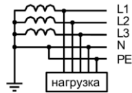
Схема TN-C-S
