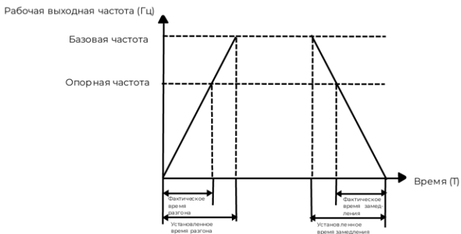
Рисунок 6.3 – Время разгона/замедления
