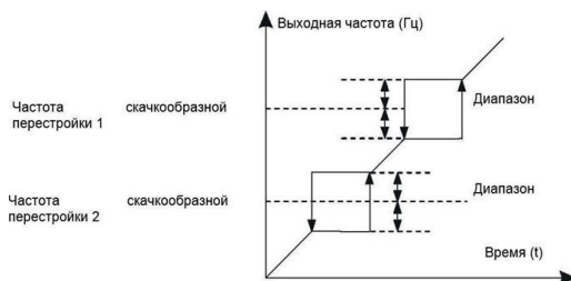
Рисунок 6.14 – Принцип работы функции скачкообразной перестройки
