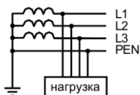
Схема TN-C
