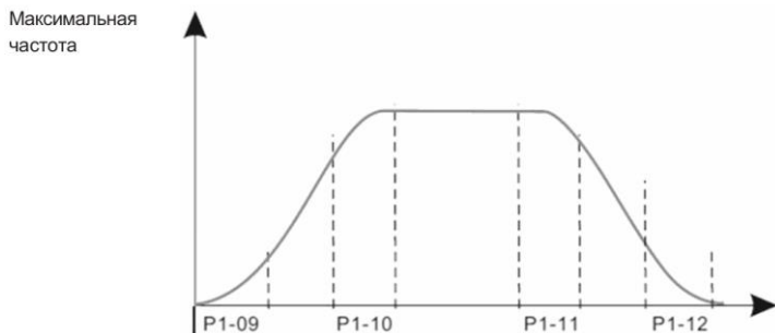
Рисунок 6.4 – S-образная кривая ускорения и замедления
