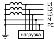
Схема TN-S
