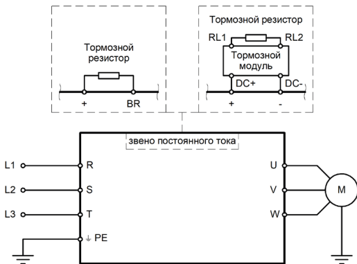
Рисунок 5 – Схема силовых подключений для моделей INPRIME MX-GY/PY-4(B/F)
