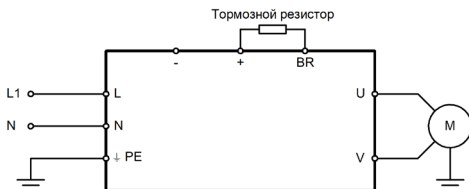
Рисунок 2 – Схема силовых подключений для моделей INPRIME MX-GY/PY-1B
