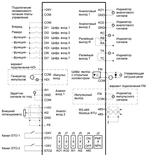
Рисунок 6 – Подключение клемм управления
