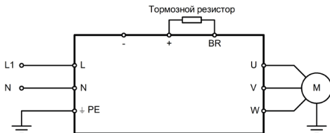
Рисунок 3 – Схема силовых подключений для моделей INPRIME MX-GY/PY-2B
