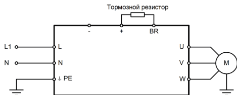
Рисунок 4 – Схема силовых подключений для моделей INPRIME MX-GY/PY-3B
