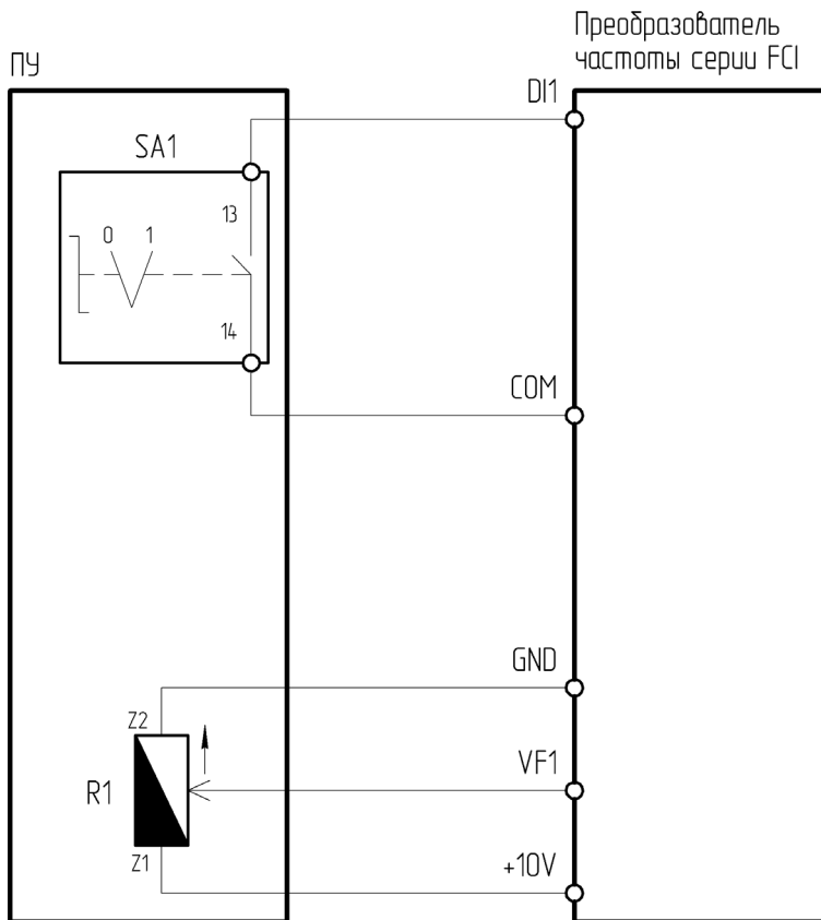
Рисунок 4.1.6– Схема подключения ПУ-2-011 к преобразователю частоты серии FCI
