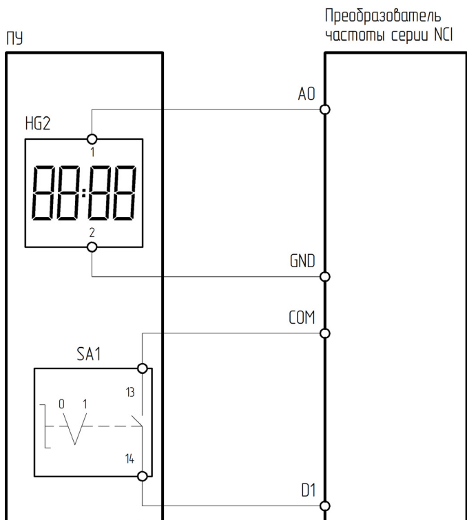
Рисунок 4.14.6 – Схема подключения ПУ-2-610 к преобразователю частоты серии NCI
