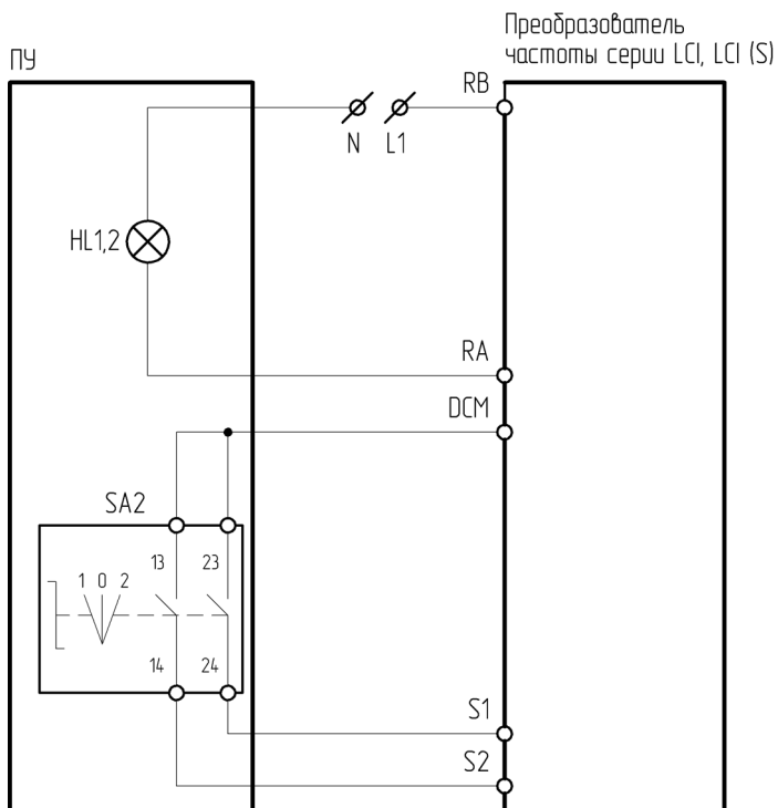
Рисунок 4.11.4 – Схема подключения ПУ-2-220, ПУ-2-520 к преобразователю частоты серии LCI/LCI(S)
