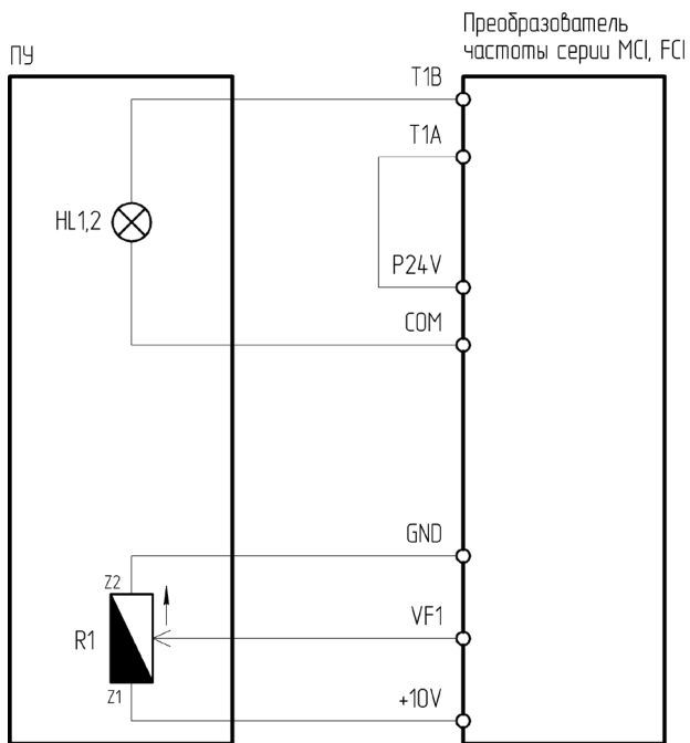
Рисунок 4.5.4 – Схема подключения ПУ-2-101, ПУ-2-401 к преобразователю частоты серии MCI/FCI
