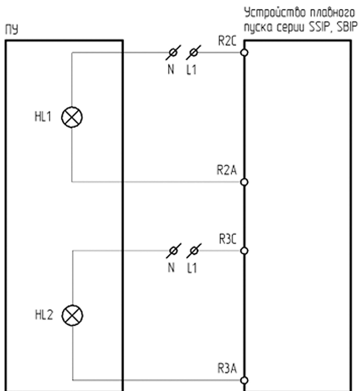
Рисунок 4.18.3 – Схема подключения ПУ-2-800 к устройству плавного пуска серии SSIP/SBIP
