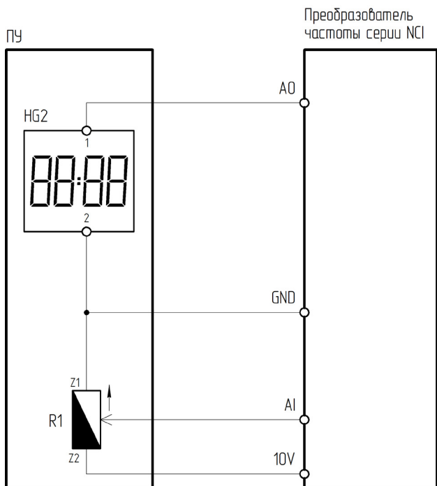
Рисунок 4.13.3 – Схема подключения ПУ-2-601 к преобразователю частоты серии NCI
