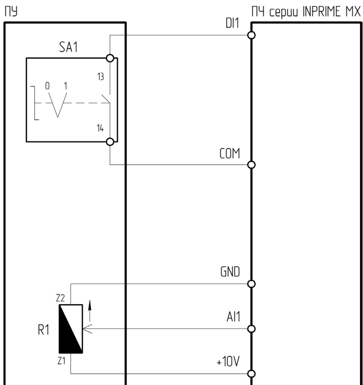
Рисунок 4.1.8 – Схема подключения ПУ-2-011 к преобразователю частоты серии INPRIME MX
