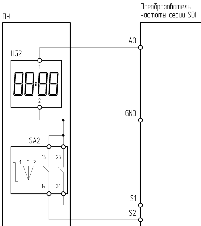
Рисунок 4.15.2 – Схема подключения ПУ-2-620 к преобразователю частоты серии SDI
