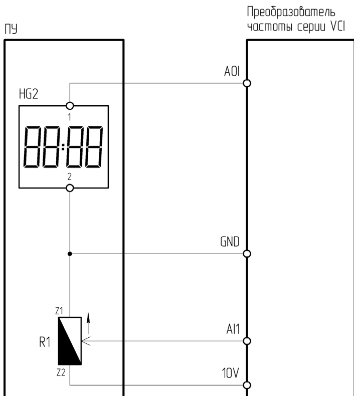
Рисунок 4.13.1 – Схема подключения ПУ-2-601 к преобразователю частоты серии VCI
