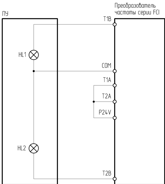
Рисунок 4.17.4 – Схема подключения ПУ-2-700 к преобразователю частоты серии FCI
