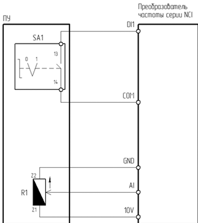
Рисунок 4.2.3 – Схема подключения ПУ-2-021 к преобразователю частоты серии NCI
