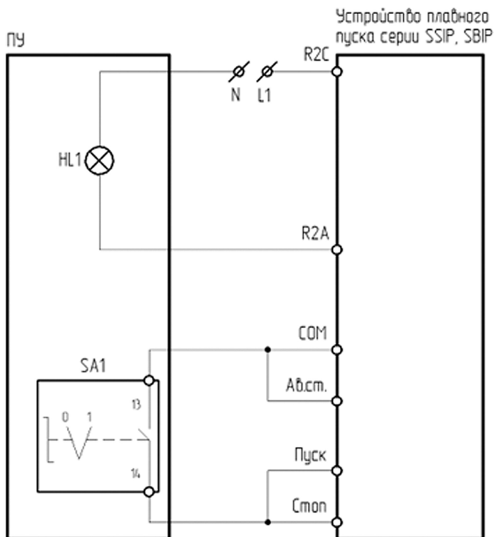
Рисунок 4.10.3а – Схема подключения ПУ-2-210, к устройству плавного пуска серии SSIP/SBIP
