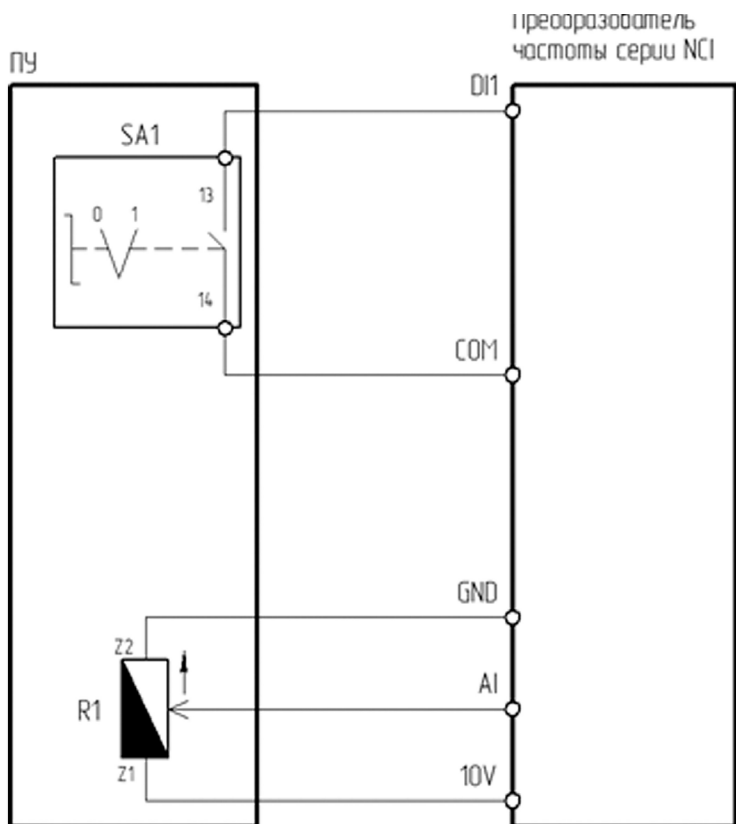
Рисунок 4.1.3 – Схема подключения ПУ-2-011 к преобразователю частоты серии NCI
