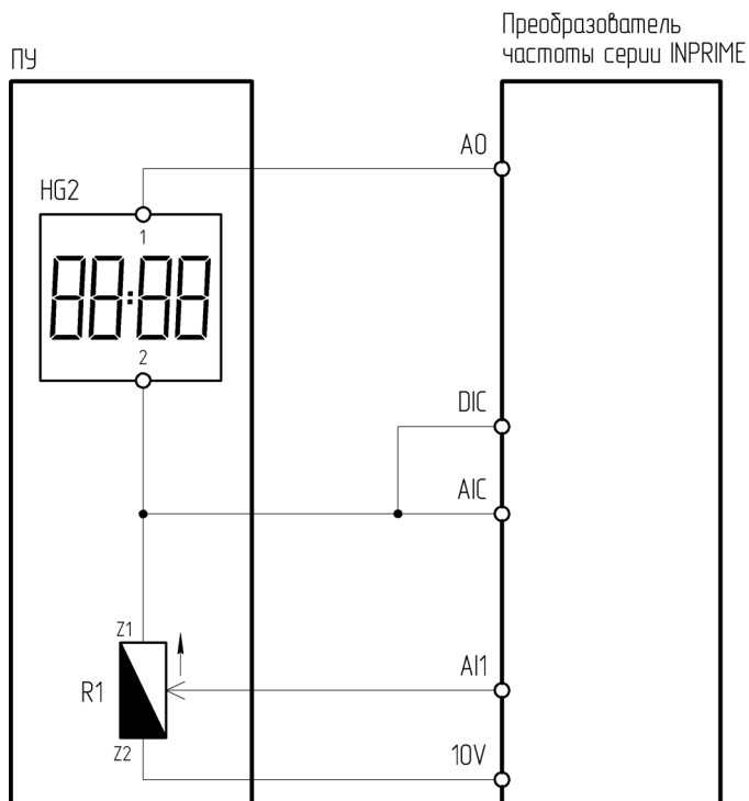
Рисунок 4.13.6 – Схема подключения ПУ-2-601 к преобразователю частоты серии INPRIME
