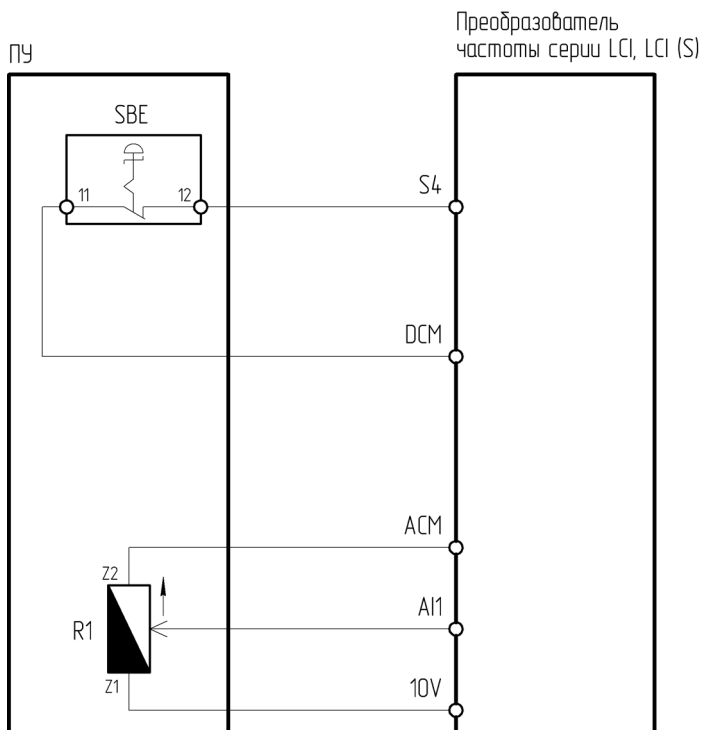
Рисунок 4.4.4 – Схема подключения ПУ-2-071 к преобразователю частоты серии LCI/LCI(S)
