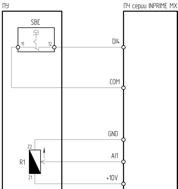
Рисунок 4.4.8 – Схема подключения ПУ-2-071 к преобразователю частоты серии INPRIME MX
