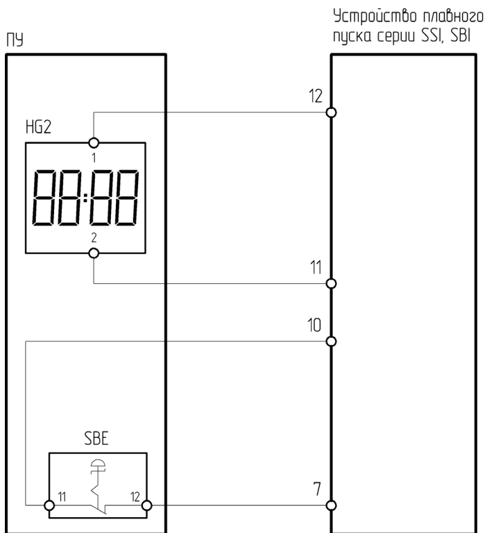
Рисунок 4.16.1 – Схема подключения ПУ-2-670 к устройству плавного пуска серии SSI/SBI
