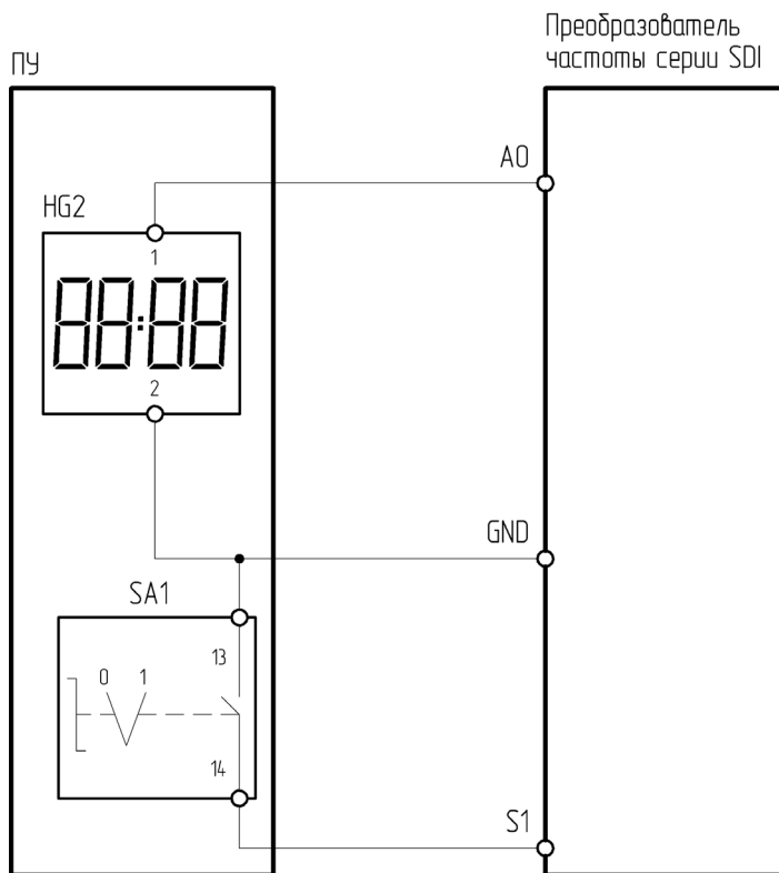
Рисунок 4.14.5 – Схема подключения ПУ-2-610 к преобразователю частоты серии SDI
