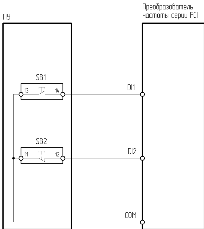
Рисунок 4.3.10 – Схема подключения ПУ-2-030 к преобразователю частоты серии FCI
