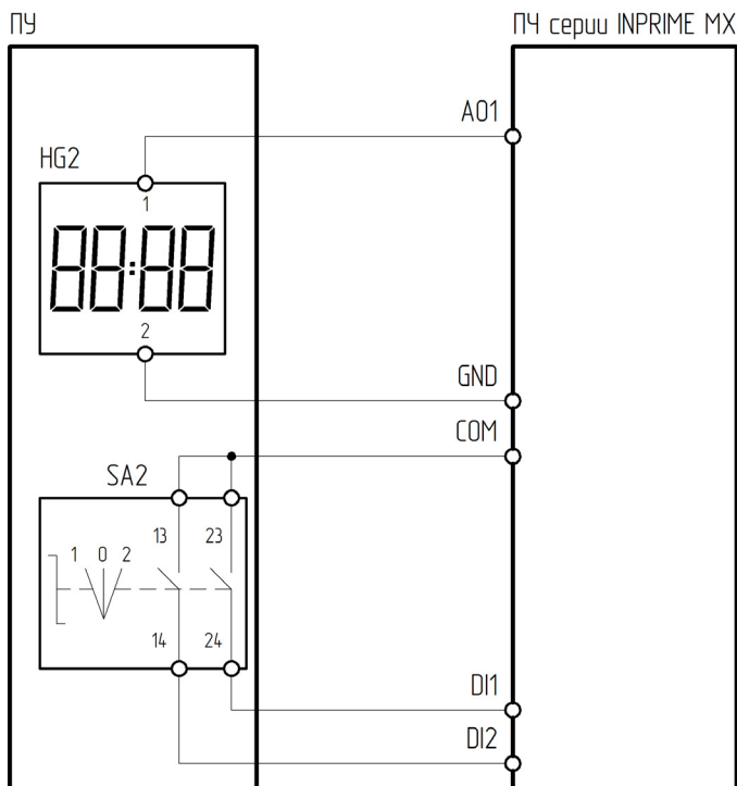
Рисунок 4.15.10 – Схема подключения ПУ-2-620 к преобразователю частоты серии INPRIME MX
