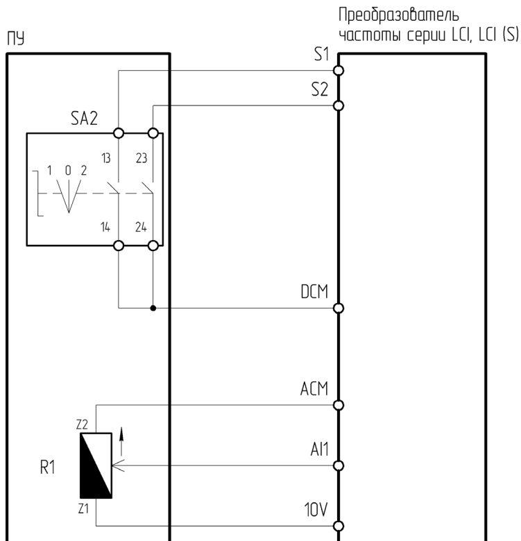
Рисунок 4.2.4 – Схема подключения ПУ-2-021 к преобразователю частоты серии LCI/LCI(S)
