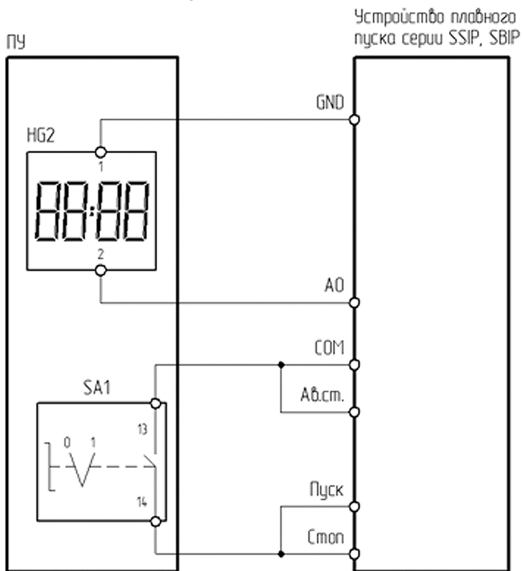
Рисунок 4.14.2 – Схема подключения ПУ-2-610 к устройству плавного пуска серии SSIP/SBIP
