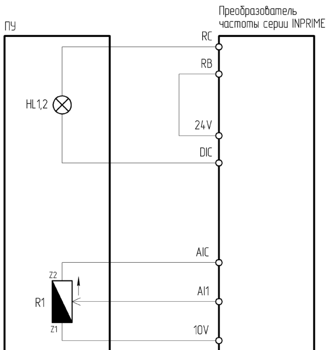
Рисунок 4.5.5 – Схема подключения ПУ-2-101, ПУ-2-401 к преобразователю частоты серии INPRIME
