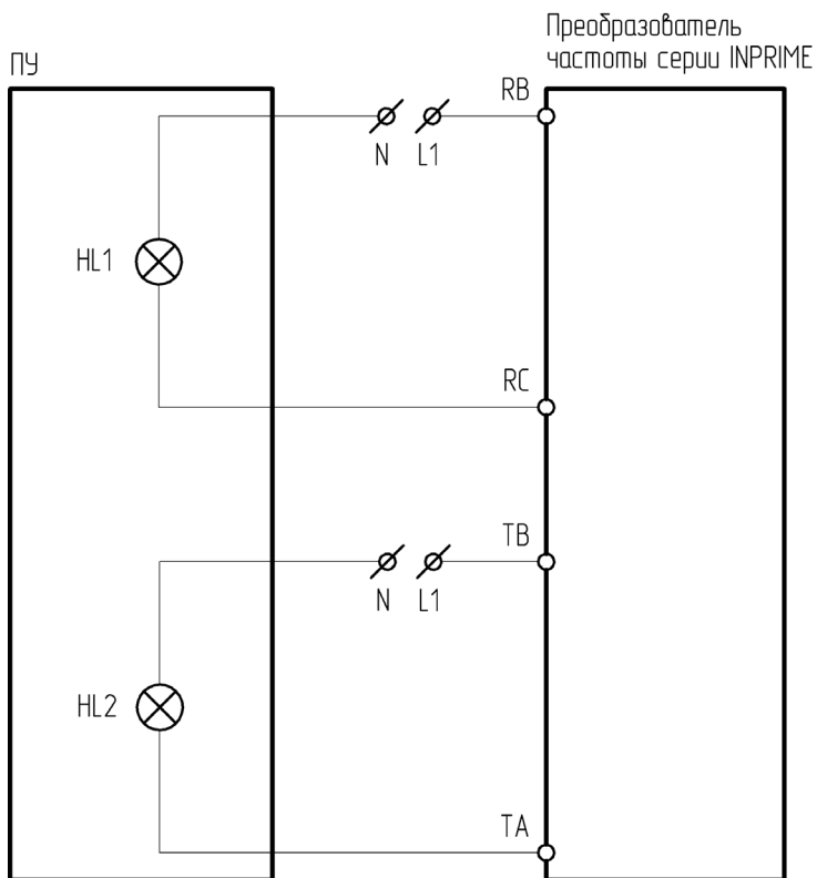
Рисунок 4.18.7 – Схема подключения ПУ-2-800 к преобразователю частоты серии INPRIME
