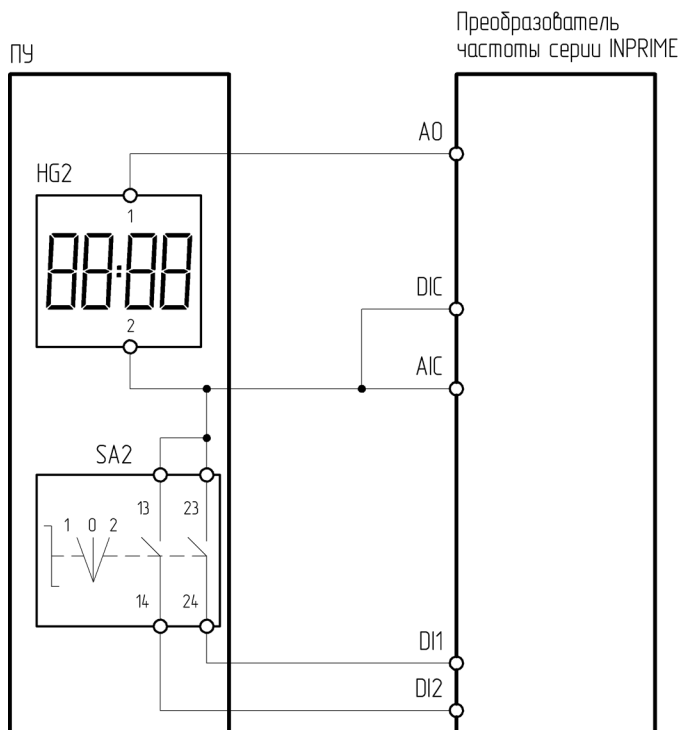
Рисунок 4.15.7 – Схема подключения ПУ-2-620 к преобразователю частоты серии INPRIME
