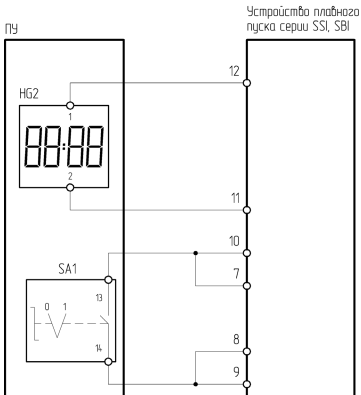
Рисунок 4.14.1 – Схема подключения ПУ-2-610 к устройству плавного пуска серии SSI/SBI
