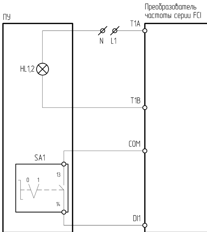
Рисунок 4.10.10 – Схема подключения ПУ-2-210, ПУ-2-510 к преобразователю частоты серии FCI
