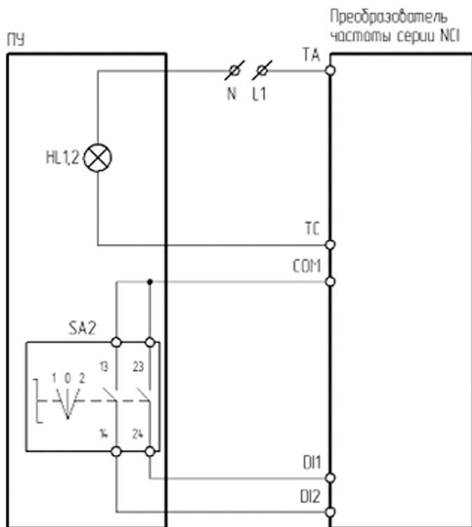
Рисунок 4.11.3 – Схема подключения ПУ-2-220, ПУ-2-520 к преобразователю частоты серии NCI
