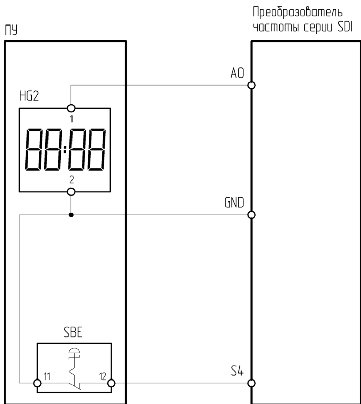
Рисунок 4.16.5 – Схема подключения ПУ-2-670 к преобразователю частоты серии SDI
