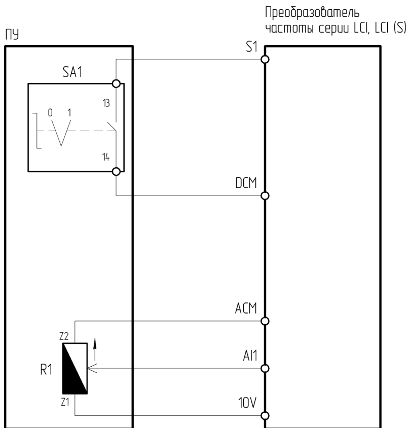
Рисунок 4.1.4 – Схема подключения ПУ-2-011 к преобразователю частоты серии LCI/LCI(S)
