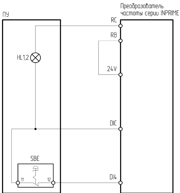
Рисунок 4.8.7 – Схема подключения ПУ-2-170, ПУ-2-470 к преобразователю частоты серии INPRIME
