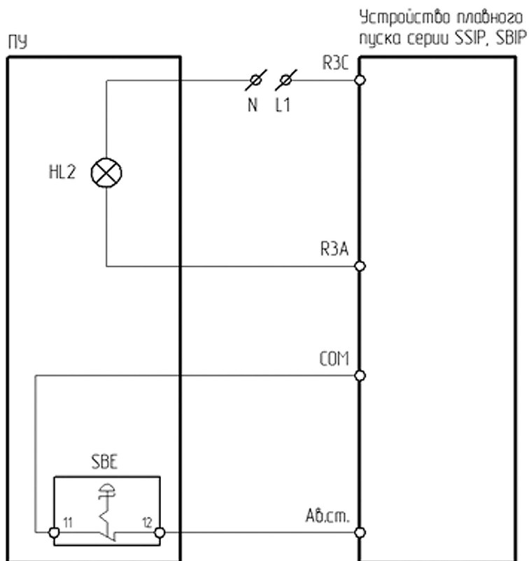
Рисунок 4.12.26 – Схема подключения ПУ-2-570 к устройству плавного пуска серии SSIP/SBIP
