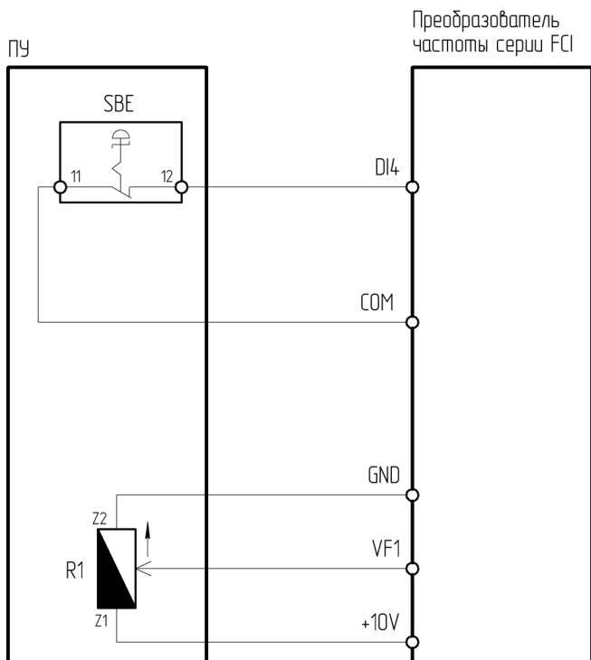
Рисунок 4.4.6 – Схема подключения ПУ-2-071 к преобразователю частоты серии FCI
