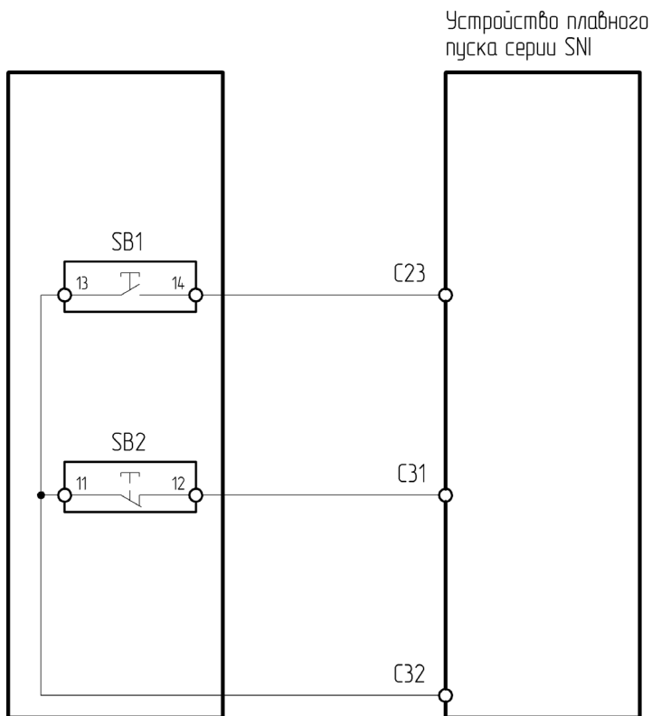
Рисунок 4.3.4 Схема подключения ПУ-2-030 к устройству плавного пуска серии SNI
