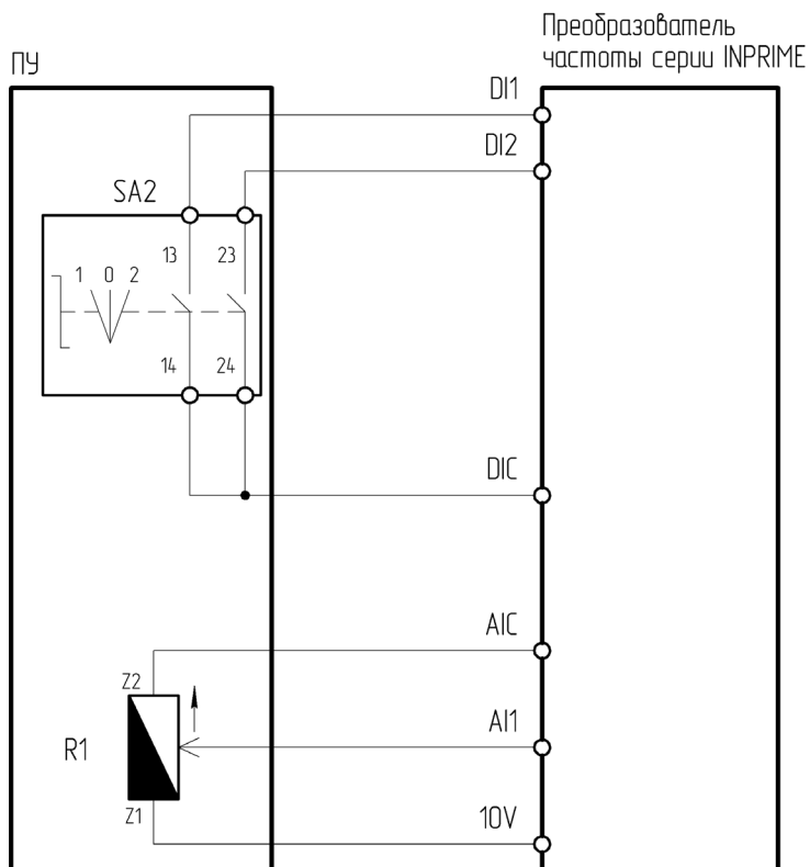
Рисунок 4.2.7 – Схема подключения ПУ-2-021 к преобразователю частоты серии INPRIME
