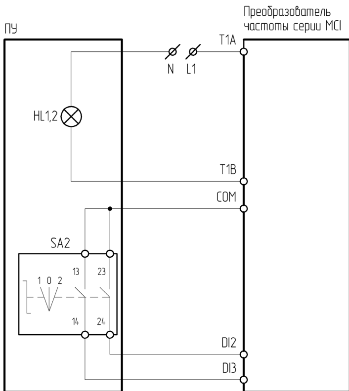
Рисунок 4.11.5 – Схема подключения ПУ-2-220, ПУ-2-520 к преобразователю частоты серии MCI
