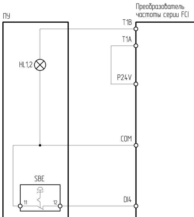
Рисунок 4.8.6 – Схема подключения ПУ-2-170, ПУ-2-470 к преобразователю частоты серии FCI
