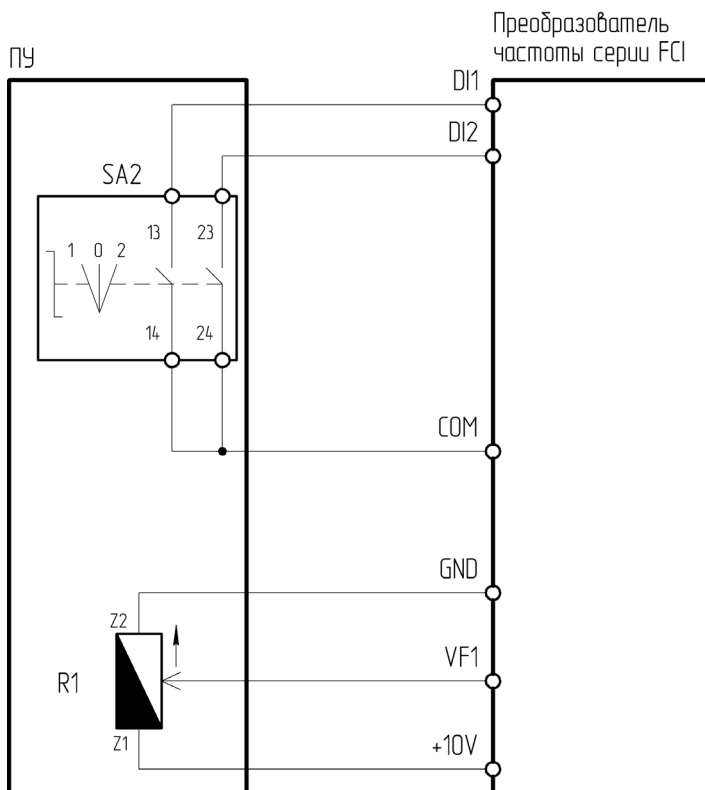
Рисунок 4.2.6 – Схема подключения ПУ-2-021 к преобразователю частоты серии FCI
