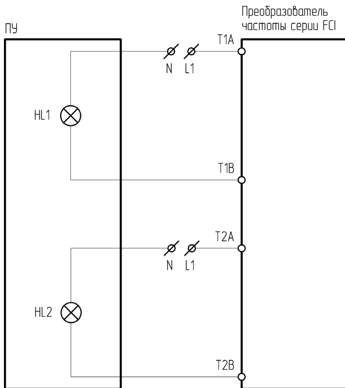
Рисунок 4.18.6 – Схема подключения ПУ-2-800 к преобразователю частоты серии FCI
