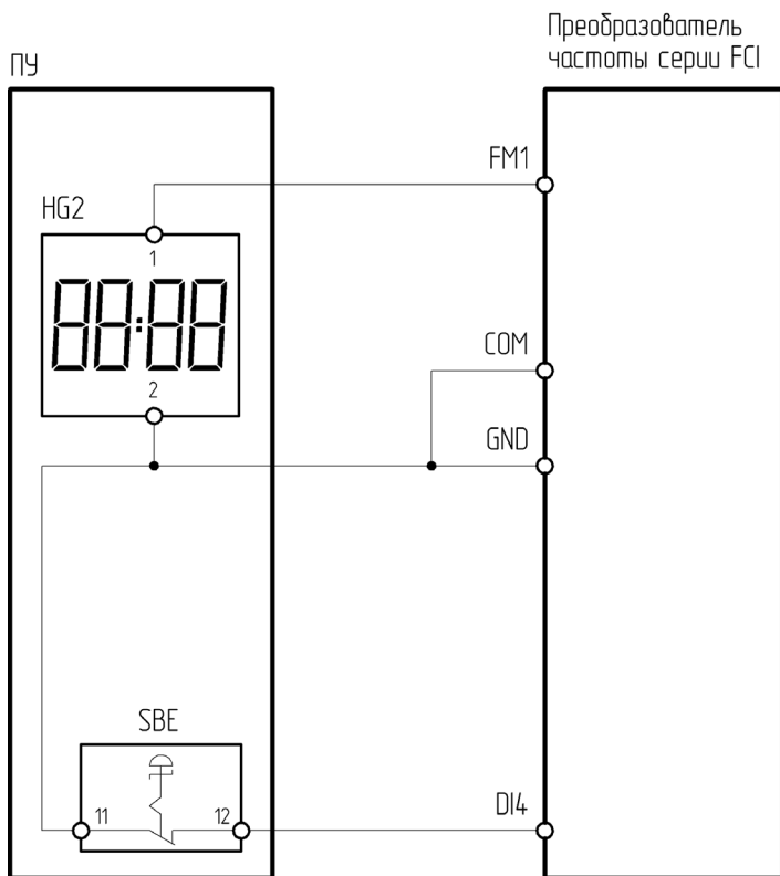
Рисунок 4.16.9 – Схема подключения ПУ-2-670 к преобразователю частоты серии FCI
