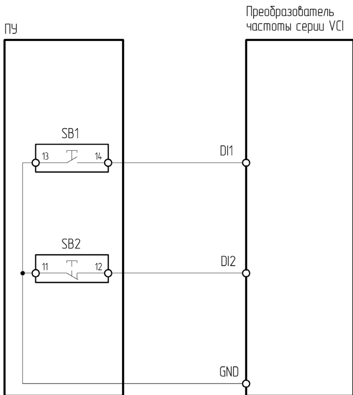
Рисунок 4.3.5 – Схема подключения ПУ-2-030 к преобразователю частоты серии VCI
