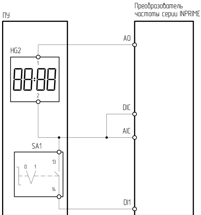
Рисунок 4.14.10 – Схема подключения ПУ-2-610 к преобразователю частоты серии INPRIME
