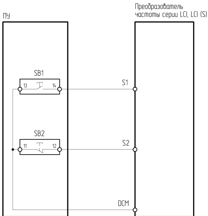
Рисунок 4.3.8 – Схема подключения ПУ-2-030 к преобразователю частоты серии LCI/LCI(S)
