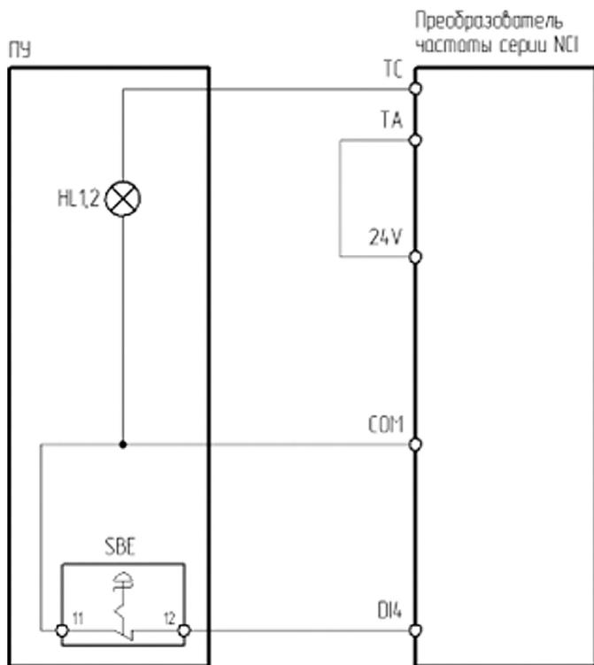
Рисунок 4.8.3 – Схема подключения ПУ-2-170, ПУ-2-470 к преобразователю частоты серии NCI
