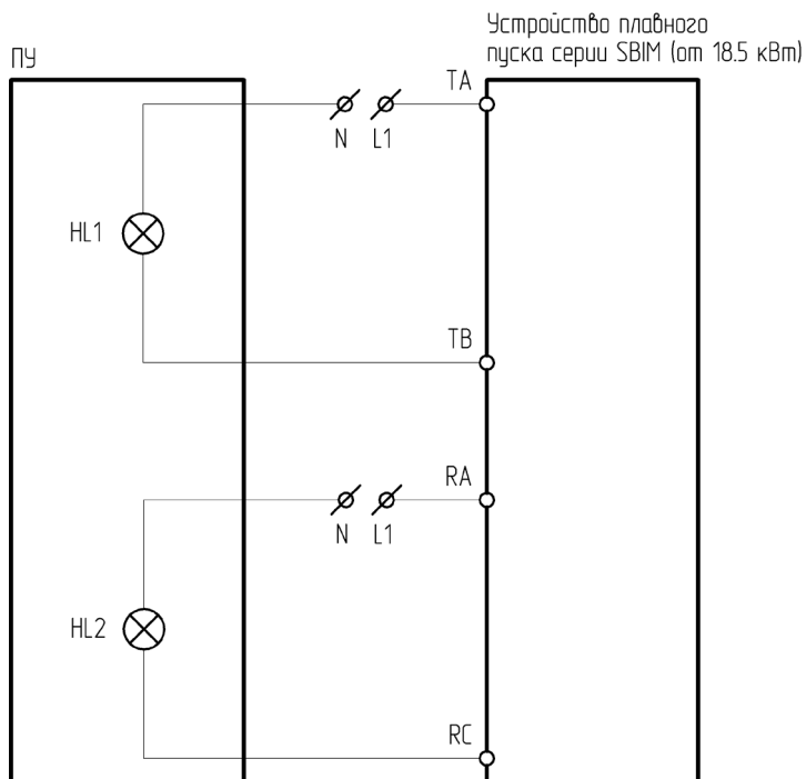
Рисунок 4.18.1 – Схема подключения ПУ-2-800 к устройству плавного пуска серии SBIM
