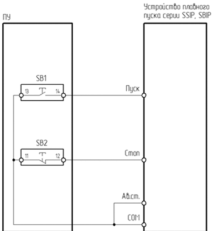
Рисунок 4.3.3 – Схема подключения ПУ-2-030 к устройству плавного пуска серии SSIP/SBIP
