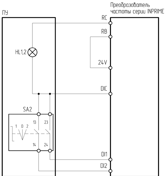
Рисунок 4.7.6 – Схема подключения ПУ-2-120, ПУ-2-420 к преобразователю частоты серии INPRIME
