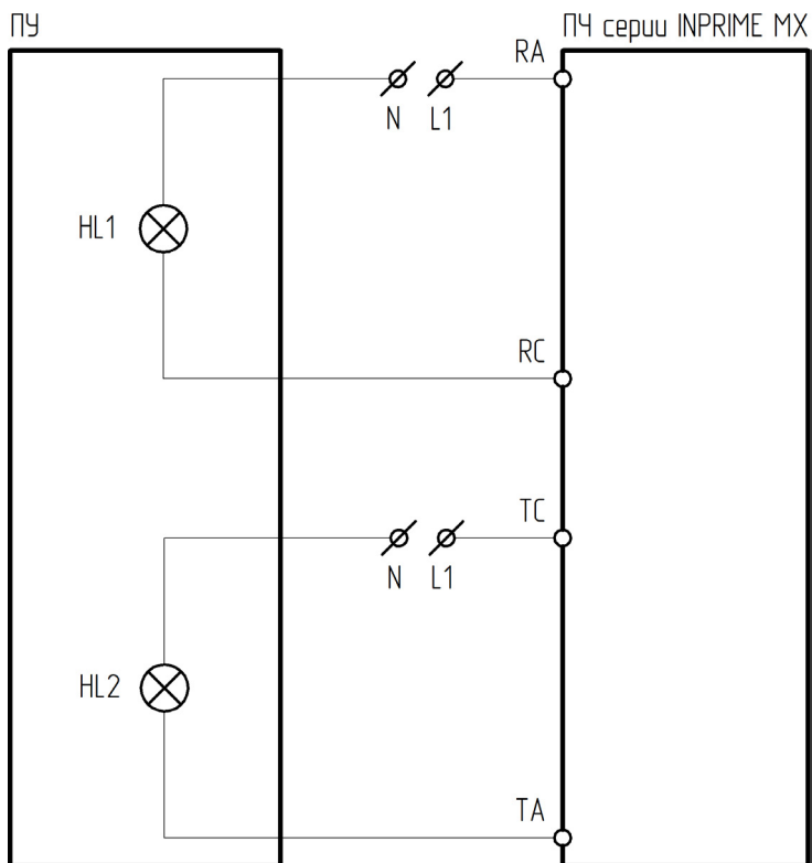
Рисунок 4.18.8 – Схема подключения ПУ-2-800 к преобразователю частоты серии INPRIME MX
