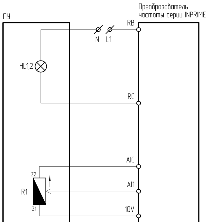
Рисунок 4.9.6 – Схема подключения ПУ-2-201, ПУ-2-501 к преобразователю частоты серии INPRIME
