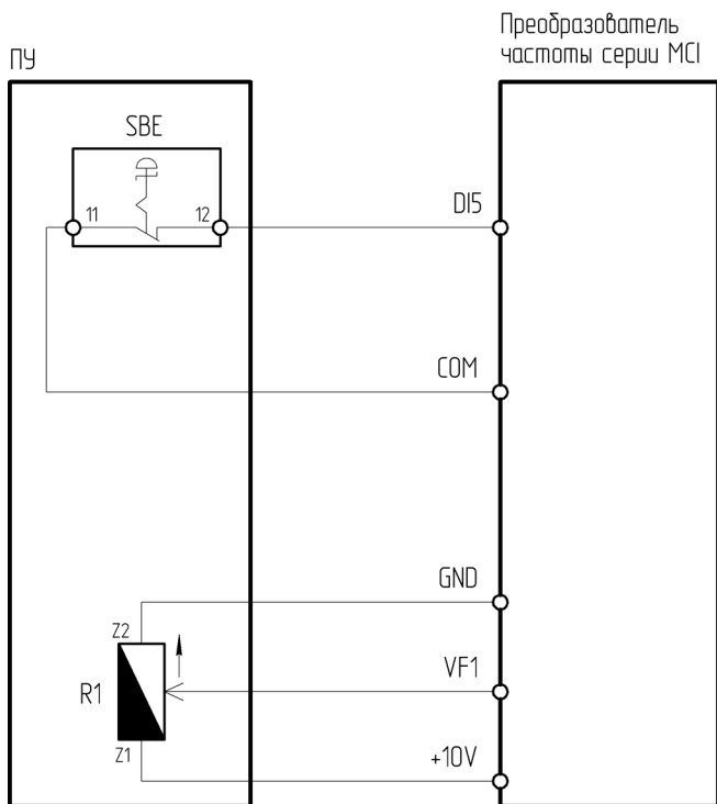
Рисунок 4.4.5 – Схема подключения ПУ-2-071 к преобразователю частоты серии МСІ
