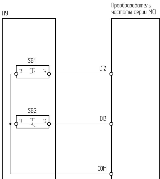
Рисунок 4.3.9 – Схема подключения ПУ-2-030 к преобразователю частоты серии MCI
