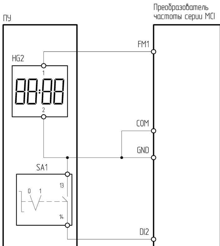
Рисунок 4.14.8 – Схема подключения ПУ-2-610 к преобразователю частоты серии МС1
