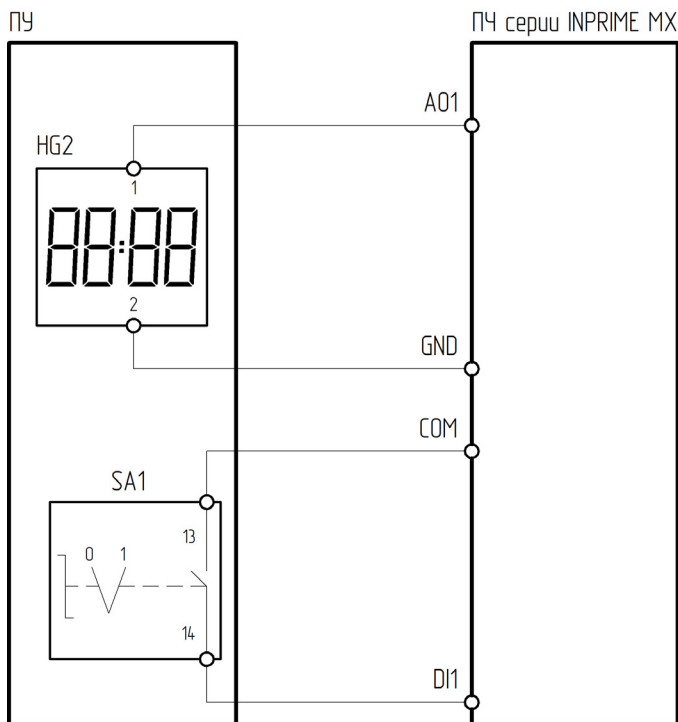
Рисунок 4.14.11 – Схема подключения ПУ-2-610 к преобразователю частоты серии INPRIME MX
