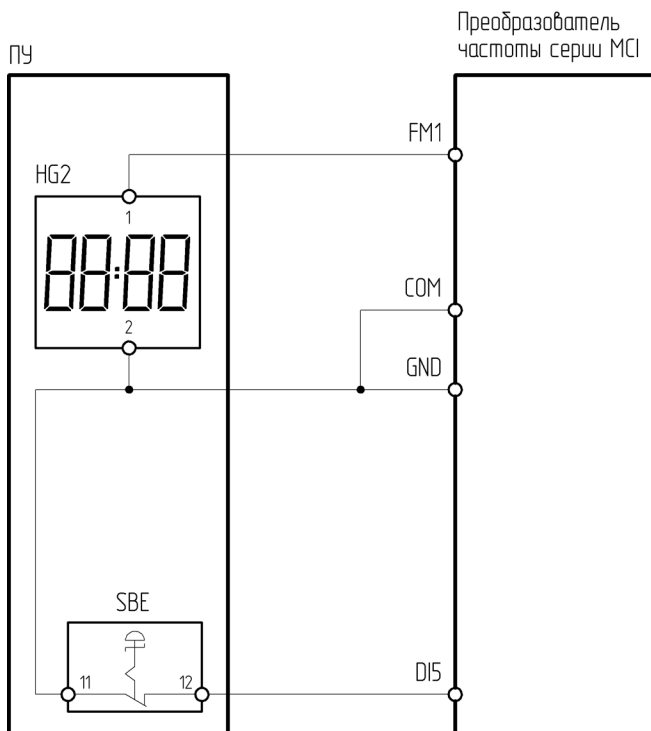
Рисунок 4.16.8 – Схема подключения ПУ-2-670 к преобразователю частоты серии МСІ
