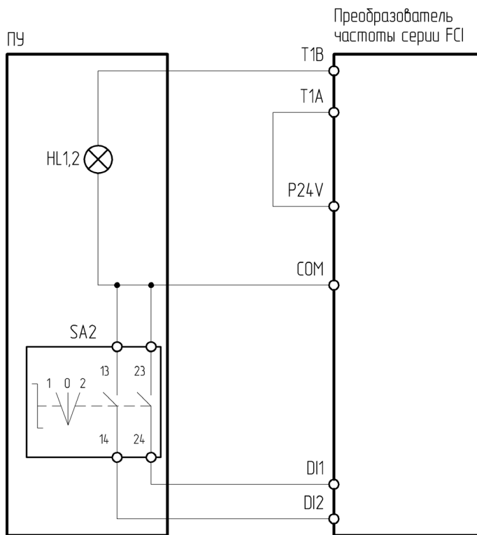
Рисунок 4.7.5 – Схема подключения ПУ-2-120, ПУ-2-420 к преобразователю частоты серии FCI
