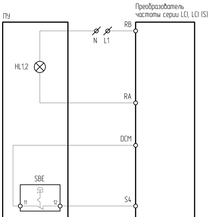
Рисунок 4.12.7 – Схема подключения ПУ-2-270, ПУ-2-570 к преобразователю частоты серии LCI/LCI(S)
