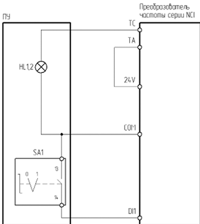
Рисунок 4.6.4 – Схема подключения ПУ-2-110, ПУ-2-410 к преобразователю частоты серии NCI
