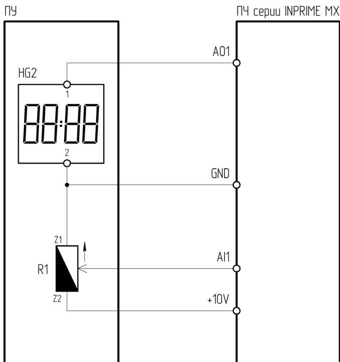
Рисунок 4.13.7 – Схема подключения ПУ-2-601 к преобразователю частоты серии INPRIME MX
