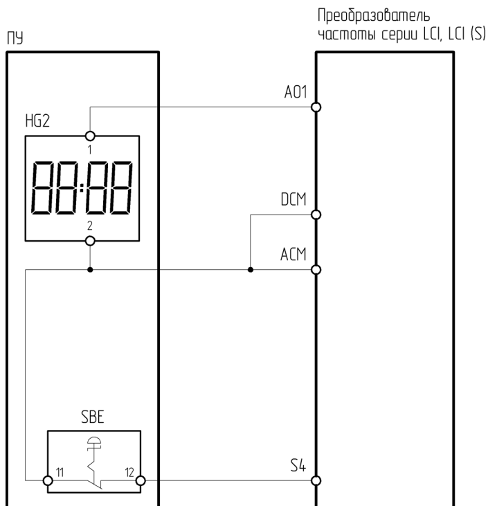
Рисунок 4.16.7 – Схема подключения ПУ-2-670 к преобразователю частоты серии LCI/LCI(S)
