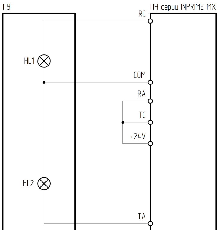
Рисунок 4.17.6 – Схема подключения ПУ-2-700 к преобразователю частоты серии INPRIME MX
