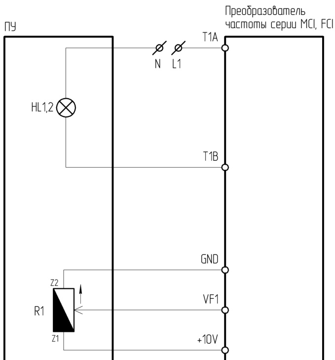
Рисунок 4.9.5 – Схема подключения ПУ-2-201, ПУ-2-501 к преобразователю частоты серии МСІ/FCІ
