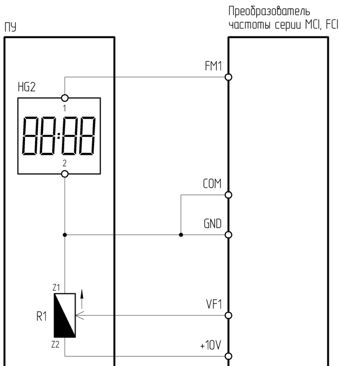
Рисунок 4.13.5 – Схема подключения ПУ-2-601 к преобразователю частоты серии MCI/FCI
