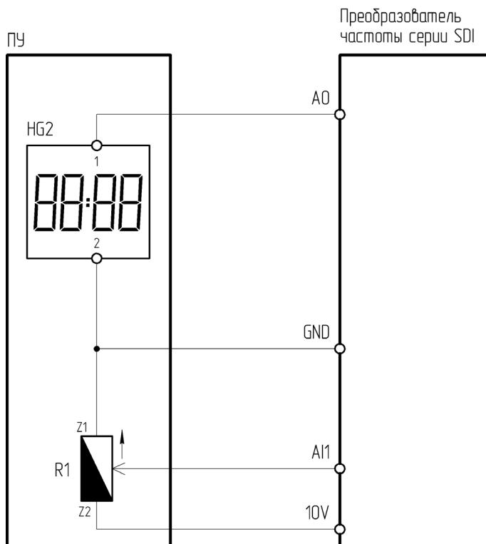
Рисунок 4.13.2 – Схема подключения ПУ-2-601 к преобразователю частоты серии SDI
