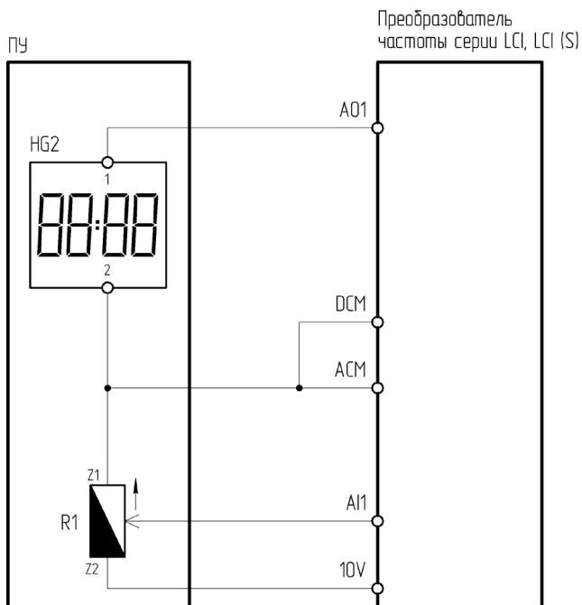
Рисунок 4.13.4 – Схема подключения ПУ-2-601 к преобразователю частоты серии LCI/LCI(S)
