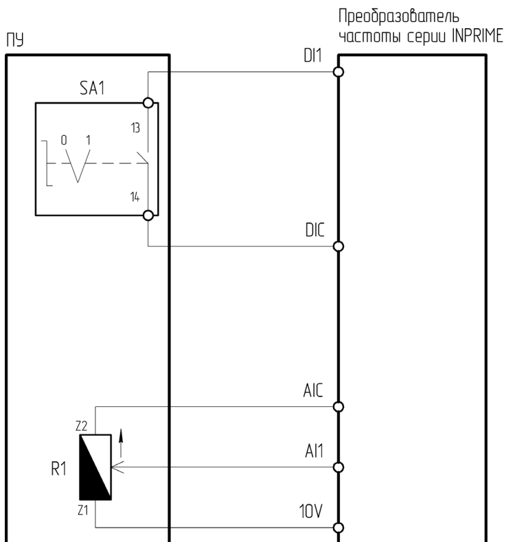
Рисунок 4.1.7 – Схема подключения ПУ-2-011 к преобразователю частоты серии INPRIME
