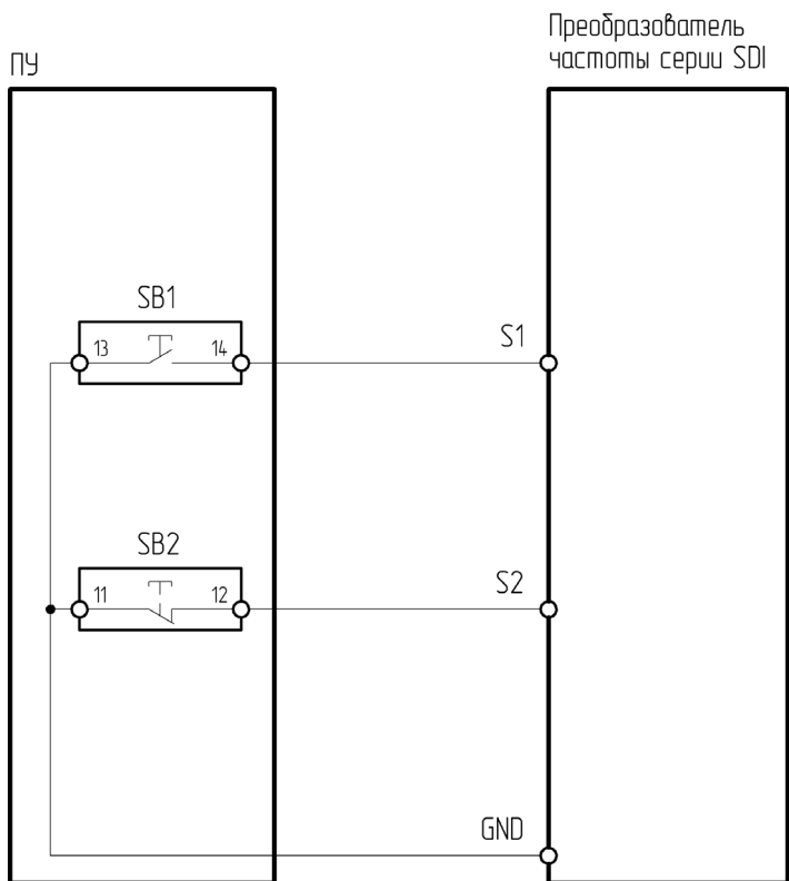
Рисунок 4.3.6 – Схема подключения ПУ-2-030 к преобразователю частоты серии SDI
