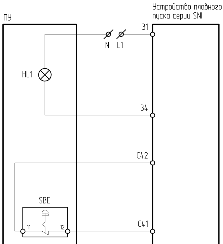
Рисунок 4.12.3а – Схема подключения ПУ-2-270 к устройству плавного пуска серии SNI
