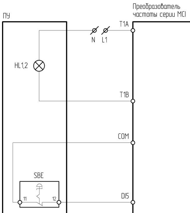
Рисунок 4.12.8 – Схема подключения ПУ-2-270, ПУ-2-570 к преобразователю частоты серии MCI
