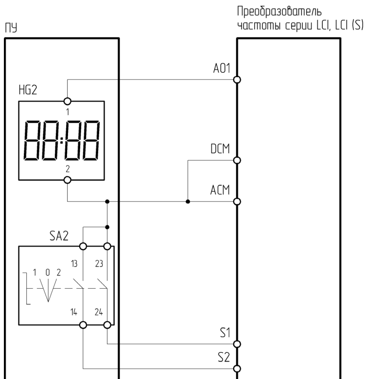
Рисунок 4.15.4 – Схема подключения ПУ-2-620 к преобразователю частоты серии LCI/LCI(S)
