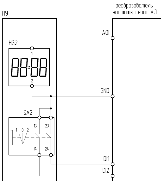
Рисунок 4.15.1 – Схема подключения ПУ-2-620 к преобразователю частоты серии VCI
