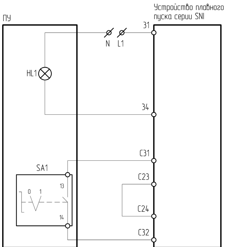
Рисунок 4.10.4а – Схема подключения ПУ-2-210 к устройству плавного пуска серии SNI
