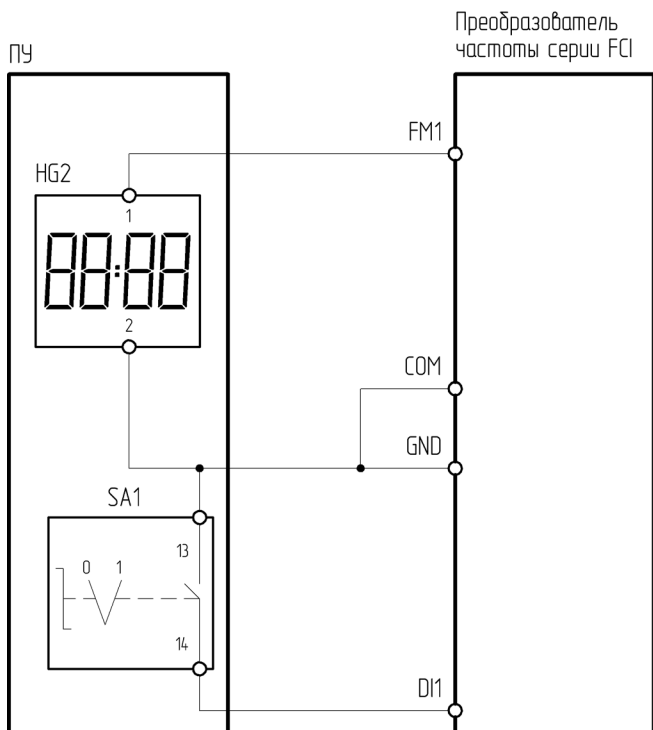
Рисунок 4.14.9 – Схема подключения ПУ-2-610 к преобразователю частоты серии FCI
