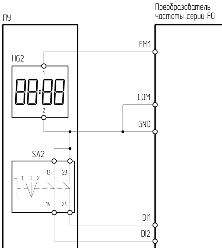
Рисунок 4.15.6 – Схема подключения ПУ-2-620 к преобразователю частоты серии FC1
