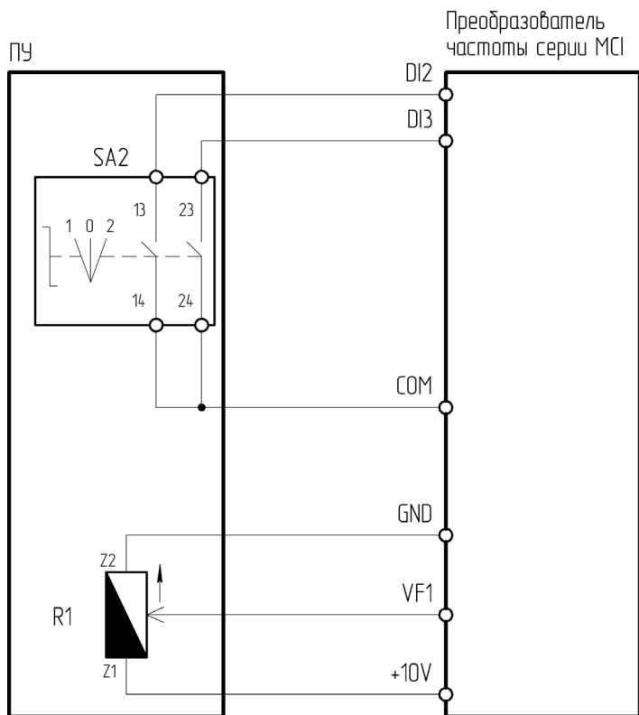
Рисунок 4.2.5 – Схема подключения ПУ-2-021 к преобразователю частоты серии МС1
