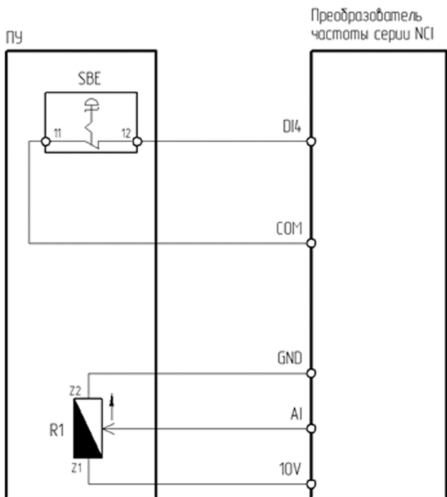
Рисунок 4.4.3 – Схема подключения ПУ-2-071 к преобразователю частоты серии NCI
