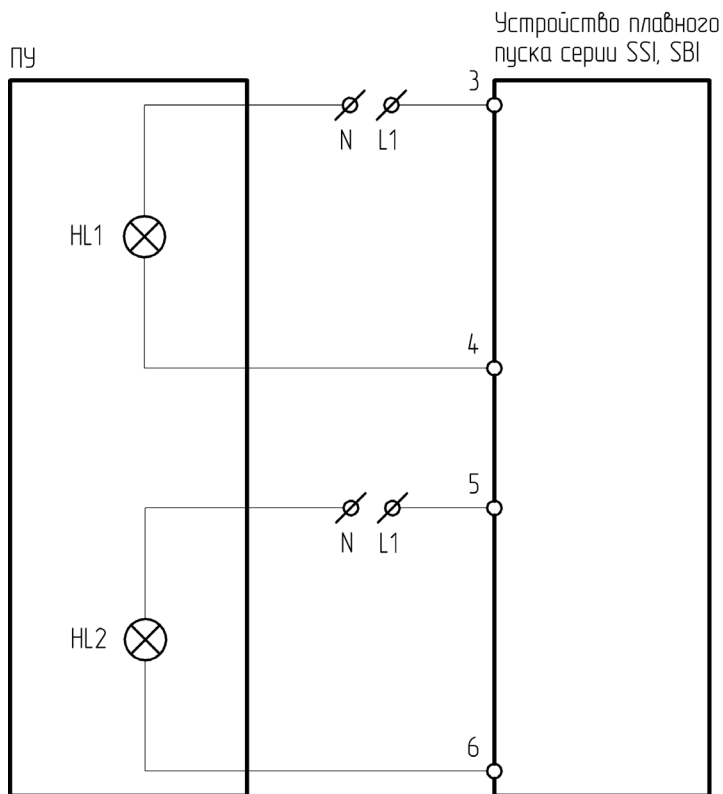
Рисунок 4.18.2 – Схема подключения ПУ-2-800 к устройству плавного пуска серии SSI/SBI
