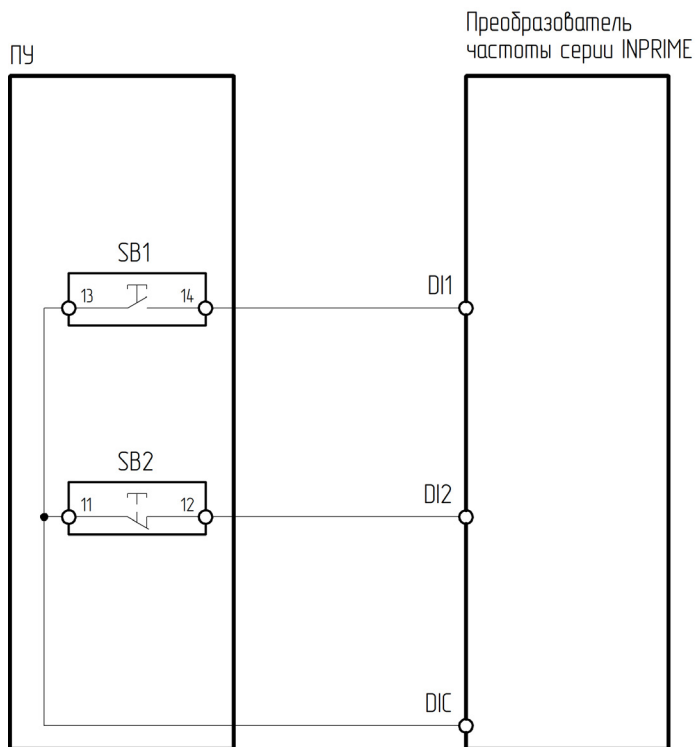
Рисунок 4.3.11 – Схема подключения ПУ-2-030 к преобразователю частоты серии INPRIME
