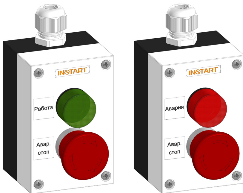
Рисунок 4.12 – Внешний вид ПУ-2-270, ПУ-2-570
