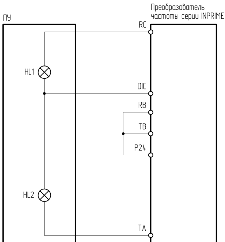
Рисунок 4.17.5 – Схема подключения ПУ-2-700 к преобразователю частоты серии INPRIME
