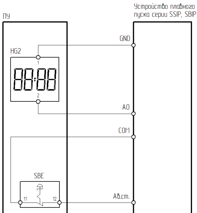
Рисунок 4.16.2 – Схема подключения ПУ-2-670 к устройству плавного пуска серии SSIP/SBIP
