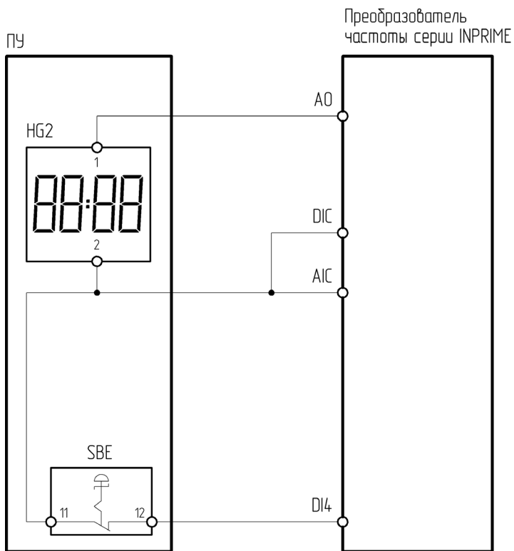
Рисунок 4.16.10 – Схема подключения ПУ-2-670 к преобразователю частоты серии INPRIME
