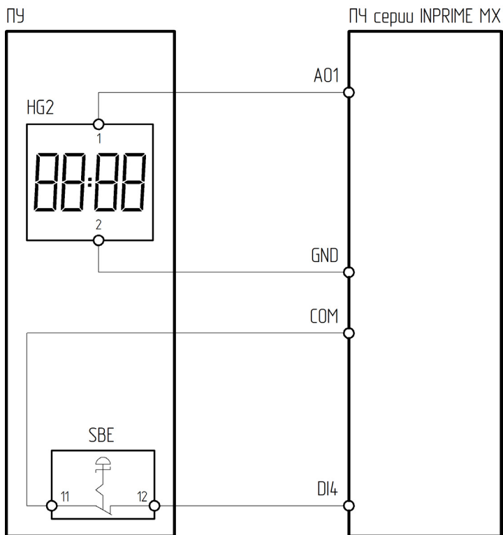
Рисунок 4.16.11 – Схема подключения ПУ-2-670 к преобразователю частоты серии INPRIME MX
