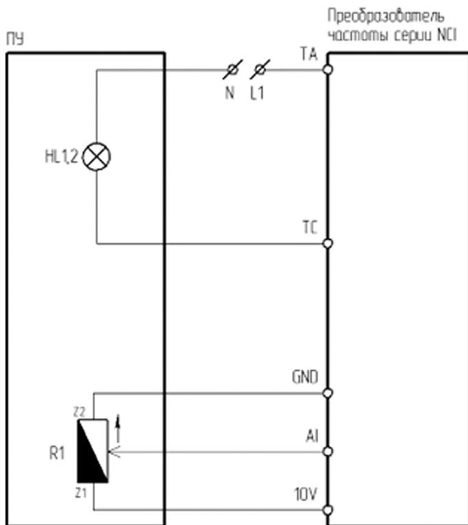
Рисунок 4.9.3 – Схема подключения ПУ-2-201/501 к преобразователю частоты серии NCI
