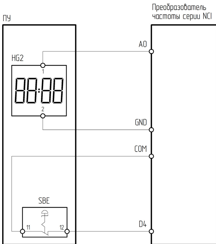
Рисунок 4.16.6 – Схема подключения ПУ-2-670 к преобразователю частоты серии NCI
