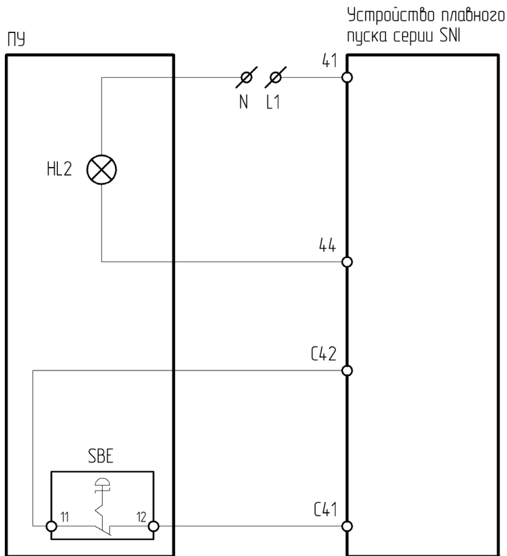
Рисунок 4.12.36 – Схема подключения ПУ-2-570 к устройству плавного пуска серии SNI
