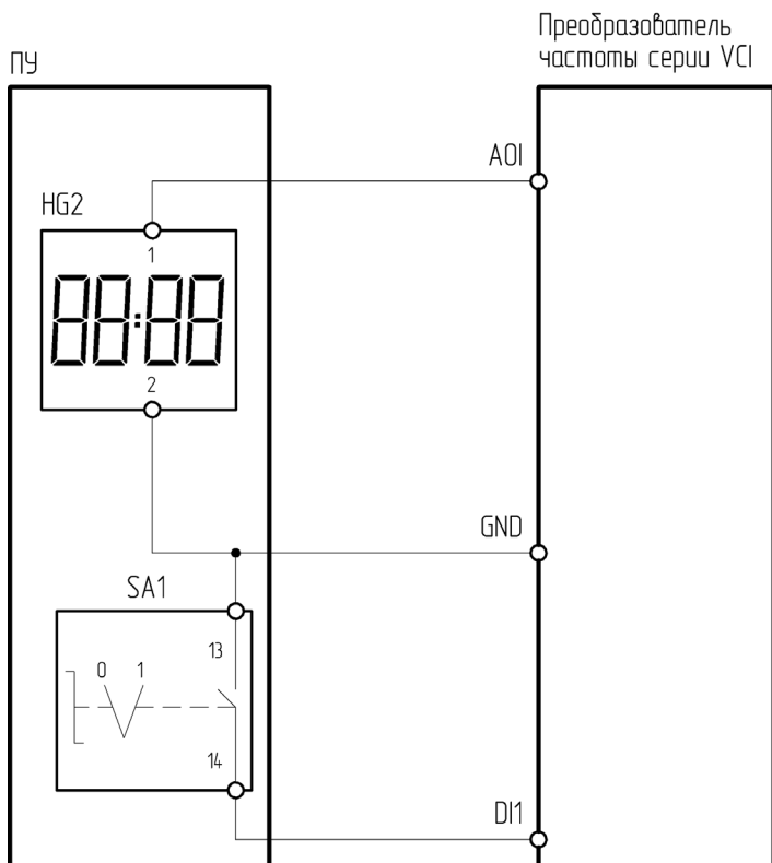
Рисунок 4.14.4 – Схема подключения ПУ-2-610 к преобразователю частоты серии VCI
