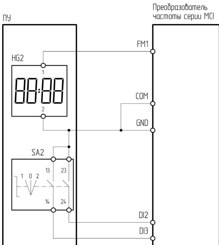
Рисунок 4.15.5 – Схема подключения ПУ-2-620 к преобразователю частоты серии MCI
