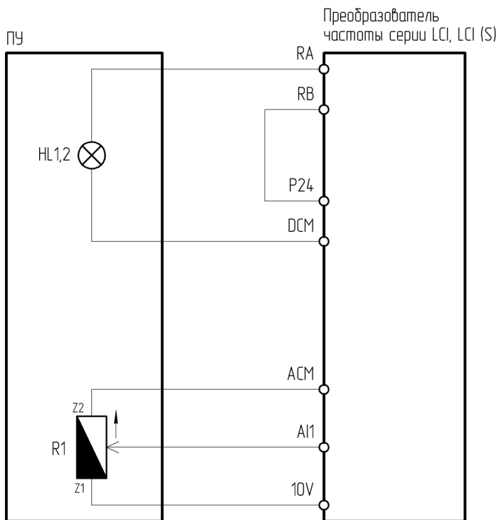
Рисунок 4.5.3 – Схема подключения ПУ-2-101, ПУ-2-401 к преобразователю частоты серии LCI/LCI(S)
