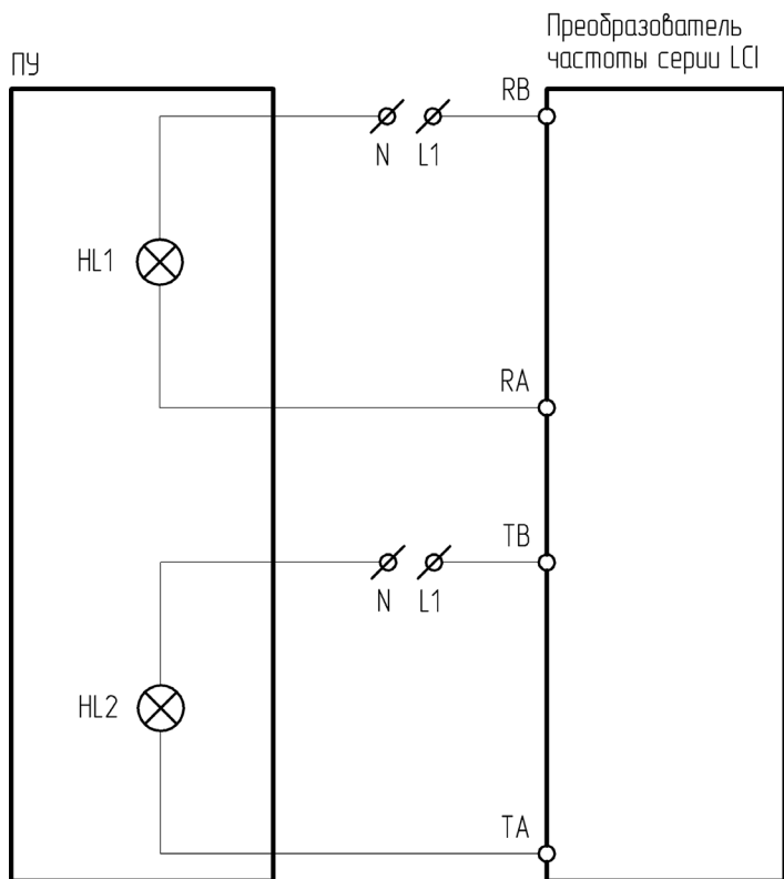
Рисунок 4.18.5 – Схема подключения ПУ-2-800 к преобразователю частоты серии LCI
