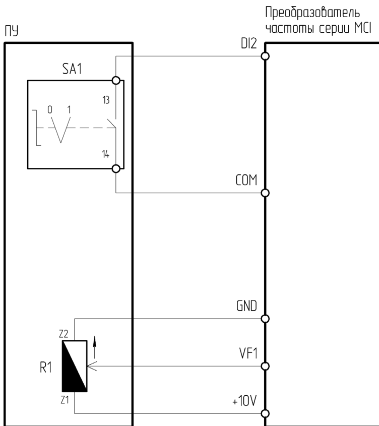
Рисунок 4.1.5 – Схема подключения ПУ-2-011 к преобразователю частоты серии МСІ
