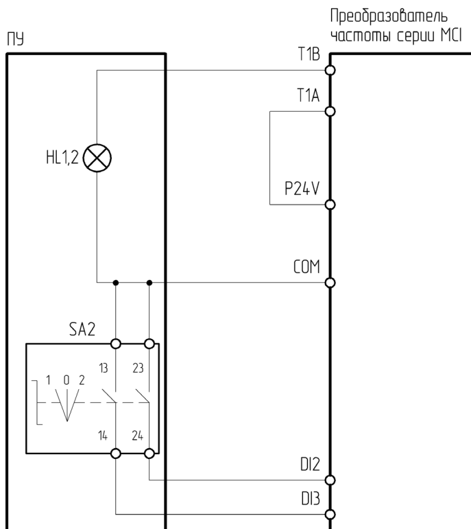
Рисунок 4.7.4 – Схема подключения ПУ-2-120, ПУ-2-420 к преобразователю частоты серии MCI
