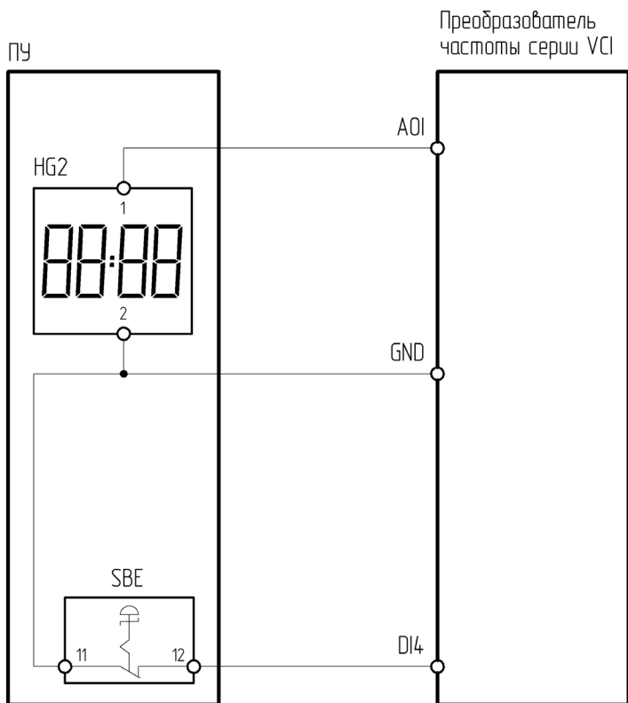
Рисунок 4.16.4 – Схема подключения ПУ-2-670 к преобразователю частоты серии VCI
