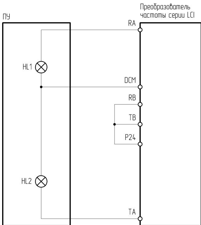
Рисунок 4.17.3 – Схема подключения ПУ-2-700 к преобразователю частоты серии LCI
