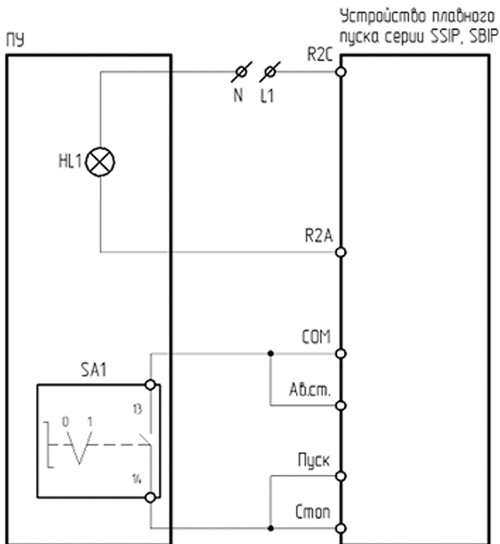
Рисунок 4.10.36 – Схема подключения ПУ-2-510 к устройству плавного пуска серии SSIP/SBIP
