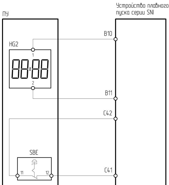
Рисунок 4.16.3 – Схема подключения ПУ-2-670 к устройству плавного пуска серии SNI
