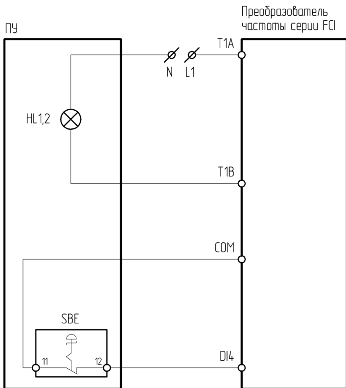
Рисунок 4.12.9 – Схема подключения ПУ-2-270, ПУ-2-570 к преобразователю частоты серии FCI
