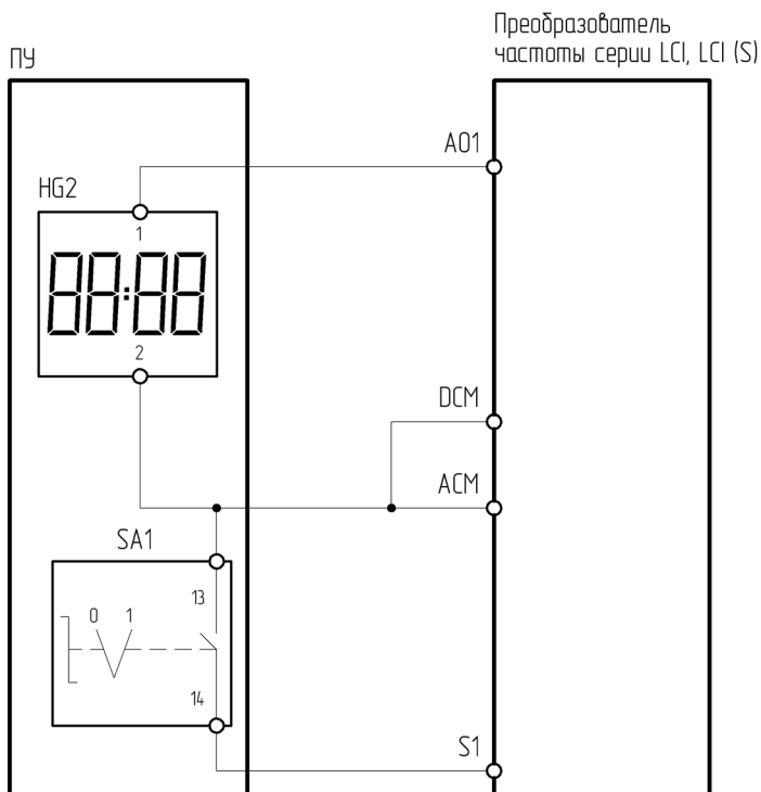
Рисунок 4.14.7 – Схема подключения ПУ-2-610 к преобразователю частоты серии LCI/LCI(S)
