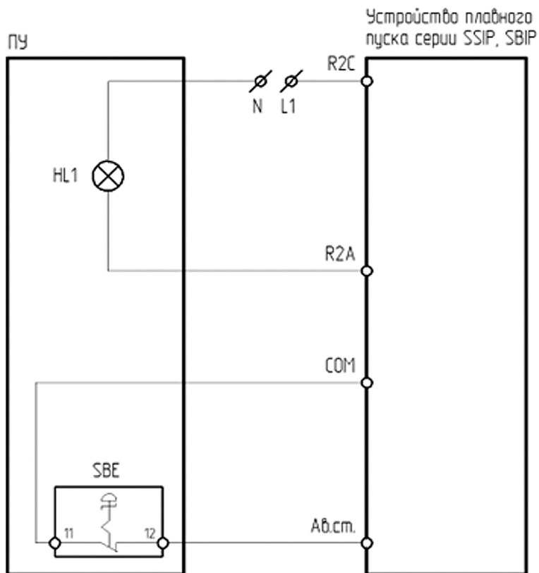
Рисунок 4.12.2а – Схема подключения ПУ-2-270 к устройству плавного пуска серии SSIP/SBIP
