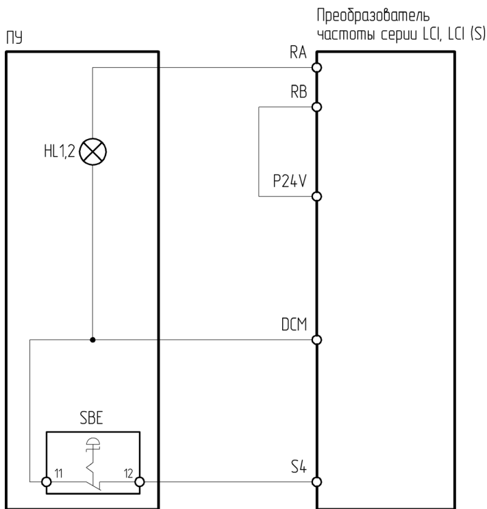
Рисунок 4.8.4 – Схема подключения ПУ-2-170, ПУ-2-470 к преобразователю частоты серии LCI/LCI(S)
