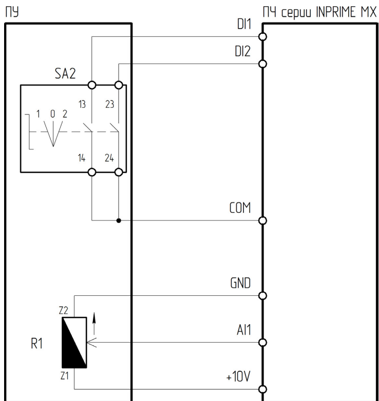
Рисунок 4.2.8 – Схема подключения ПУ-2-021 к преобразователю частоты серии INPRIME MX
