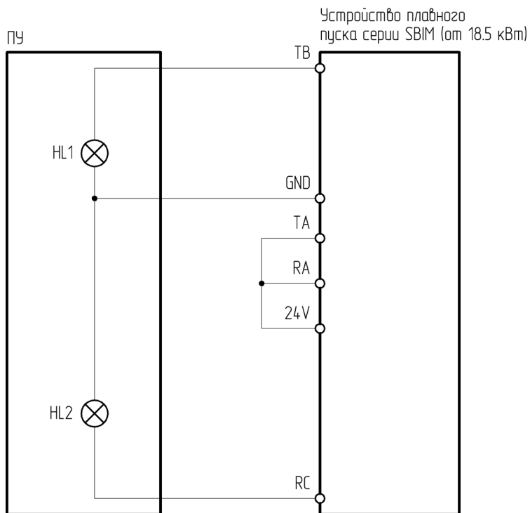
Рисунок 4.17.1 – Схема подключения ПУ-2-700 к устройству плавного пуска серии SBIM
