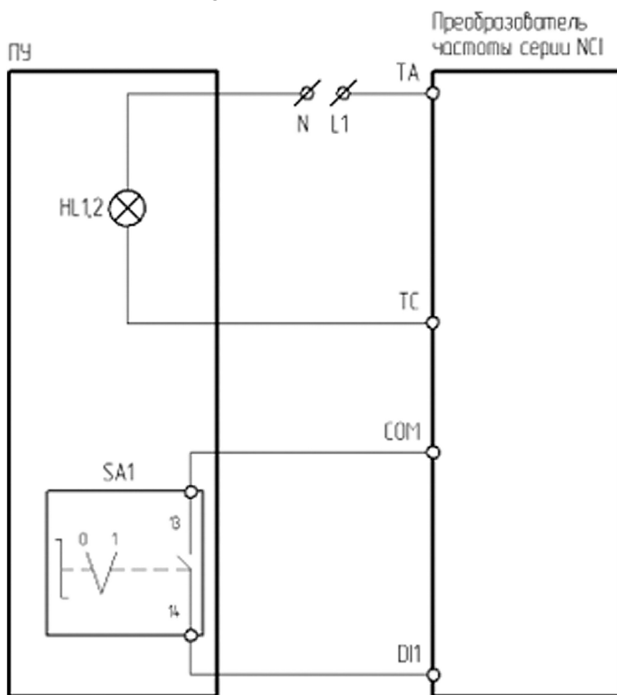
HL1 – лампа зеленая, HL2 – лампа красная
