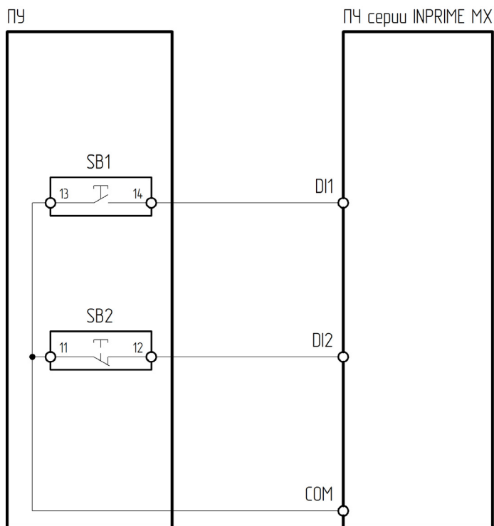
Рисунок 4.3.12 – Схема подключения ПУ-2-030 к преобразователю частоты серии INPRIME MX
