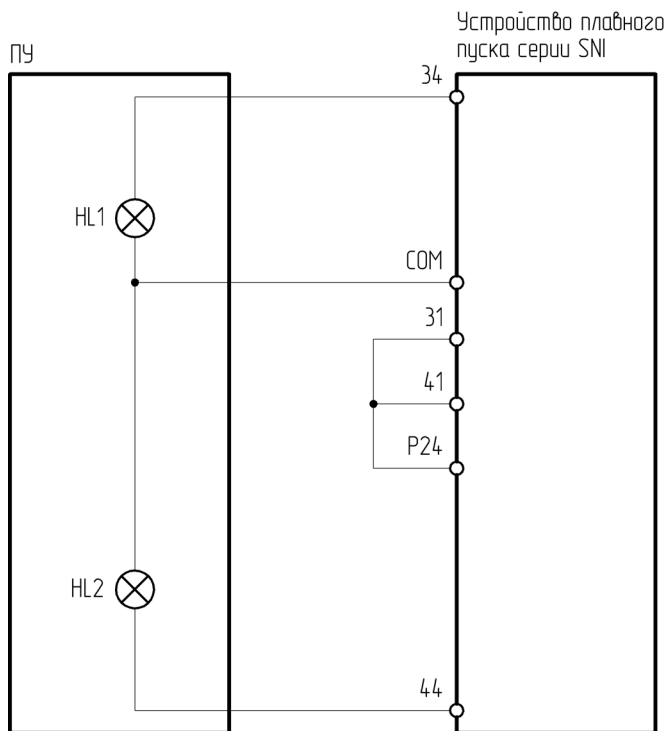
Рисунок 4.17.2 – Схема подключения ПУ-2-700 к устройству плавного пуска серии SNI
