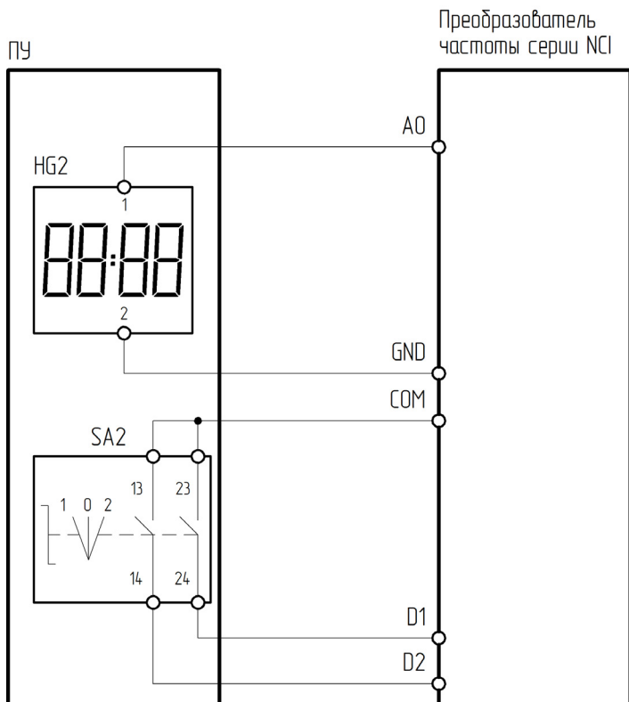
Рисунок 4.15.3 – Схема подключения ПУ-2-620 к преобразователю частоты серии NCI
