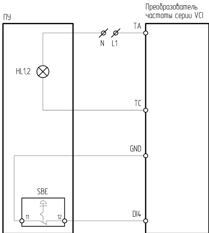
Рисунок 4.12.4 – Схема подключения ПУ-2-270, ПУ-2-570 к преобразователю частоты серии VCI
