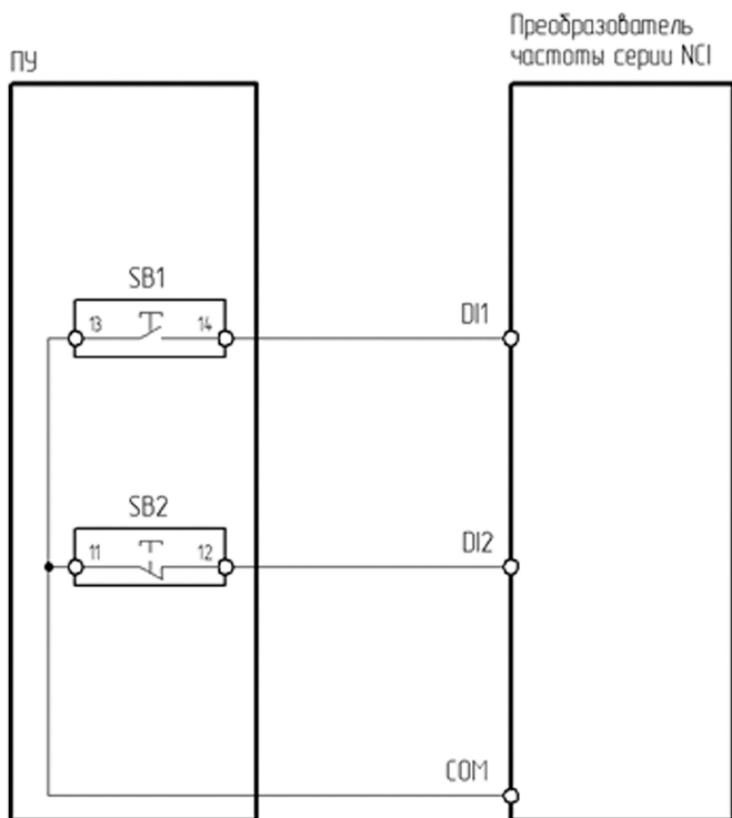
Рисунок 4.3.7 – Схема подключения ПУ-2-030 к преобразователю частоты серии NCI
