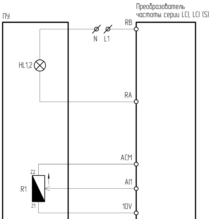
Рисунок 4.9.4 – Схема подключения ПУ-2-201, ПУ-2-501 к преобразователю частоты серии LCI/LCI(S)
