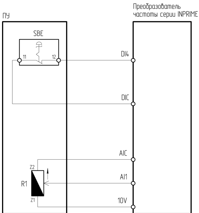
Рисунок 4.4.7 – Схема подключения ПУ-2-071 к преобразователю частоты серии INPRIME
