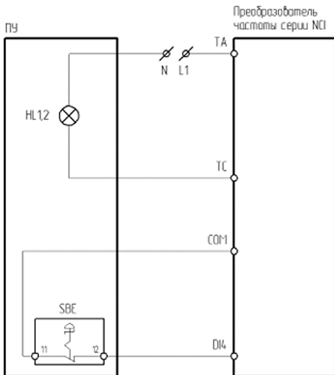
Рисунок 4.12.6 – Схема подключения ПУ-2-270, ПУ-2-570 к преобразователю частоты серии NCI
