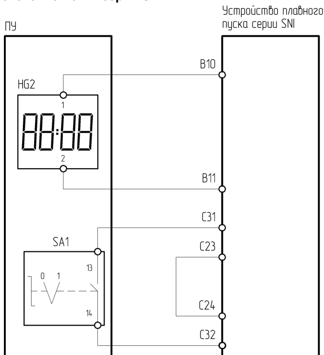
Рисунок 4.14.3 – Схема подключения ПУ-2-610 к устройству плавного пуска серии SNI
