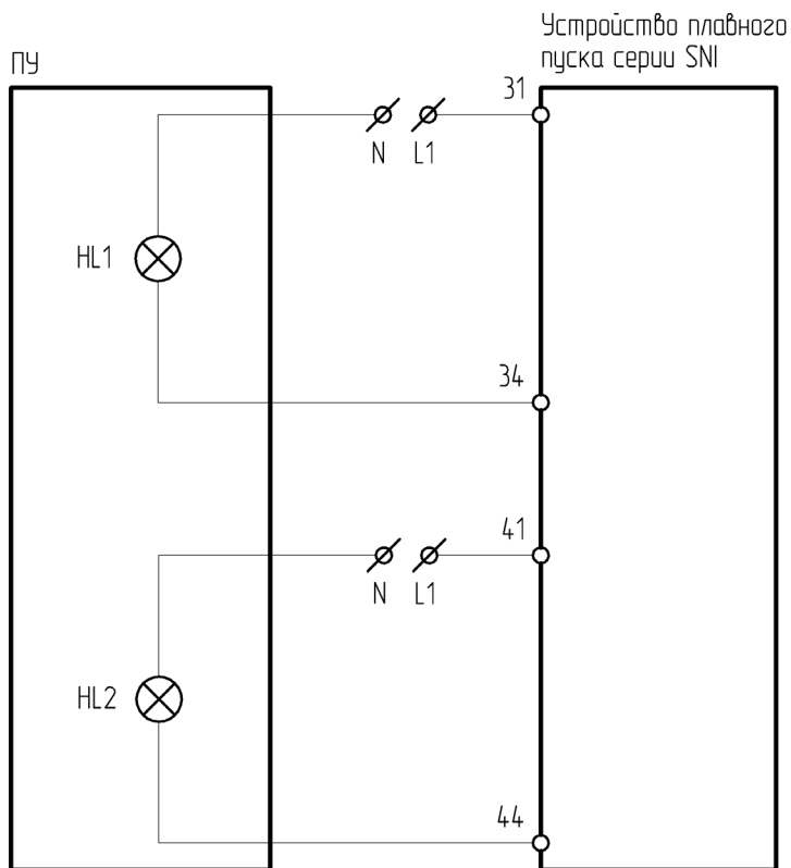
Рисунок 4.18.4 – Схема подключения ПУ-2-800 к устройству плавного пуска серии SNI
