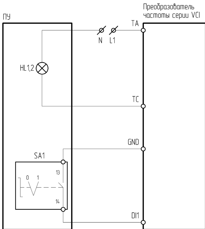
Рисунок 4.10.5 – Схема подключения ПУ-2-210, ПУ-2-510 к преобразователю частоты серии VCI
