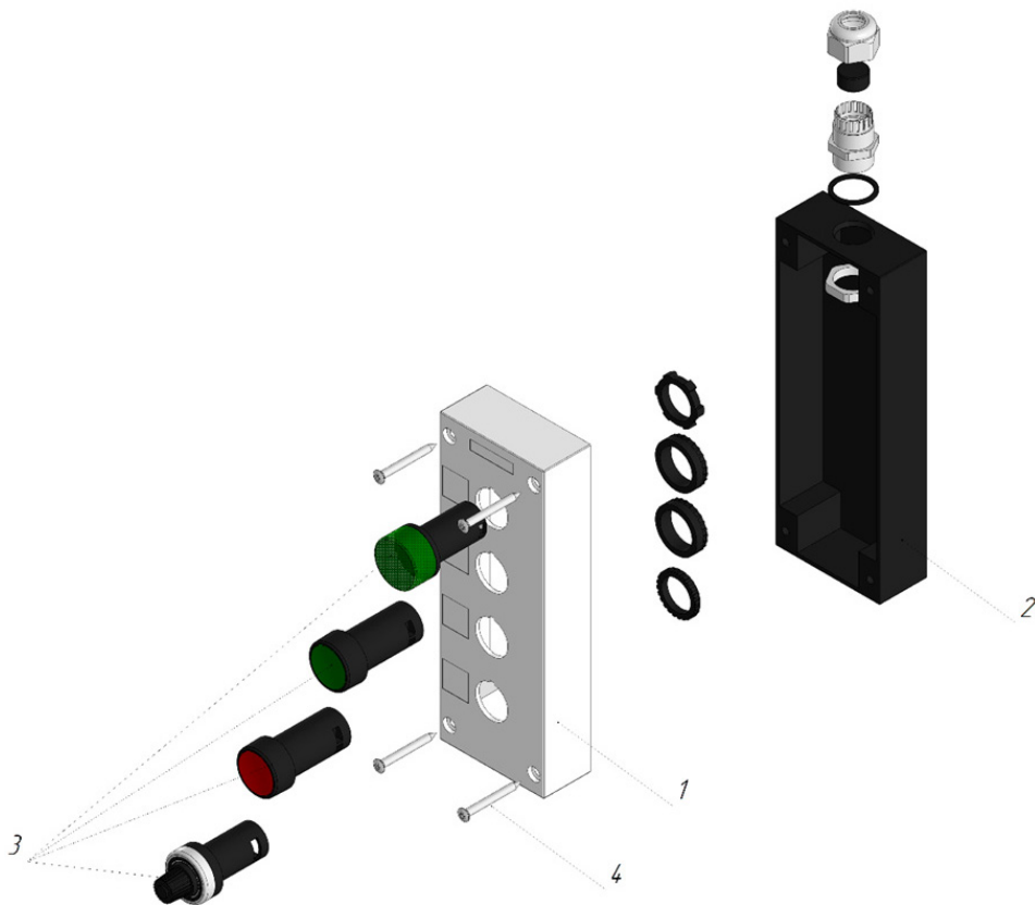
Рисунок 3.2.1 – 3D-модель пульта на примере ПУ-4-131
