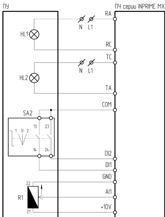
Рисунок 4.16.4 – Схема подключения ПУ-4-821 к преобразователю частоты серии INPRIME MX
