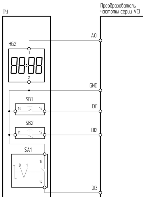
Рисунок 4.10.1 – Схема подключения ПУ-4-640 к преобразователю частоты серии VCI
