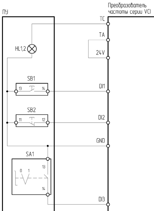
Рисунок 4.4.1 – Схема подключения ПУ-4-140, ПУ-4-440 к преобразователю частоты серии VCI
