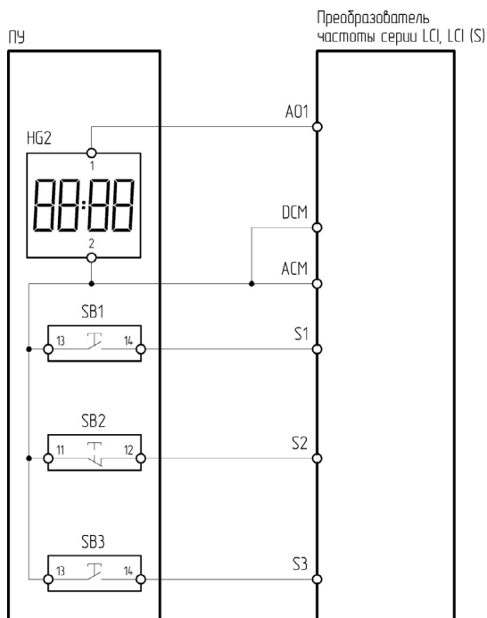
Рисунок 4.11.4 – Схема подключения ПУ-4-650 к преобразователю частоты серии LCI/LCI(S)
