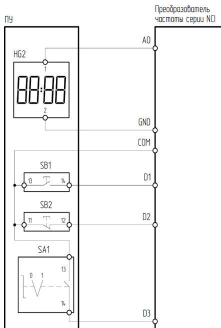
Рисунок 4.10.3 – Схема подключения ПУ-4-640 к преобразователю частоты серии NCI
