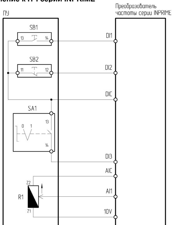
Рисунок 4.1.7 – Схема подключения ПУ-4-041 к преобразователю частоты серии INPRIME
