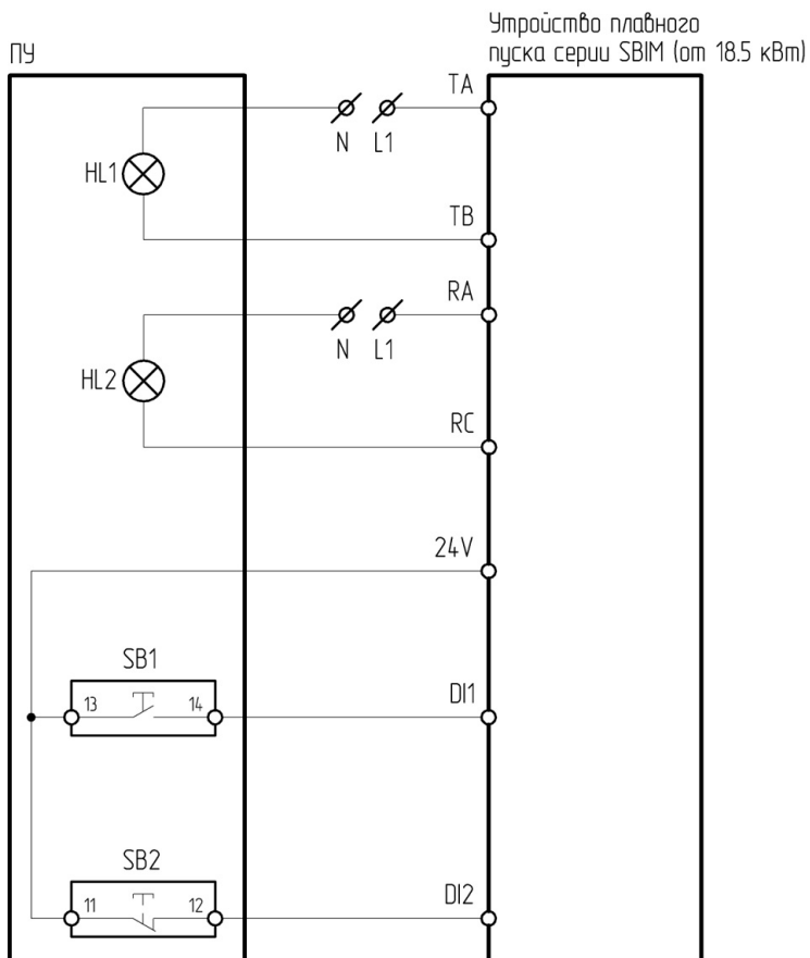
Рисунок 4.17.1 – Схема подключения ПУ-4-830 к устройству плавного пуска серии SBIM
