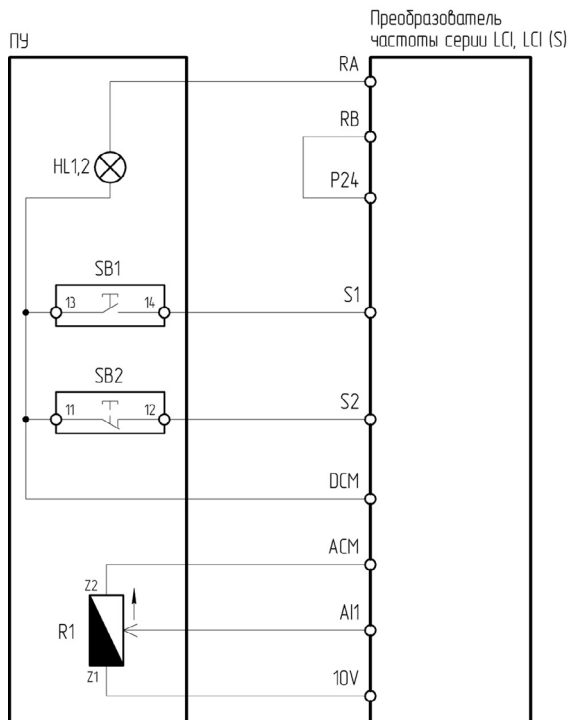
Рисунок 4.3.3 – Схема подключения ПУ-4-131, ПУ-4-431 к преобразователю частоты серии LCI/LCI(S)
