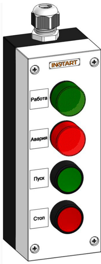
Рисунок 4.17 – Внешний вид ПУ-4-830
