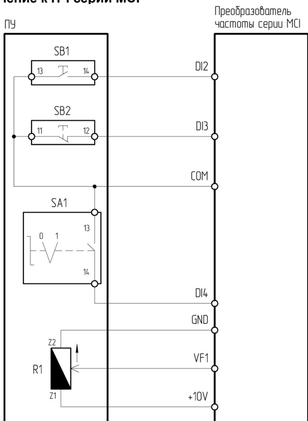
Рисунок 4.1.5 – Схема подключения ПУ-4-041 к преобразователю частоты серии МС1
