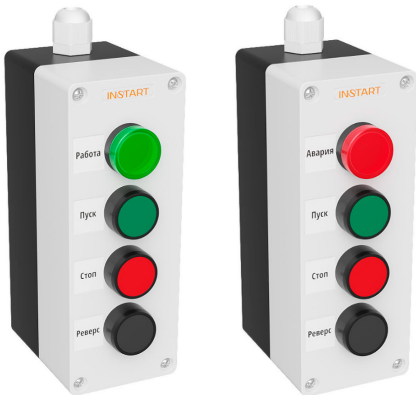
Рисунок 4.8 – Внешний вид ПУ-4-250, ПУ-4-550
