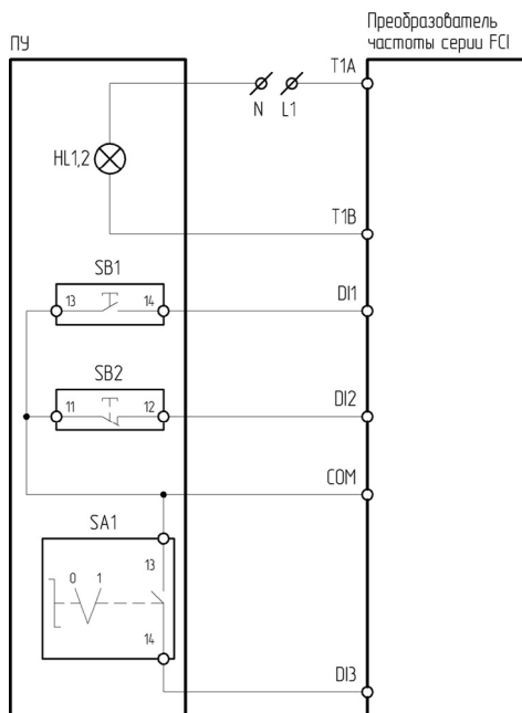
Рисунок 4.7.6 – Схема подключения ПУ-4-240, ПУ-4-540 к преобразователю частоты серии FCI
