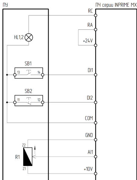
Рисунок 4.3.7 – Схема подключения ПУ-4-131, ПУ-4-431 к преобразователю частоты серии INPRIME MX
