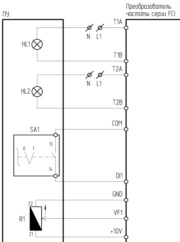
Рисунок 4.15.2 – Схема подключения ПУ-4-811 к преобразователю частоты серии FCI
