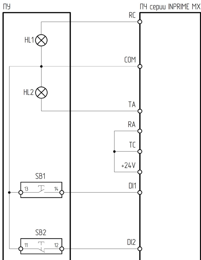
Рисунок 4.14.6 – Схема подключения ПУ-4-730 к преобразователю частоты серии INPRIME MX
