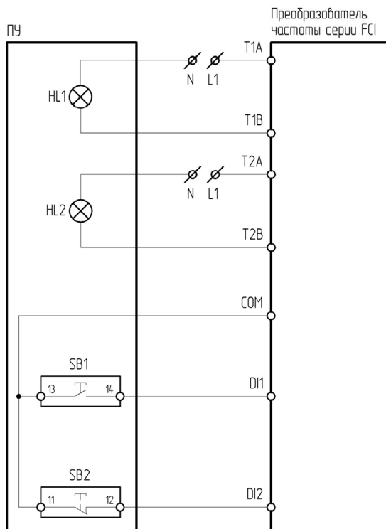
Рисунок 4.17.6 – Схема подключения ПУ-4-830 к преобразователю частоты серии FCI
