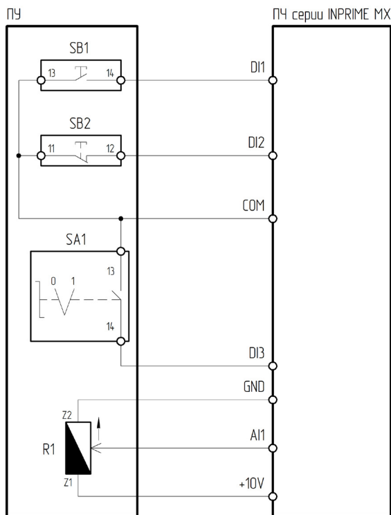
Рисунок 4.1.8 – Схема подключения ПУ-4-041 к преобразователю частоты серии INPRIME MX
