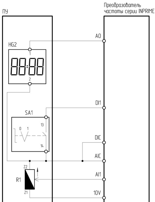
Рисунок 4.11.7 – Схема подключения ПУ-4-650 к преобразователю частоты серии INPRIME
