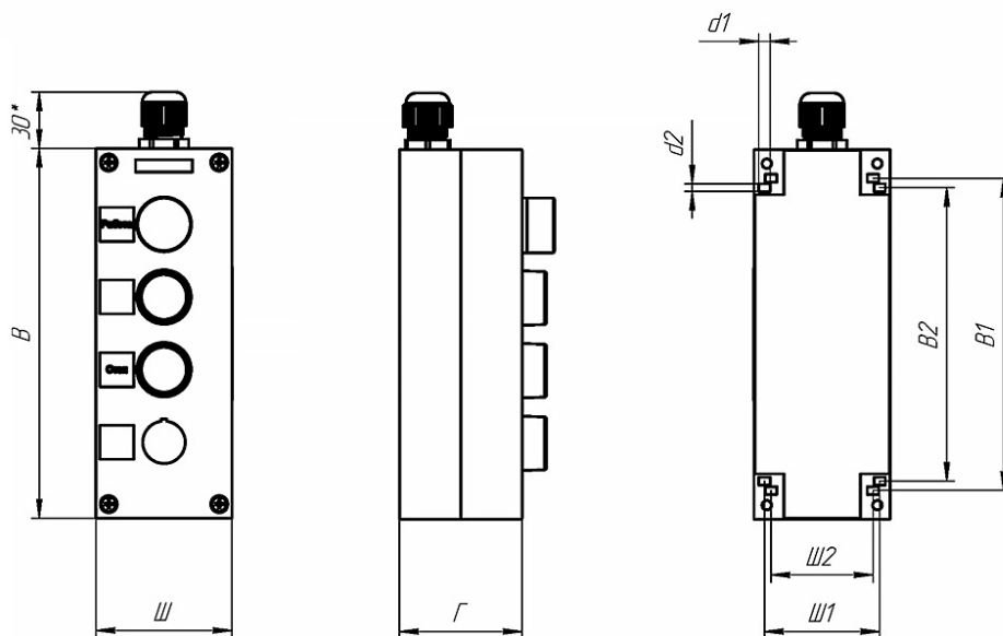
Рисунок 2.4.1 – Внешний вид и габаритные размеры пульта управления серии ПУ-4
