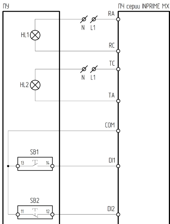
Рисунок 4.17.7 – Схема подключения ПУ-4-830 к преобразователю частоты серии INPRIME
