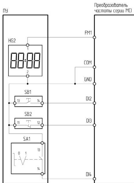
Рисунок 4.10.5 – Схема подключения ПУ-4-640 к преобразователю частоты серии МС1
