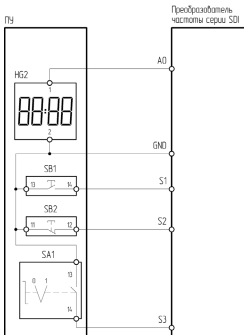
Рисунок 4.10.2 – Схема подключения ПУ-4-640 к преобразователю частоты серии SDI
