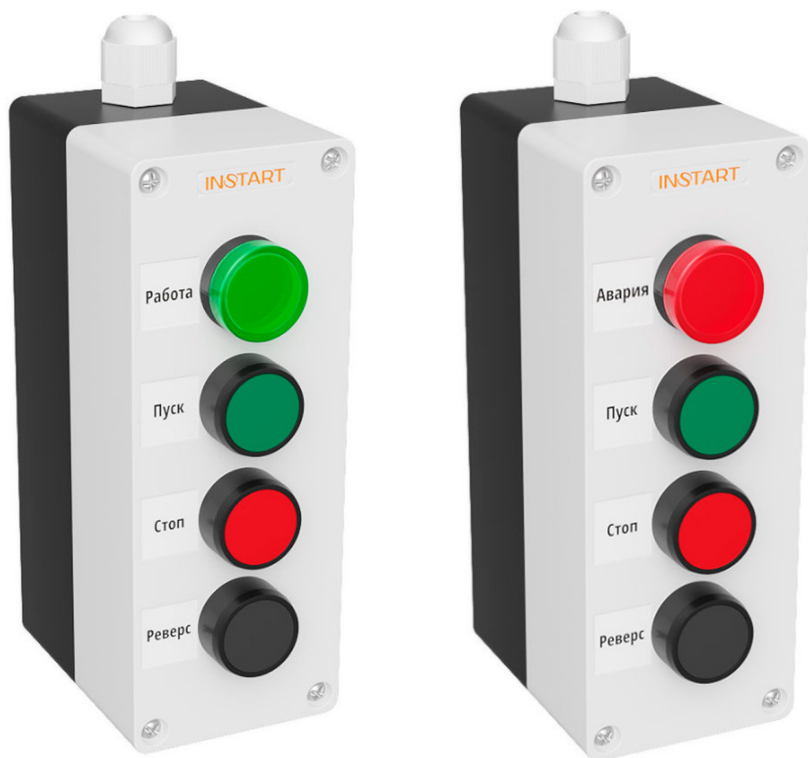
Рисунок 4.5 – Внешний вид ПУ-4-150, ПУ-4-450
