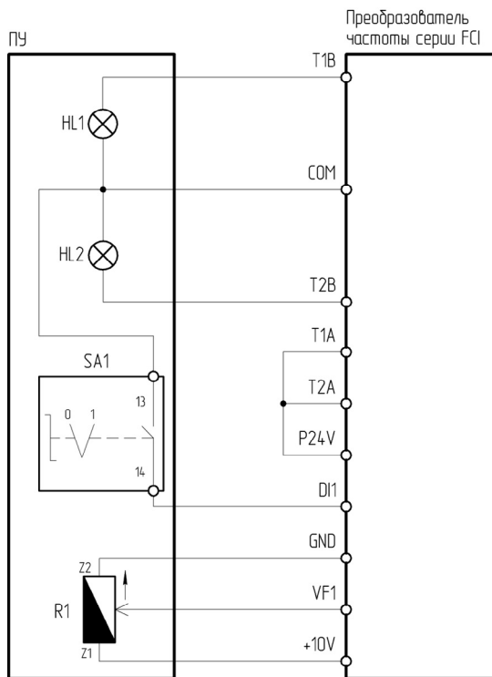
Рисунок 4.12.2 – Схема подключения ПУ-4-711 к преобразователю частоты серии FCI
