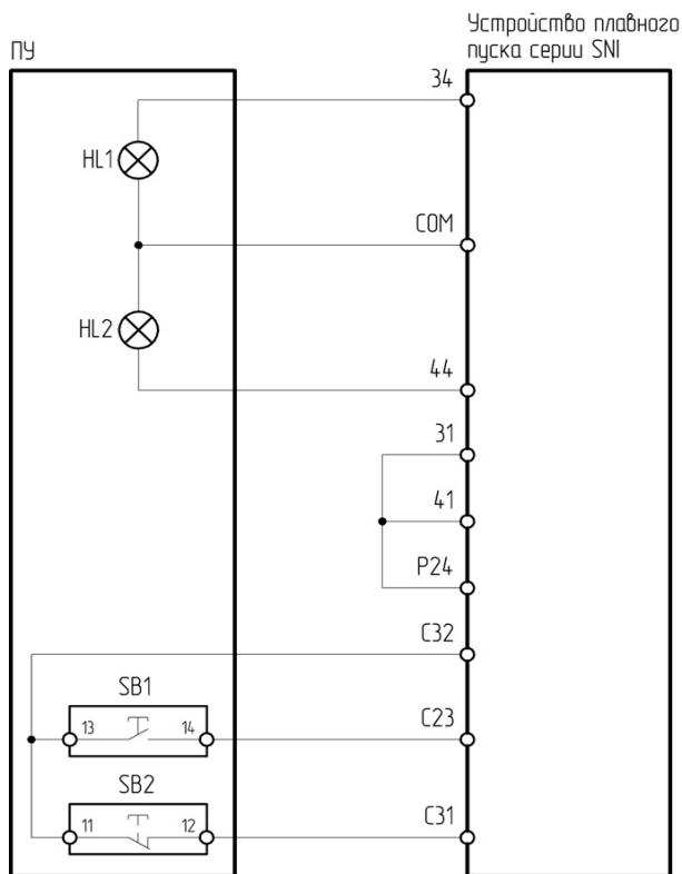
Рисунок 4.14.2 – Схема подключения ПУ-4-730 к устройству плавного пуска серии SNI
