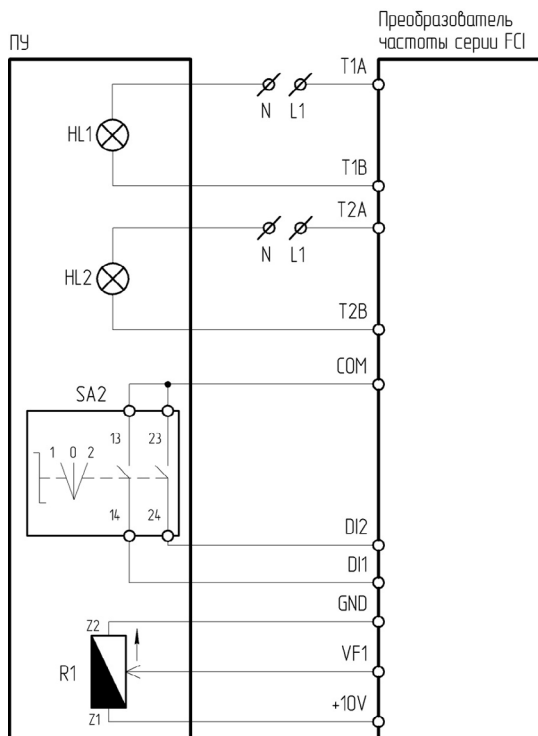
Рисунок 4.16.2 – Схема подключения ПУ-4-821 к преобразователю частоты серии FCI
