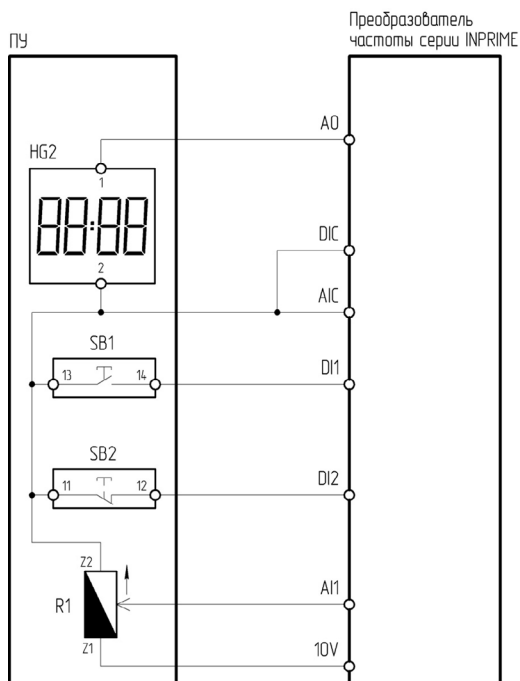
Рисунок 4.9.7 – Схема подключения ПУ-4-631 к преобразователю частоты серии INPRIME
