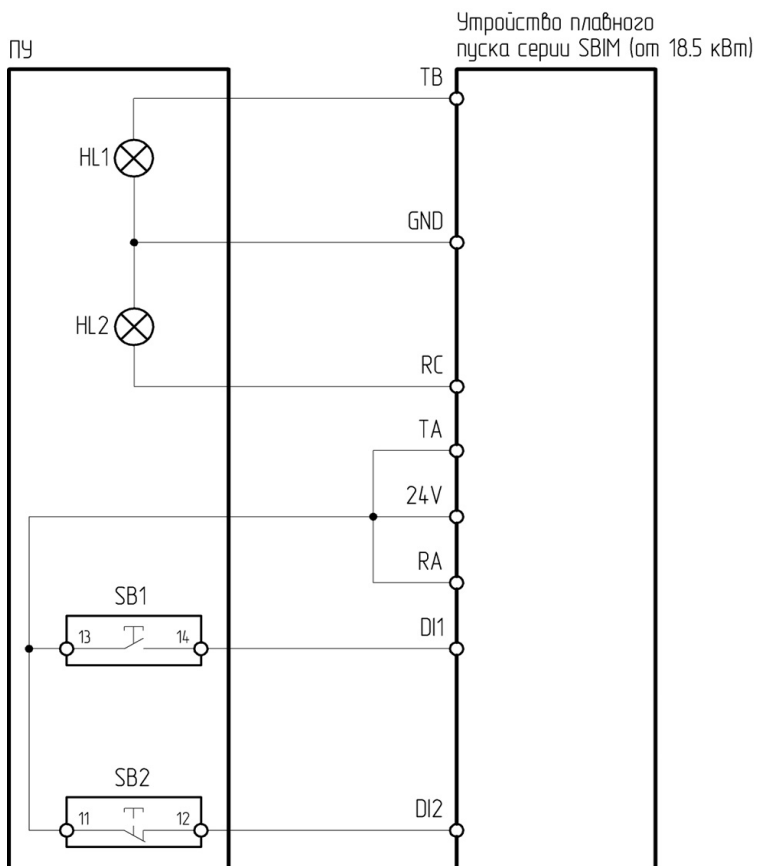
Рисунок 4.14.1 – Схема подключения ПУ-4-730 к устройству плавного пуска серии SBIM
