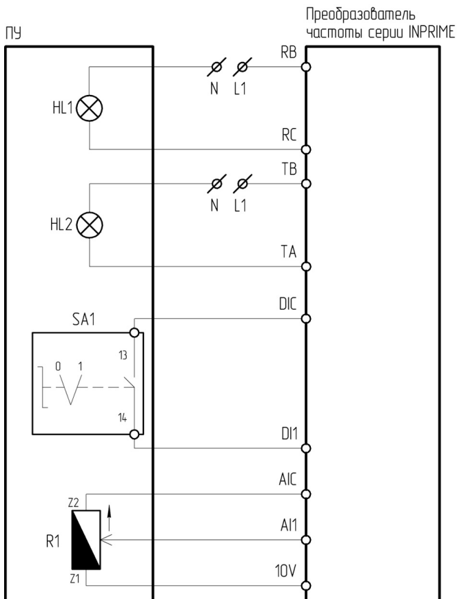
Рисунок 4.15.3 – Схема подключения ПУ-4-811 к преобразователю частоты серии INPRIME
