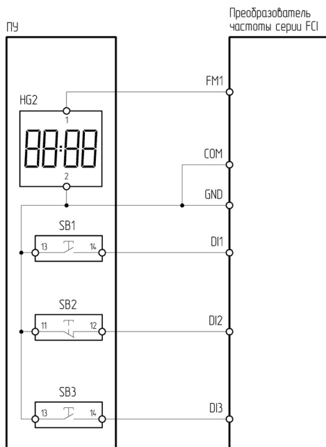
Рисунок Рисунок 4.11.6 – Схема подключения ПУ-4-650 к преобразователю частоты серии FCI
