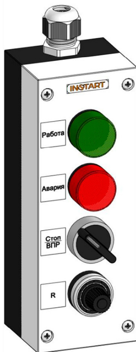
Рисунок 4.15 – Внешний вид ПУ-4-811
