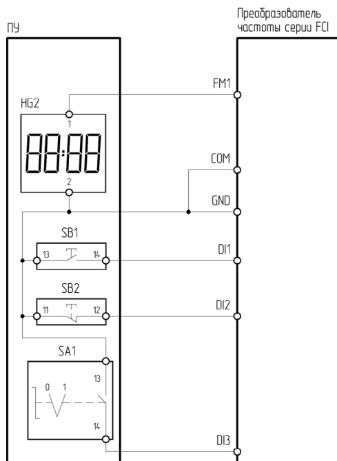
Рисунок 4.10.6 – Схема подключения ПУ-4-640 к преобразователю частоты серии FC1
