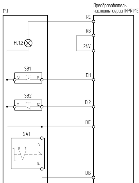
Рисунок 4.4.6 – Схема подключения ПУ-4-140, ПУ-4-440 к преобразователю частоты серии INPRIME
