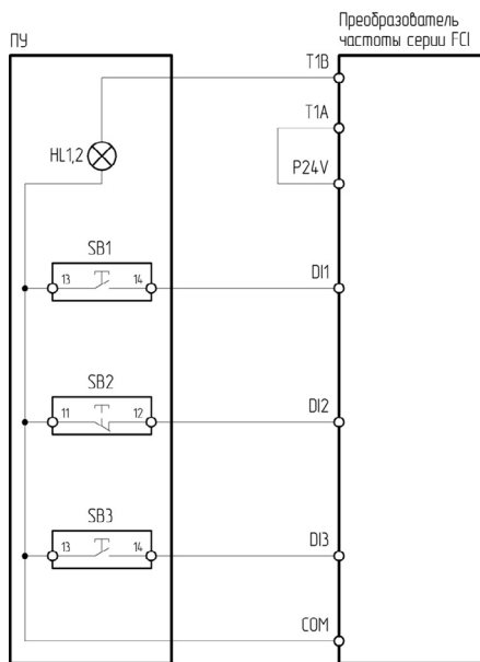
Рисунок 4.5.5 – Схема подключения ПУ-4-150, ПУ-4-450 к преобразователю частоты серии FCI
