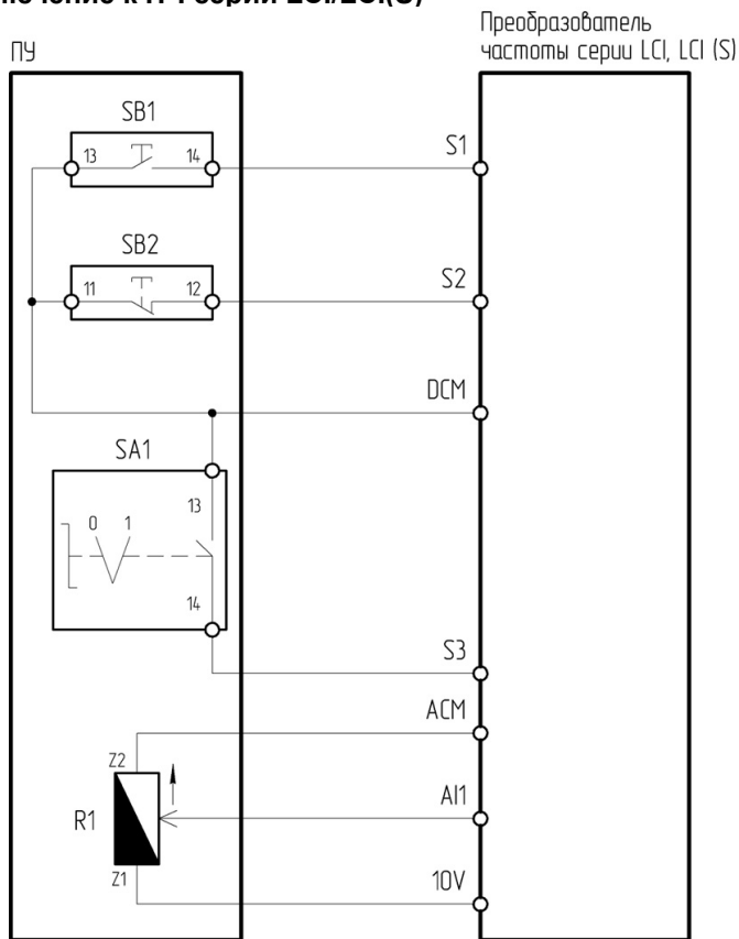
Рисунок 4.1.4 – Схема подключения ПУ-4-041 к преобразователю частоты серии LCI/LCI(S)
