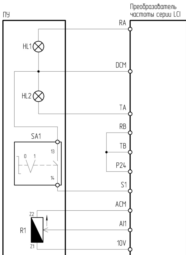
Рисунок 4.12.1 – Схема подключения ПУ-4-711 к преобразователю частоты серии LCI
