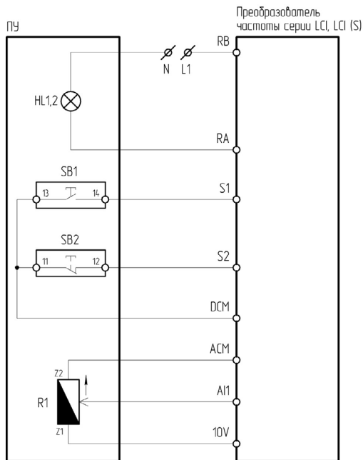
Рисунок 4.6.4 – Схема подключения ПУ-4-231, ПУ-4-531 к преобразователю частоты серии LCI/LCI(S)
