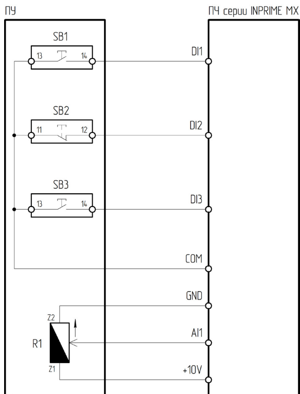
Рисунок 4.2.8 – Схема подключения ПУ-4-051 к преобразователю частоты серии INPRIME MX
