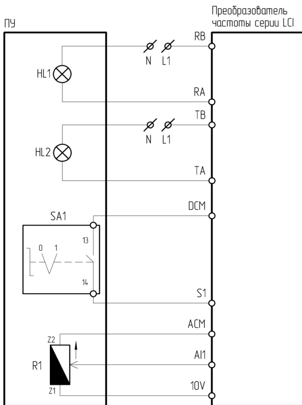
Рисунок 4.15.1 – Схема подключения ПУ-4-811 к преобразователю частоты серии LCI
