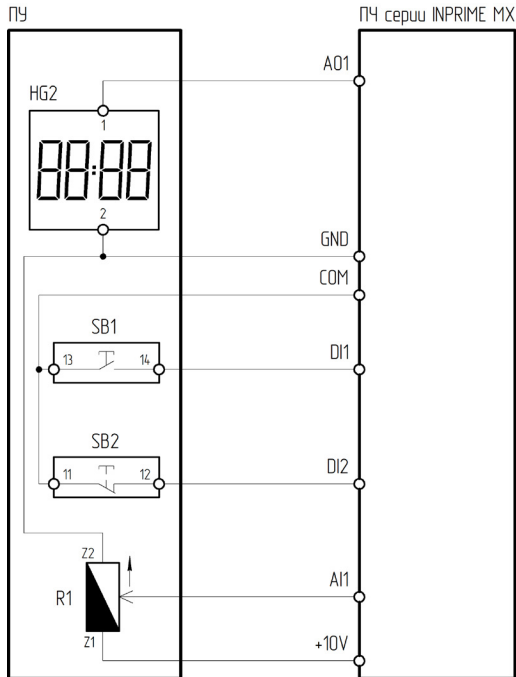
Рисунок 4.9.9 – Схема подключения ПУ-4-631 к преобразователю частоты серии INPRIME MX
