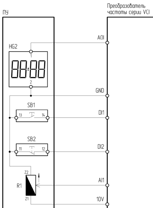
Рисунок 4.9.1 – Схема подключения ПУ-4-631 к преобразователю частоты серии VCI
