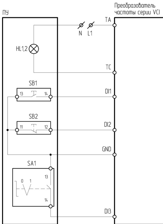
Рисунок 4.7.1 – Схема подключения ПУ-4-240, ПУ-4-540 к преобразователю частоты серии VCI
