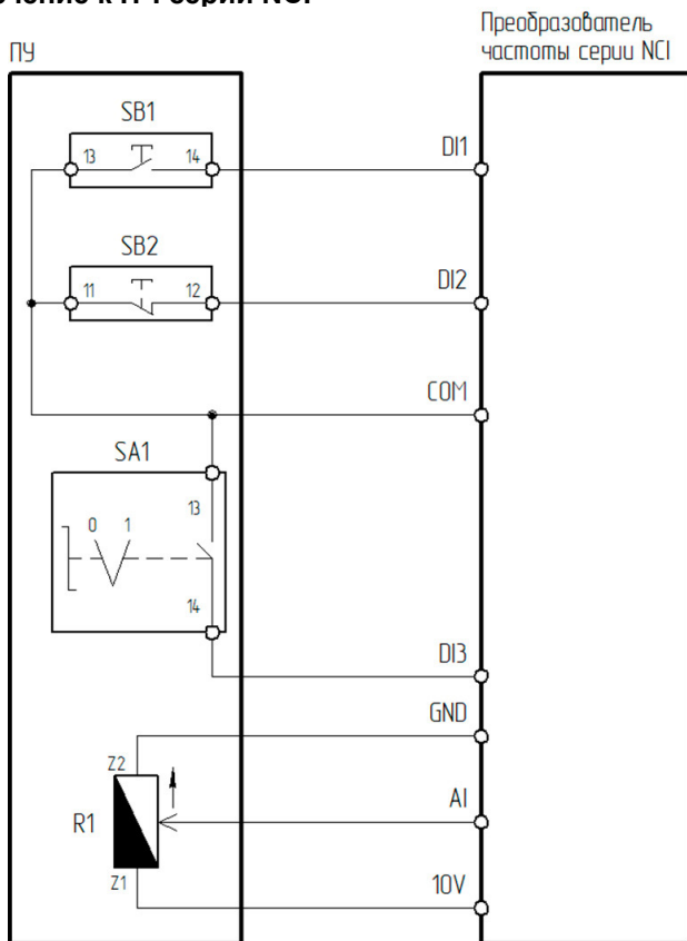
Рисунок 4.1.3 – Схема подключения ПУ-4-041 к преобразователю частоты серии NCI
