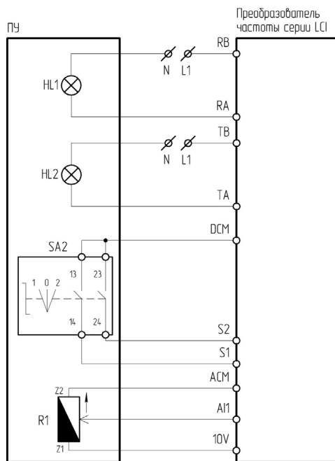
Рисунок 4.16.1 – Схема подключения ПУ-4-821 к преобразователю частоты серии LCI
