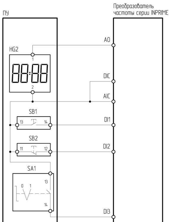
Рисунок 4.10.7 – Схема подключения ПУ-4-640 к преобразователю частоты серии INPRIME
