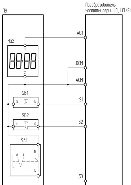
Рисунок 4.10.4 – Схема подключения ПУ-4-640 к преобразователю частоты серии LCI/LCI(S)
