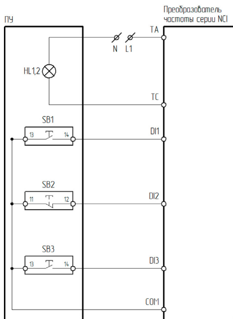
Рисунок 4.8.3 – Схема подключения ПУ-4-250, ПУ-4-550 к преобразователю частоты серии NCI
