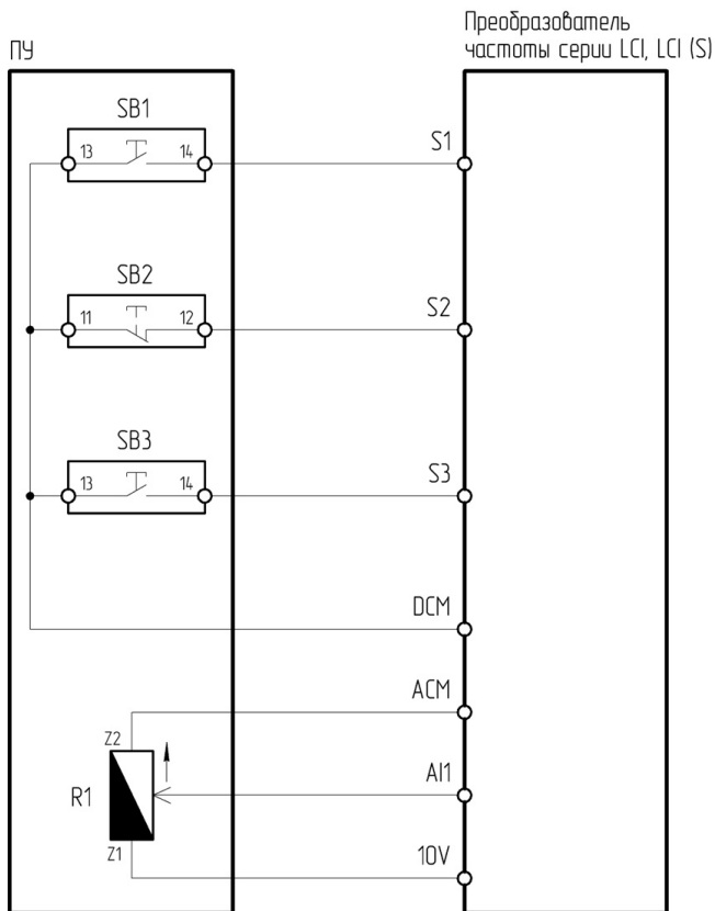
Рисунок 4.2.4 – Схема подключения ПУ-4-051 к преобразователю частоты серии LCI/LCI(S)
