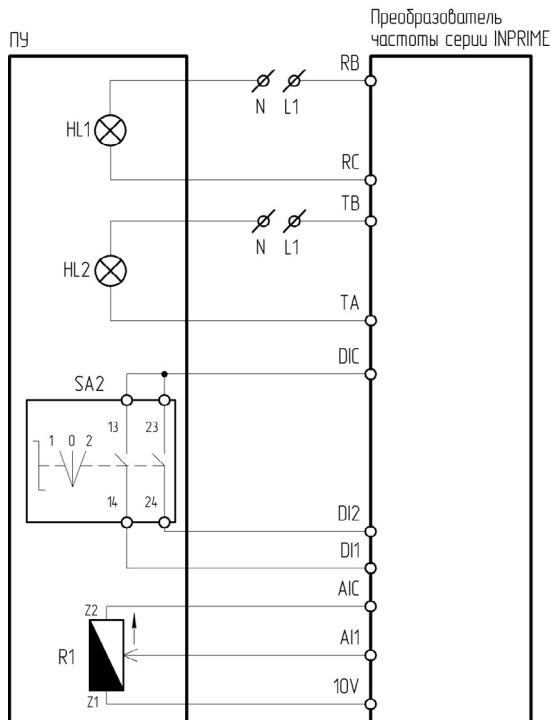
Рисунок 4.16.3 – Схема подключения ПУ-4-821 к преобразователю частоты серии INPRIME
