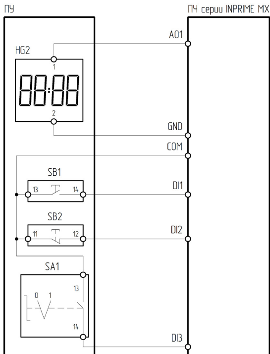
Рисунок 4.10.8 – Схема подключения ПУ-4-640 к преобразователю частоты серии INPRIME MX
