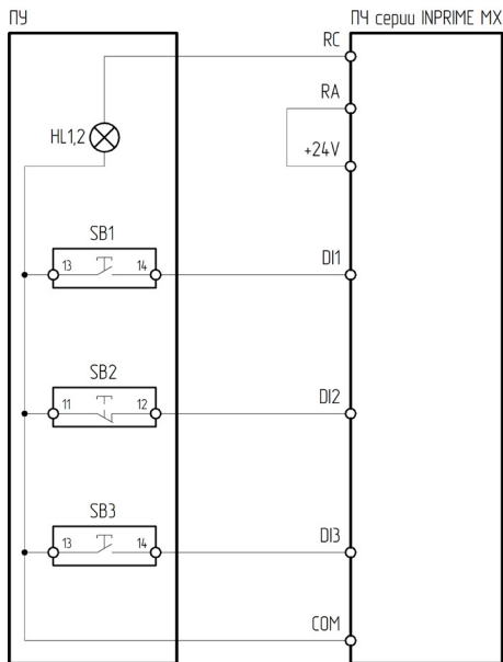
Рисунок 4.5.7 – Схема подключения ПУ-4-150, ПУ-4-450 к преобразователю частоты серии INPRIME MX
