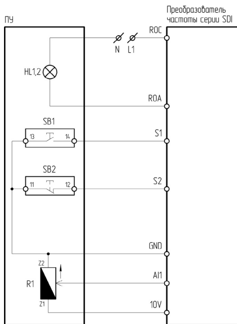
Рисунок 4.6.2 – Схема подключения ПУ-4-231, ПУ-4-531 к преобразователю частоты серии SDI
