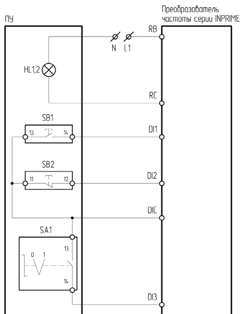
Рисунок 4.7.7 – Схема подключения ПУ-4-240, ПУ-4-540 к преобразователю частоты серии INPRIME
