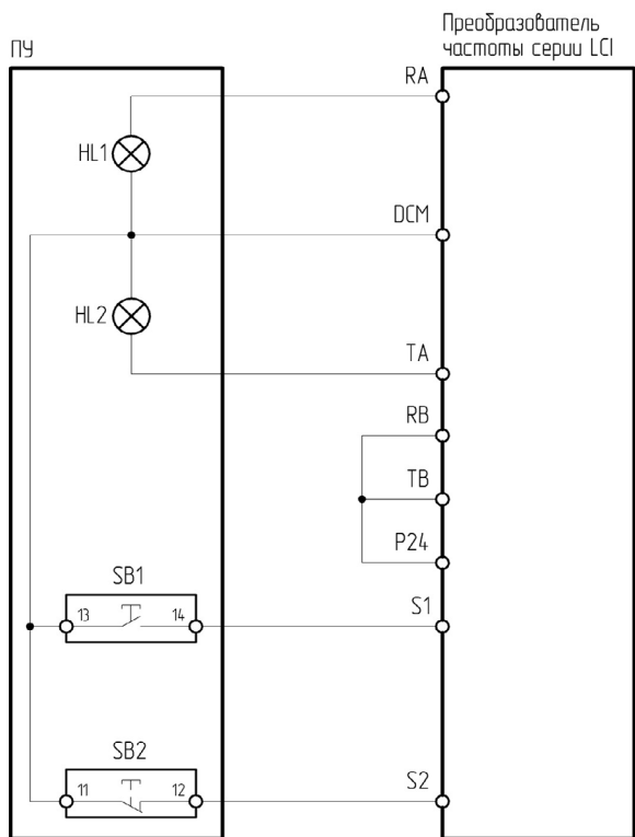
Рисунок 4.14.3 – Схема подключения ПУ-4-730 к преобразователю частоты серии LCI
