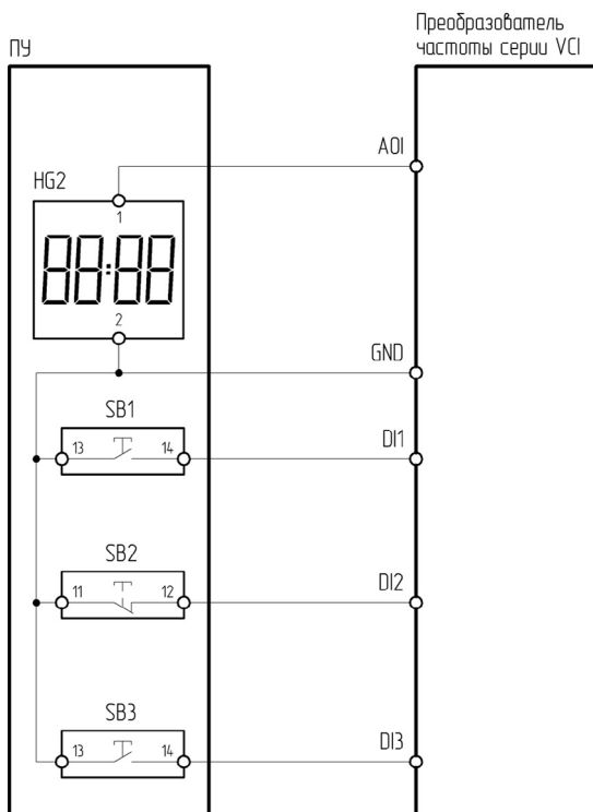
Рисунок 4.11.1 – Схема подключения ПУ-4-650 к преобразователю частоты серии VCI
