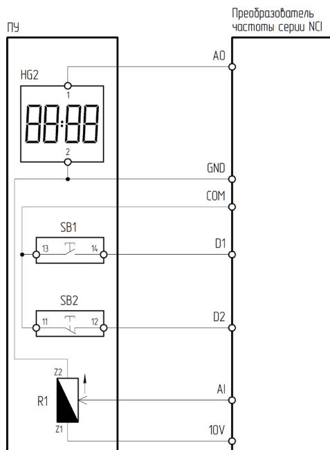
Рисунок 4.9.3 – Схема подключения ПУ-4-631 к преобразователю частоты серии NCI
