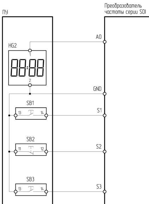
Рисунок 4.11.2 – Схема подключения ПУ-4-650 к преобразователю частоты серии SDI
