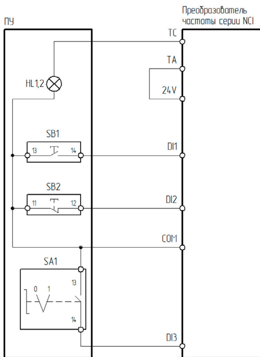
Рисунок 4.4.2 – Схема подключения ПУ-4-140, ПУ-4-440 к преобразователю частоты серии NCI
