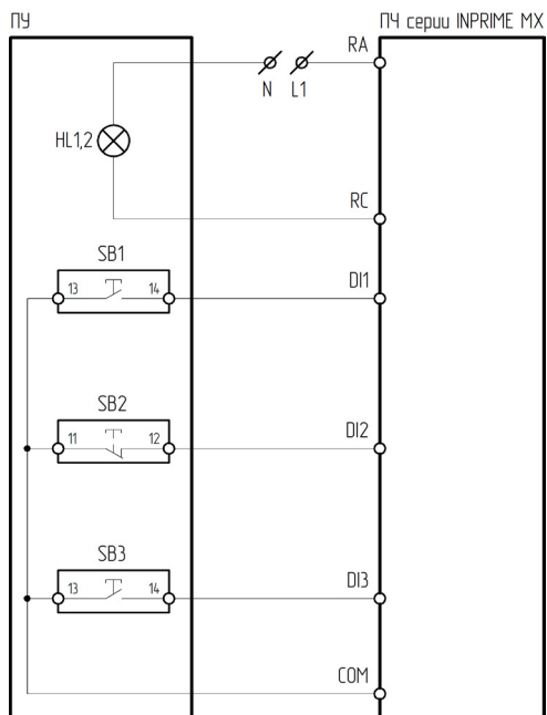
Рисунок 4.8.8 – Схема подключения ПУ-4-250, ПУ-4-550 к преобразователю частоты серии INPRIME MX
