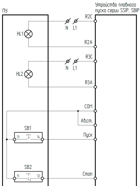
Рисунок 4.17.3 – Схема подключения ПУ-4-830 к устройству плавного пуска серии SSIP/SBIP
