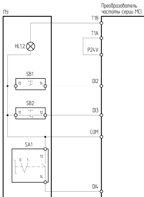
Рисунок 4.4.4 – Схема подключения ПУ-4-140, ПУ-4-440 к преобразователю частоты серии MCI
