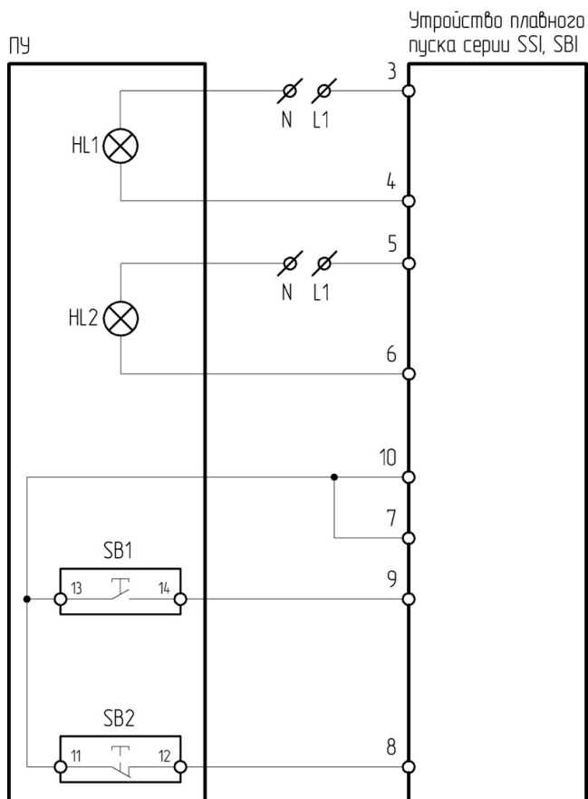
Рисунок 4.17.2 – Схема подключения ПУ-4-830 к устройству плавного пуска серии SSI/SBI
