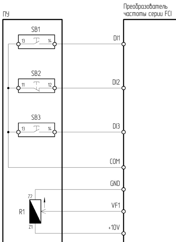
Рисунок 4.2.6 – Схема подключения ПУ-4-051 к преобразователю частоты серии FCI
