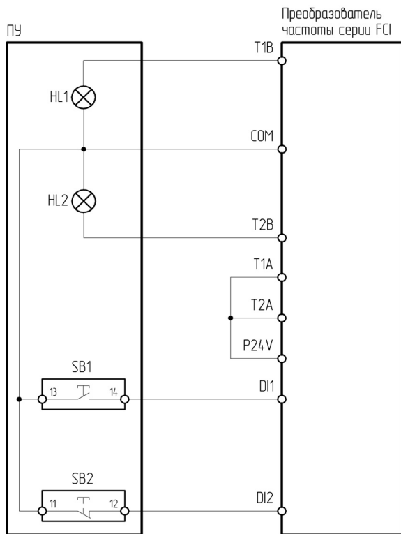
Рисунок 4.14.4 – Схема подключения ПУ-4-730 к преобразователю частоты серии FC1
