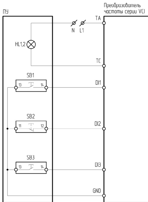
Рисунок 4.8.1 – Схема подключения ПУ-4-250, ПУ-4-550 к преобразователю частоты серии VCI
