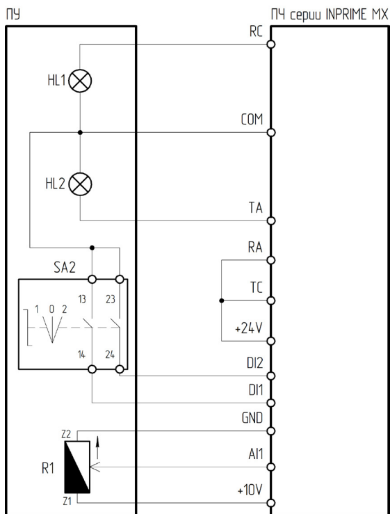
Рисунок 4.13.4 – Схема подключения ПУ-3-721 к преобразователю частоты серии INPRIME MX
