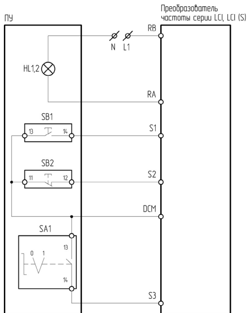
Рисунок 4.7.4 – Схема подключения ПУ-4-240, ПУ-4-540 к преобразователю частоты серии LCI/LCI(S)
