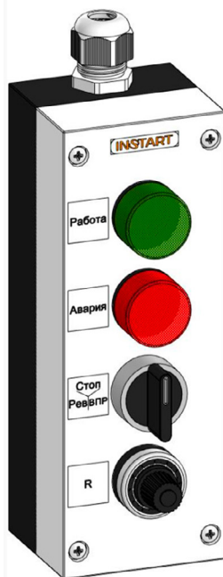
Рисунок 4.16 – Внешний вид ПУ-4-821
