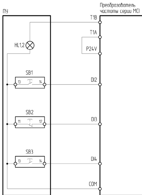
Рисунок 4.5.4 – Схема подключения ПУ-4-150, ПУ-4-450 к преобразователю частоты серии MCI
