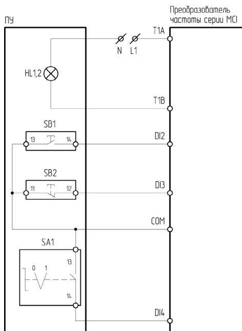
Рисунок 4.7.5 – Схема подключения ПУ-4-240, ПУ-4-540 к преобразователю частоты серии MCI
