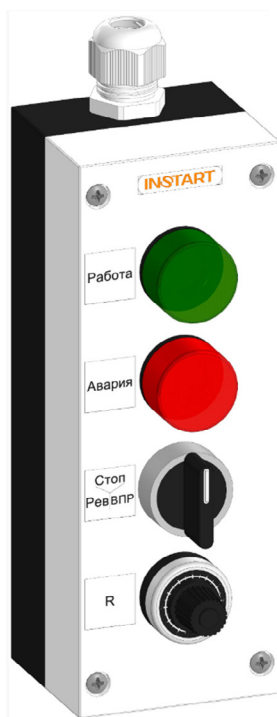
Рисунок 4.13 – Внешний вид ПУ-4-721
