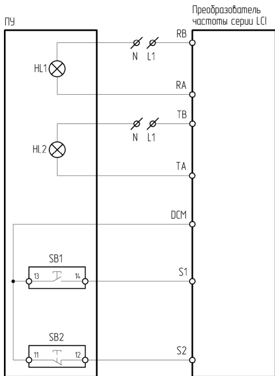
Рисунок 4.17.5 – Схема подключения ПУ-4-830 к преобразователю частоты серии LCI
