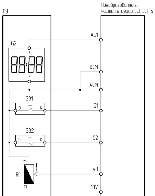
Рисунок 4.9.4 – Схема подключения ПУ-4-631 к преобразователю частоты серии LCI/LCI(S)
