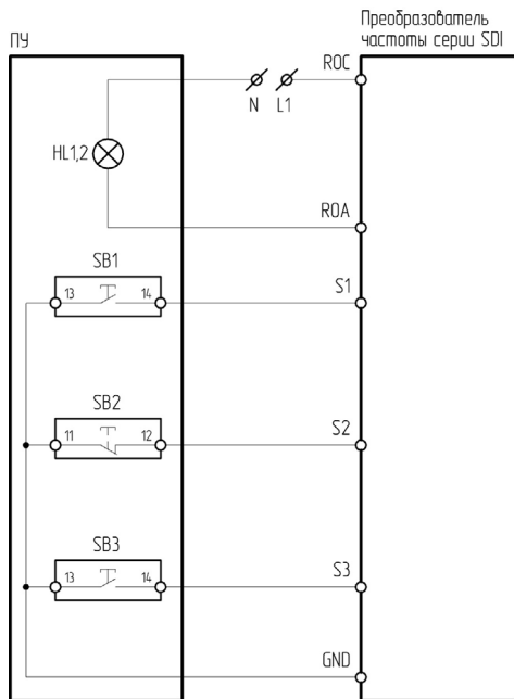
Рисунок 4.8.2 – Схема подключения ПУ-4-250, ПУ-4-550 к преобразователю частоты серии SDI
