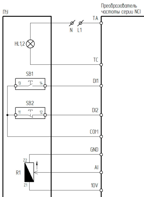
Рисунок 4.6.3 – Схема подключения ПУ-4-231, ПУ-4-531 к преобразователю частоты серии NCI
