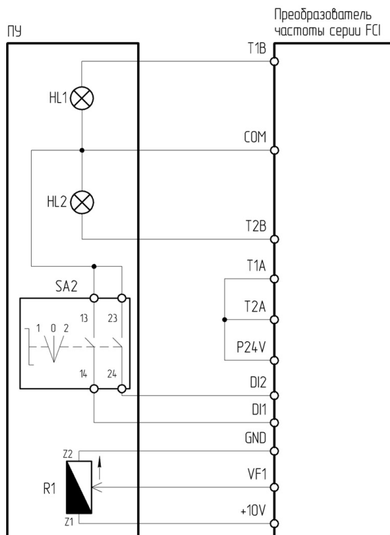
Рисунок 4.13.2 – Схема подключения ПУ-4-721 к преобразователю частоты серии FC1
