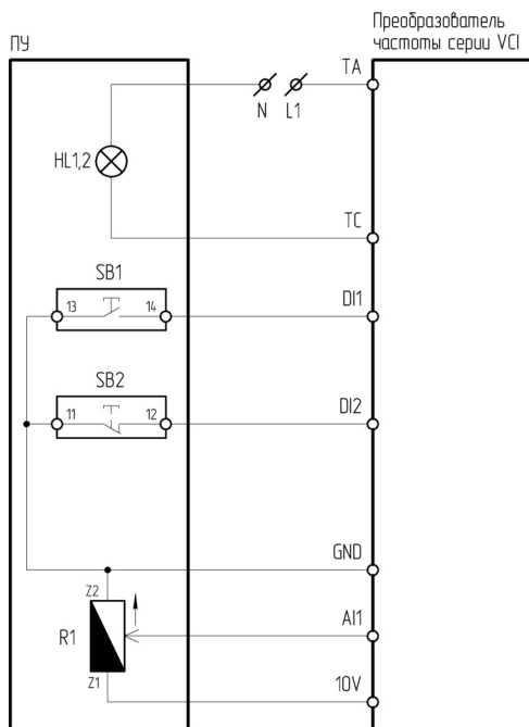
Рисунок 4.6.1 – Схема подключения ПУ-4-231, ПУ-4-531 к преобразователю частоты серии VCI
