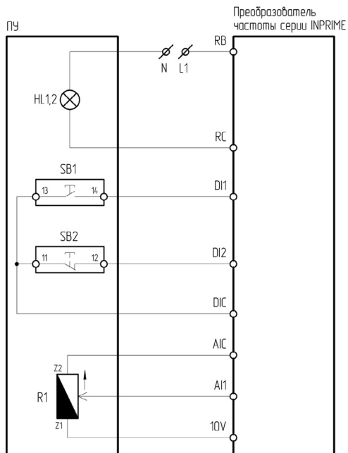
Рисунок 4.6.7 – Схема подключения ПУ-4-231, ПУ-4-531 к преобразователю частоты серии INPRIME
