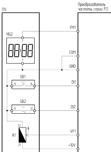
Рисунок 4.9.6 – Схема подключения ПУ-4-631 к преобразователю частоты серии FCI
