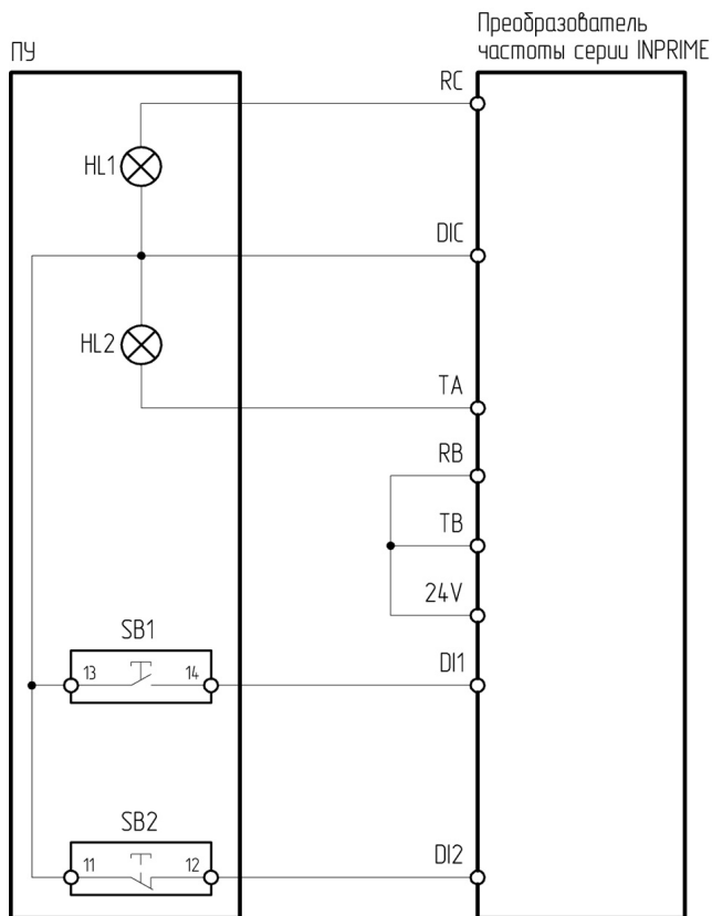
Рисунок 4.14.5 – Схема подключения ПУ-4-730 к преобразователю частоты серии INPRIME
