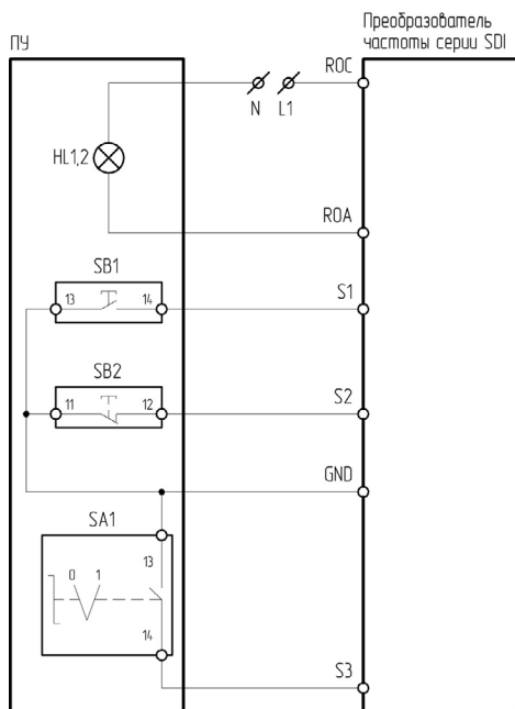
Рисунок 4.7.2 – Схема подключения ПУ-4-240, ПУ-4-540 к преобразователю частоты серии SDI
