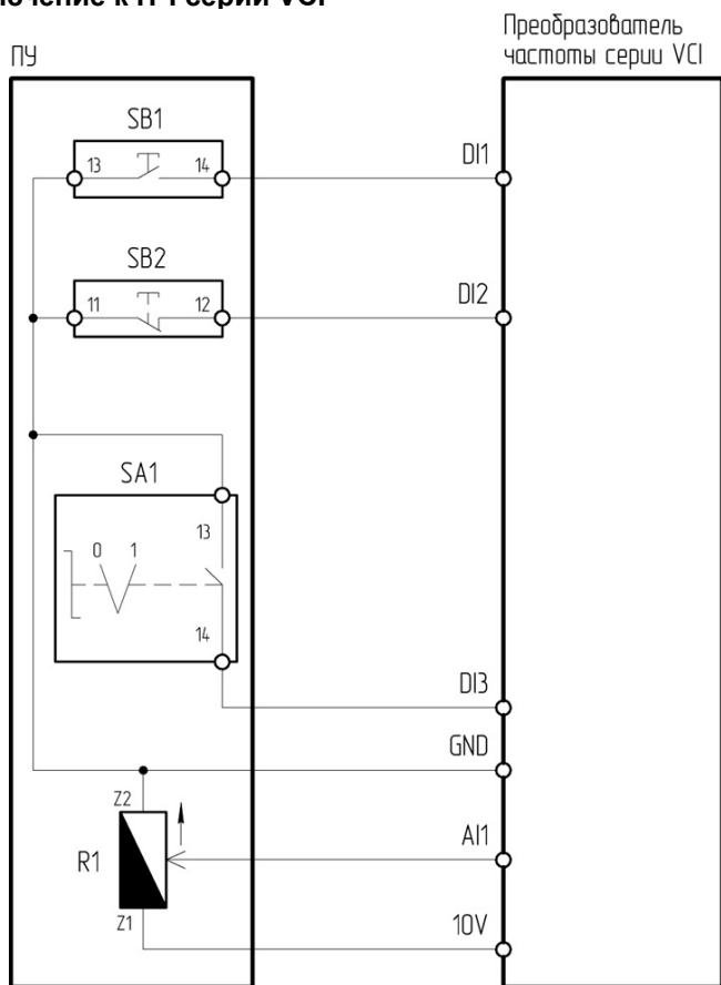
Рисунок 4.1.1 – Схема подключения ПУ-4-041 к преобразователю частоты серии VCI
