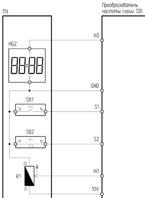
Рисунок 4.9.2 – Схема подключения ПУ-4-631 к преобразователю частоты серии SDI
