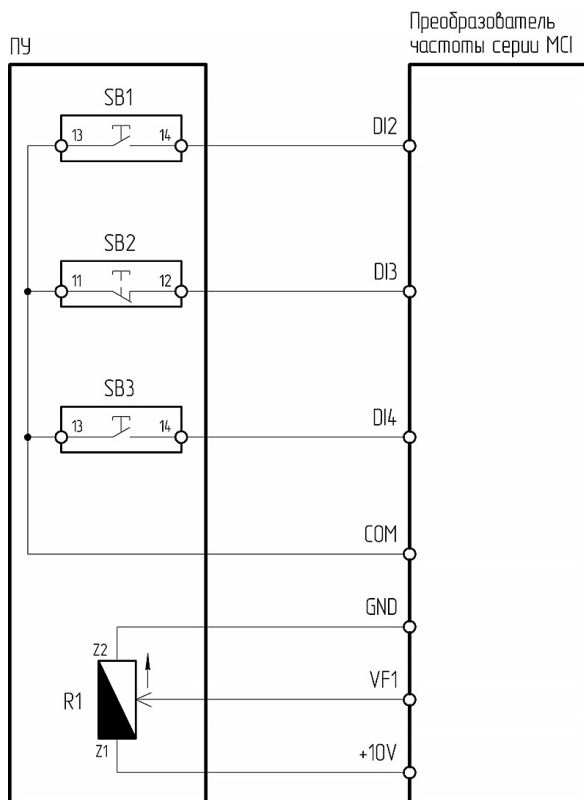
Рисунок 4.2.5 – Схема подключения ПУ-4-051 к преобразователю частоты серии МС1
