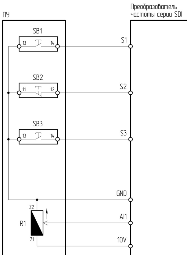
Рисунок 4.2.2 – Схема подключения ПУ-4-051 к преобразователю частоты серии SDI
