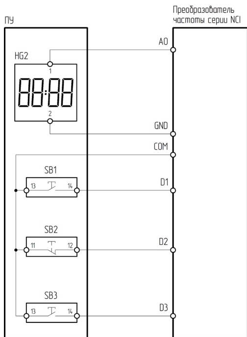
Рисунок 4.11.3 – Схема подключения ПУ-4-650 к преобразователю частоты серии NCI
