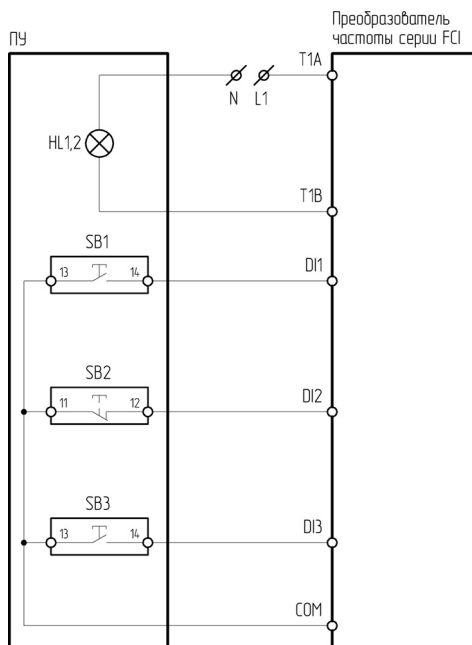
Рисунок 4.8.6 – Схема подключения ПУ-4-250, ПУ-4-550 к преобразователю частоты серии FCI
