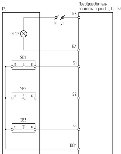
Рисунок 4.8.4 – Схема подключения ПУ-4-250, ПУ-4-550 к преобразователю частоты серии LCI/LCI(S)
