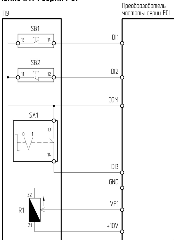
Рисунок 4.1.6 – Схема подключения ПУ-4-041 к преобразователю частоты серии FCI
