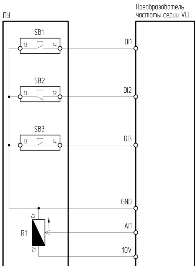
Рисунок 4.2.1 – Схема подключения ПУ-4-051 к преобразователю частоты серии VCI
