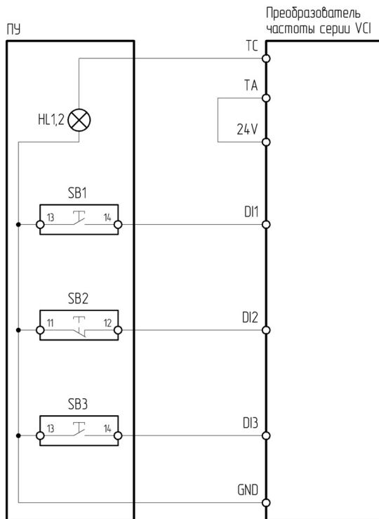
Рисунок 4.5.1 – Схема подключения ПУ-4-150, ПУ-4-450 к преобразователю частоты серии VCI
