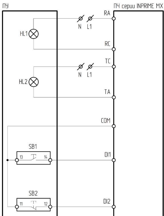
Рисунок 4.17.8 – Схема подключения ПУ-4-830 к преобразователю частоты серии INPRIME MX
