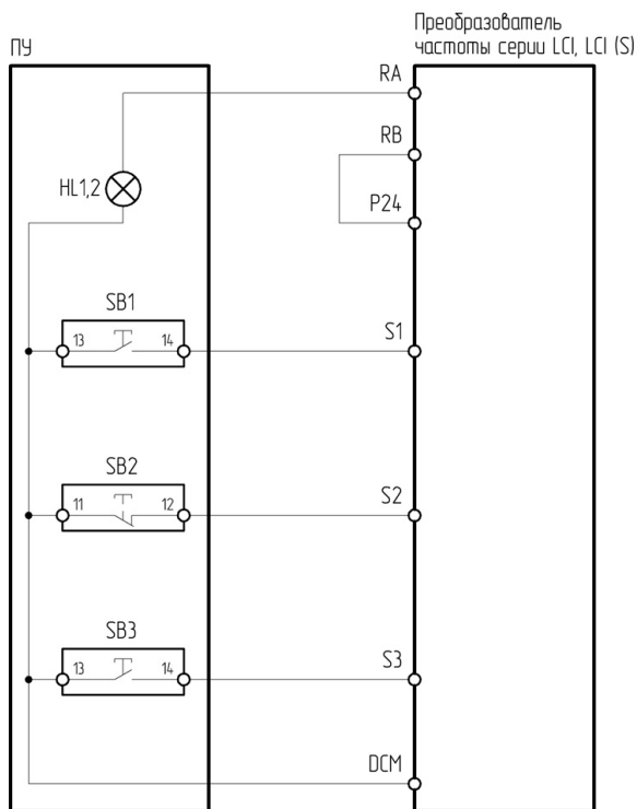
Рисунок 4.5.3 – Схема подключения ПУ-4-150, ПУ-4-450 к преобразователю частоты серии LCI/LCI(S)
