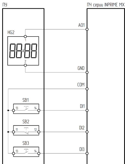
Рисунок 4.11.8 – Схема подключения ПУ-4-650 к преобразователю частоты серии INPRIME MX
