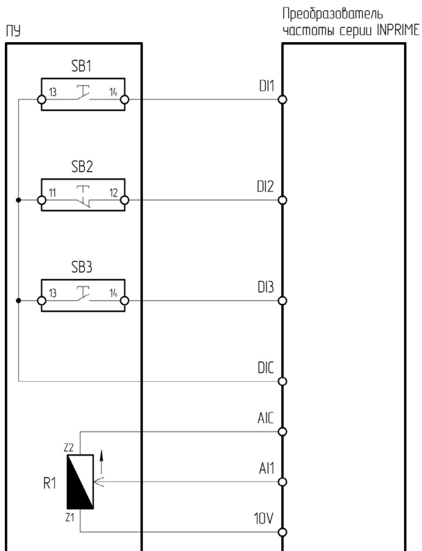
Рисунок 4.2.7 – Схема подключения ПУ-4-051 к преобразователю частоты серии INPRIME
