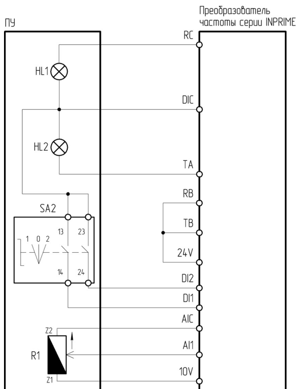
Рисунок 4.13.3 – Схема подключения ПУ-4-721 к преобразователю частоты серии INPRIME
