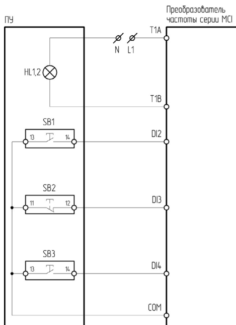
Рисунок 4.8.5 – Схема подключения ПУ-4-250, ПУ-4-550 к преобразователю частоты серии MCI
