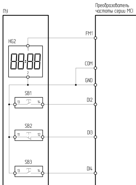
Рисунок 4.11.5 – Схема подключения ПУ-4-650 к преобразователю частоты серии MCI
