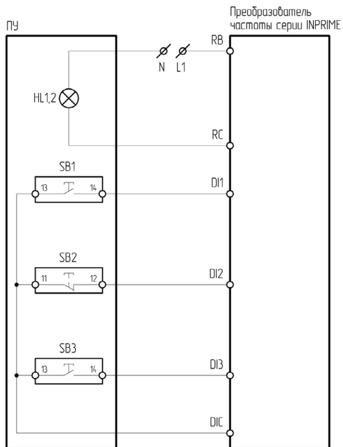
Рисунок 4.8.7 – Схема подключения ПУ-4-250, ПУ-4-550 к преобразователю частоты серии INPRIME
