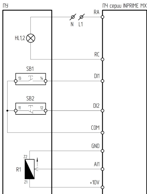
Рисунок 4.6.9 – Схема подключения ПУ-4-231, ПУ-4-531 к преобразователю частоты серии INPRIME MX
