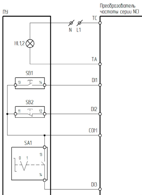
Рисунок 4.7.3 – Схема подключения ПУ-4-240, ПУ-4-540 к преобразователю частоты серии NCI
