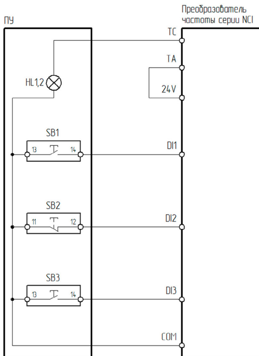
Рисунок 4.5.2 – Схема подключения ПУ-4-150, ПУ-4-450 к преобразователю частоты серии NCI
