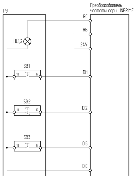
Рисунок 4.5.6 – Схема подключения ПУ-4-150, ПУ-4-450 к преобразователю частоты серии INPRIME
