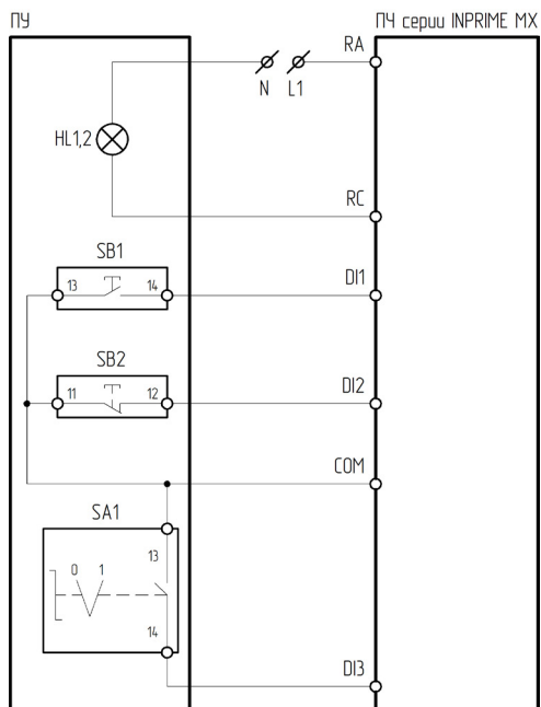
Рисунок 4.7.8 – Схема подключения ПУ-4-240, ПУ-4-540 к преобразователю частоты серии INPRIME MX
