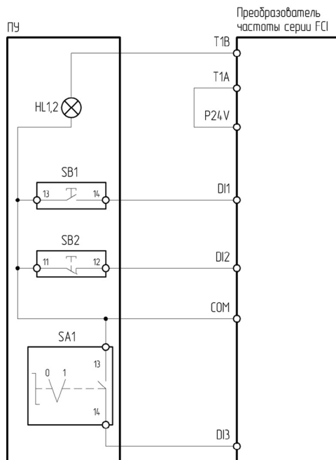
Рисунок 4.4.5 – Схема подключения ПУ-4-140, ПУ-4-440 к преобразователю частоты серии FCI
