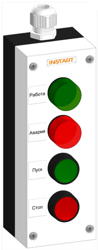
Рисунок 4.14 – Внешний вид ПУ-4-730
