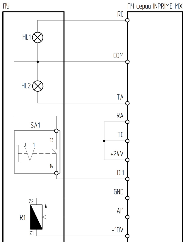
Рисунок 4.12.4 – Схема подключения ПУ-4-711 к преобразователю частоты серии INPRIME MX
