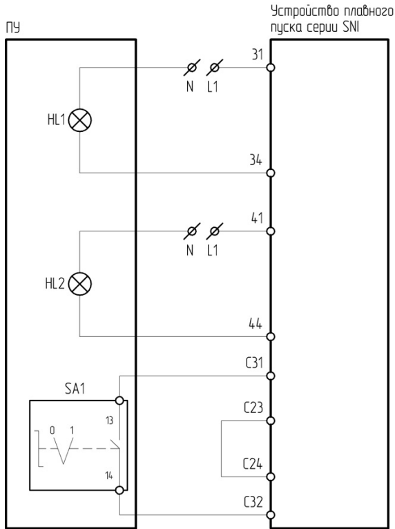
Рисунок Рисунок 4.17.4 – Схема подключения ПУ-4-830 к устройству плавного пуска серии SNI
