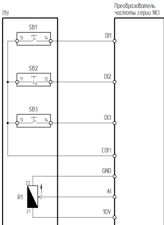
Рисунок 4.2.3 – Схема подключения ПУ-4-051 к преобразователю частоты серии NCI
