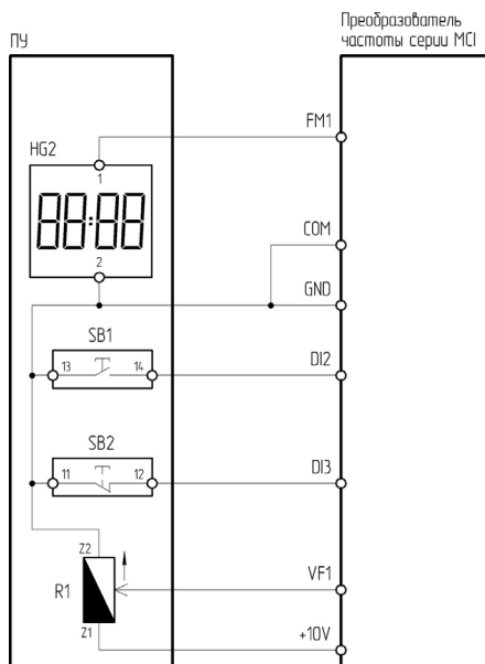
Рисунок 4.9.5 – Схема подключения ПУ-4-631 к преобразователю частоты серии МС1
