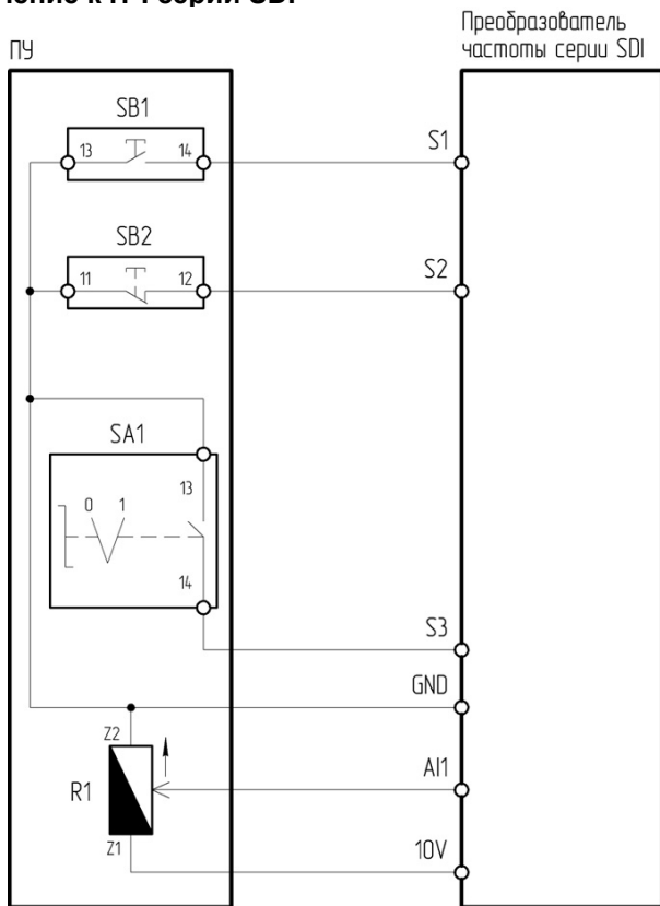
Рисунок 4.1.2 – Схема подключения ПУ-4-041 к преобразователю частоты серии SDI
