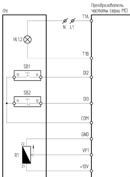
Рисунок 4.6.5 – Схема подключения ПУ-4-231, ПУ-4-531 к преобразователю частоты серии МС1
