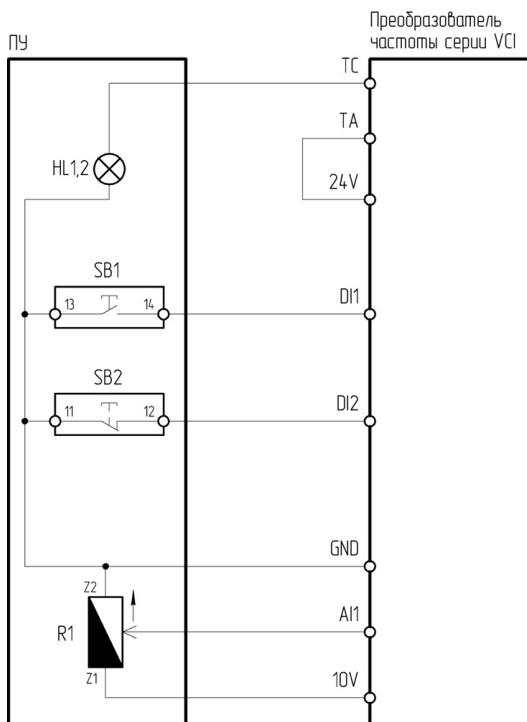
Рисунок 4.3.1 – Схема подключения ПУ-4-131, ПУ-4-431 к преобразователю частоты серии VCI
