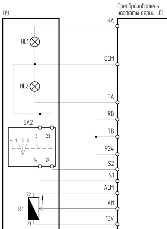
Рисунок 4.13.1 – Схема подключения ПУ-4-721 к преобразователю частоты серии LCI
