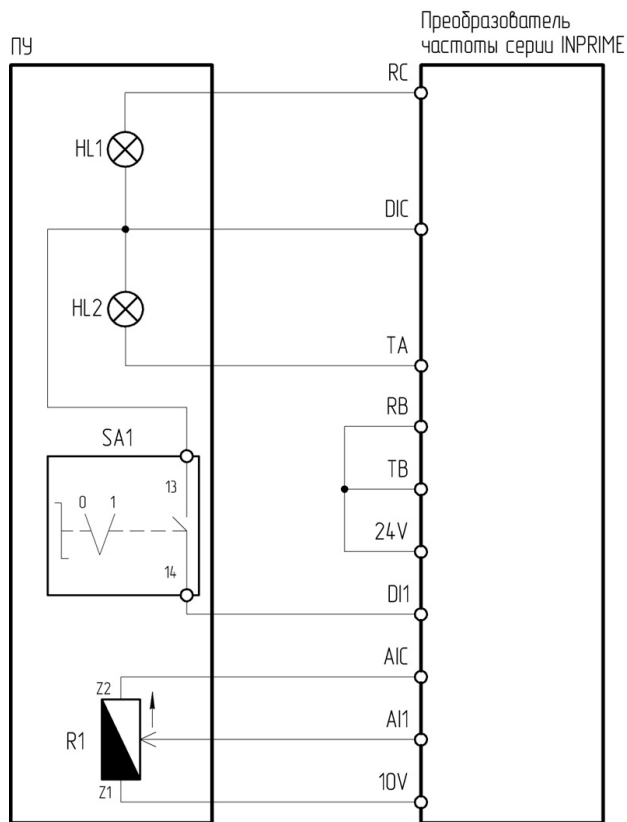
Рисунок 4.12.3 – Схема подключения ПУ-4-711 к преобразователю частоты серии INPRIME
