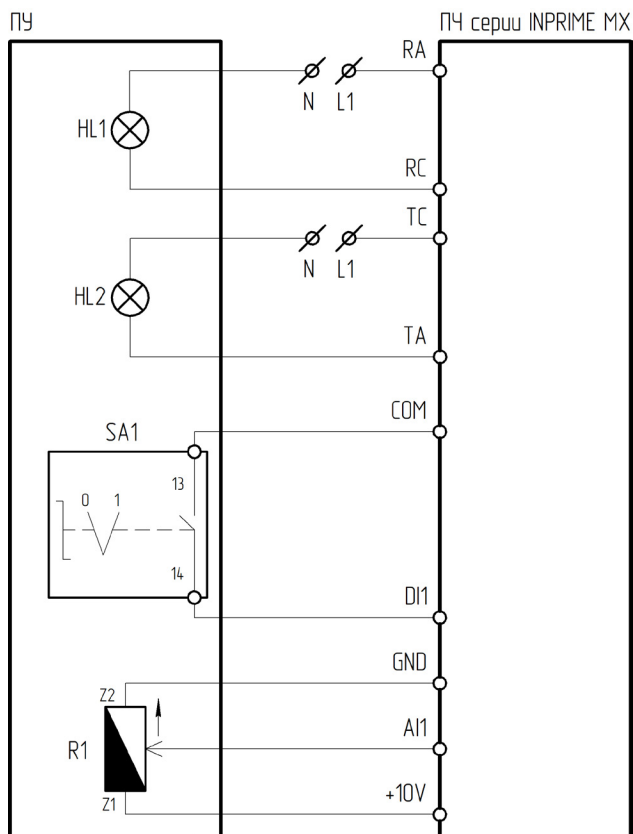
Рисунок 4.15.4 – Схема подключения ПУ-4-811 к преобразователю частоты серии INPRIME MX
