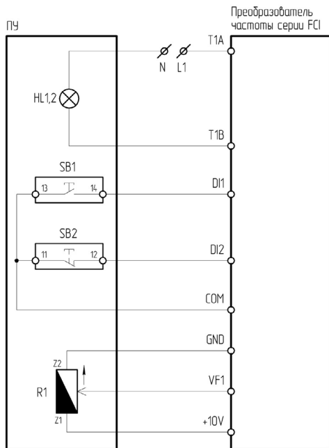
Рисунок 4.6.6 – Схема подключения ПУ-4-231, ПУ-4-531 к преобразователю частоты серии FCI
