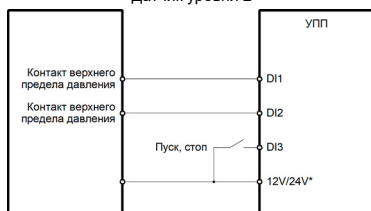
Датчик уровня 2
