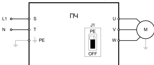
Рисунок 3.2 – Схема силовых подключений для моделей INVENT-GY-2
