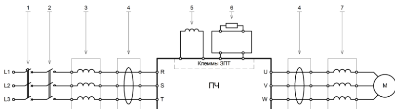
Рисунок 3.4 – Схема подключения дополнительного оборудования
