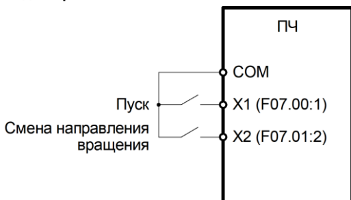
Рисунок 6.13 – Схема двухпроводного подключения 2
