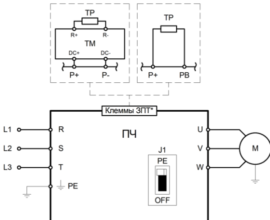
Рисунок 3.3 – Схема силовых подключений для моделей INVENT-GY-4(B)
