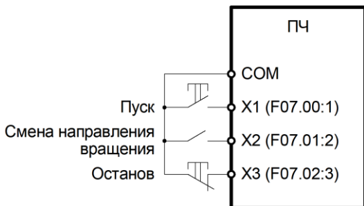
Рисунок 6.15 – Схема трехпроводного подключения 2
