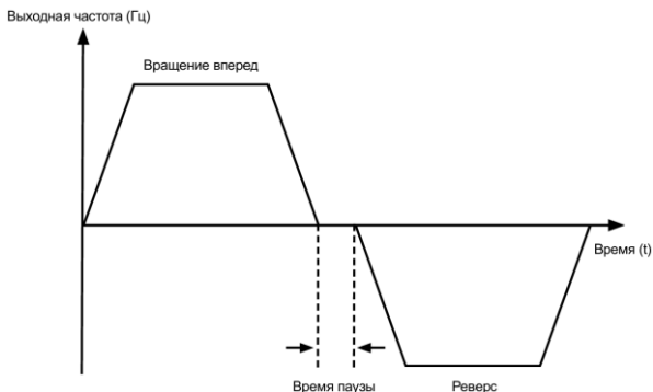
Рисунок 6.6 – Время паузы при смене направления вращения
