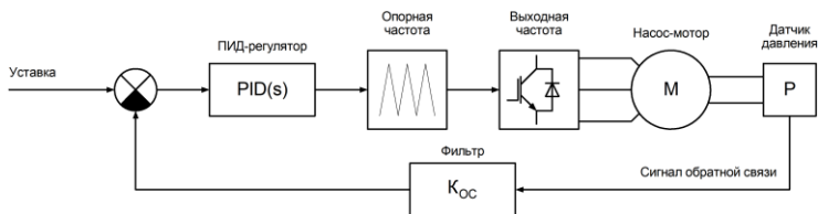
Рисунок 6.16 – Схема ПИД-регулирования
