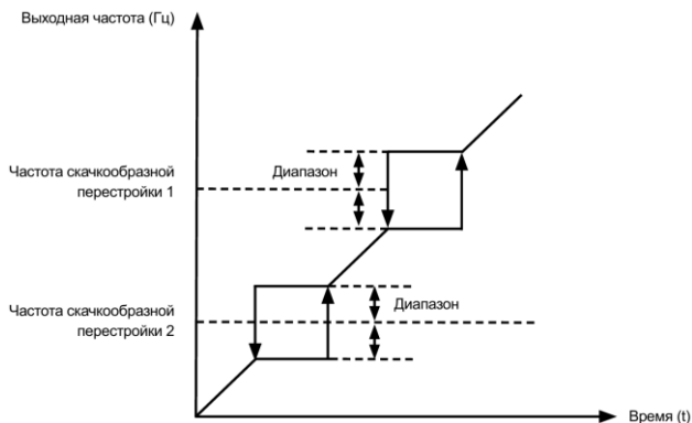
Рисунок 6.5 – Принцип работы функции скачкообразной перестройки
