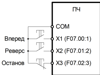
Рисунок 6.14 – Схема трехпроводного подключения 1
