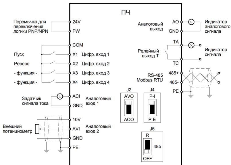
Рисунок 3.6 – Схема подключения управляющих клемм серии INVENT
