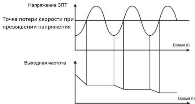
Рисунок 6.19 – Иллюстрация работы защиты от перенапряжения
