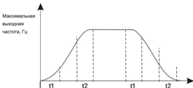
Рисунок 6.3 – S-образная кривая ускорения и замедления
