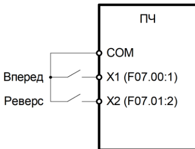
Рисунок 6.12 – Схема двухпроводного подключения 1
