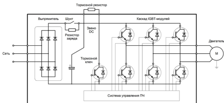
Рисунок 2.1 – Принципиальная электрическая схема устройства трехфазных моделей INVENT со встроенным тормозным модулем
