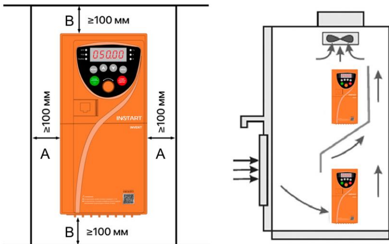
Рисунок 3.1 – Схема установки ПЧ серии INVENT
