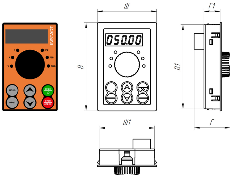
Рисунок 5.2 – Выносная панель управления INVENT-KP
