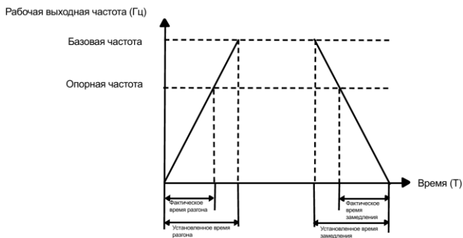
Рисунок 6.2 – Время разгона/замедления
