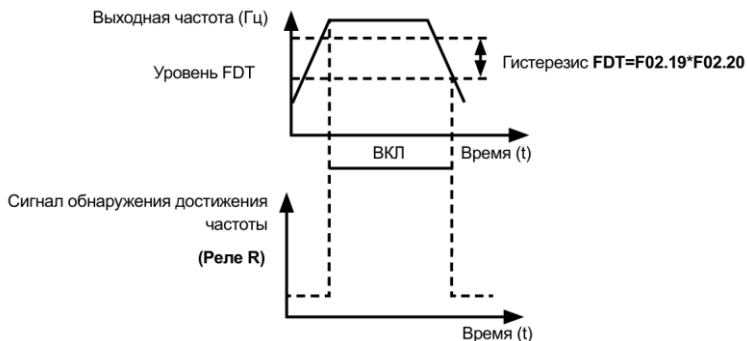
Рисунок 6.7 – Значение обнаружения выходной частоты
