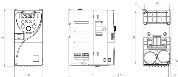
Рисунок 2.3 – Внешний вид моделей ПЧ серии INVENT
