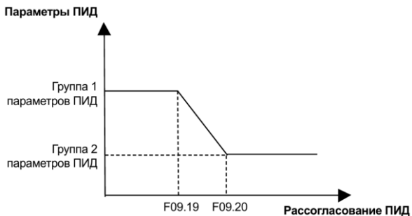
Рисунок 6.17 – Переключение параметров ПИД
