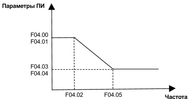
Рисунок 6.9 – Зависимость параметров ПИ от частоты
