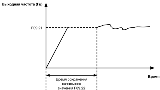
Рисунок 6.18 – Время сохранения опорного значения
