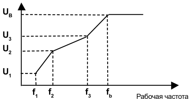
Рисунок 6.11 – Ломанная характеристика U/f
