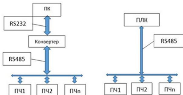
Рисунок. 7.2 - Сетевой режим Master/Slaves
