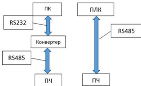
Рисунок 7.1 – Сетевой режим Master/Slave
