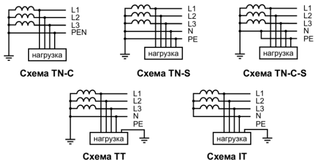
Рисунок 3.8 – Типы систем заземления
