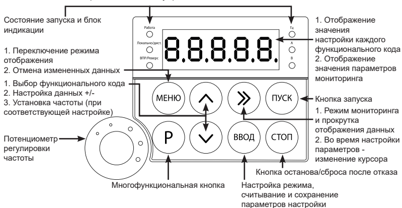
Рисунок 4 – Описание встроенной панели управления
