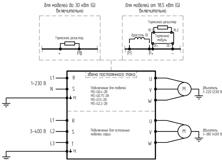
Рис. 2 – Подключение силовых клемм
