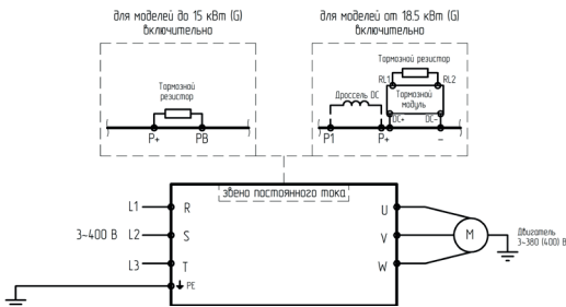
Рис. 2 – Подключение силовых клемм
