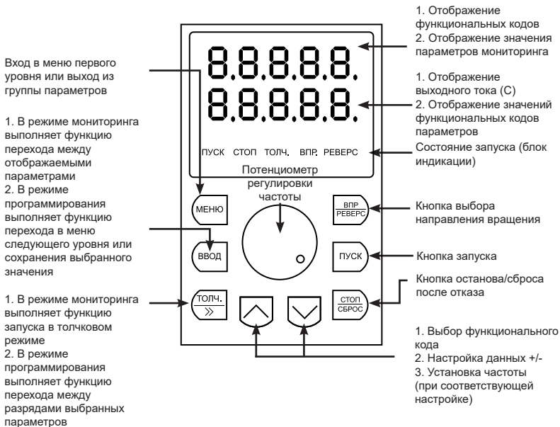
Рисунок 7 – Описание панели управления LCI-KP
