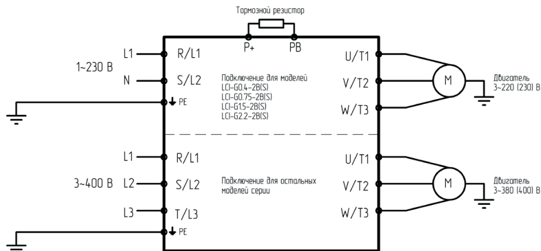
Рисунок 2 – Подключение силовых клемм для преобразователя частоты серии LCI(S)
