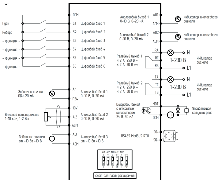
Рисунок 5 – Подключение управляющих клемм для преобразователя частоты серии LC1
