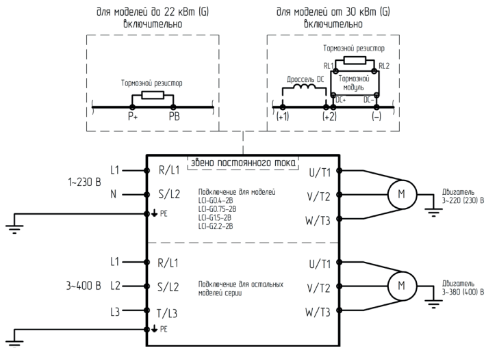
Рисунок 3 – Подключение силовых клемм для преобразователя частоты серии LCI
