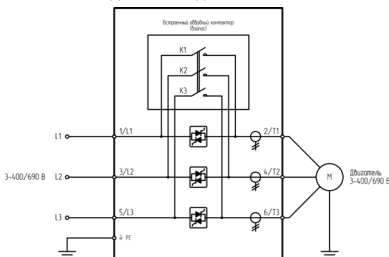
Рисунок 2 – Подключение силовых клемм
