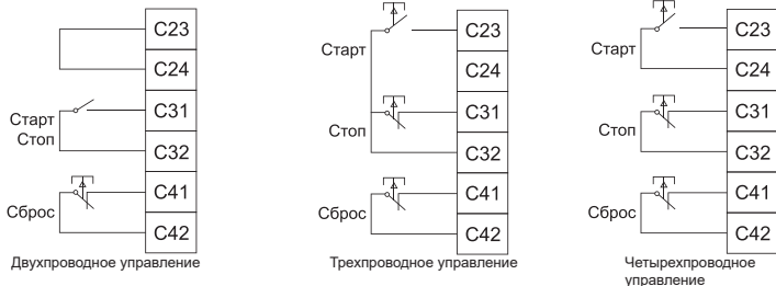
Рисунок 3 – Схемы управления
