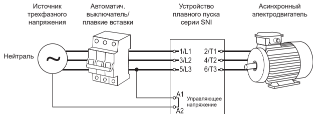
Рисунок 1 – Дополнительное оборудование
