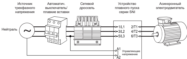
Рисунок 1 – Дополнительное оборудование
