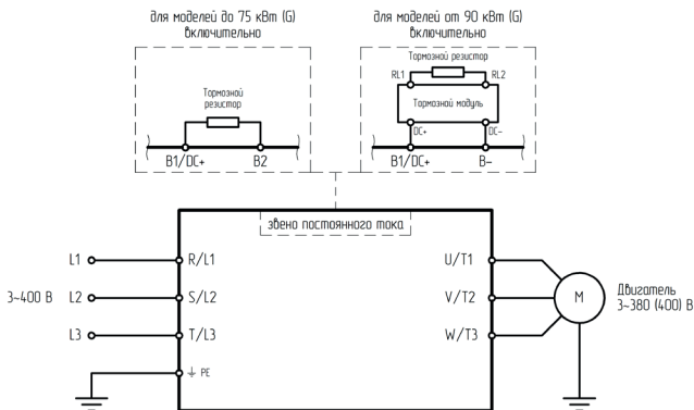
Рисунок 2 – Подключение силовых клемм для преобразователя частоты серии INPRIME
