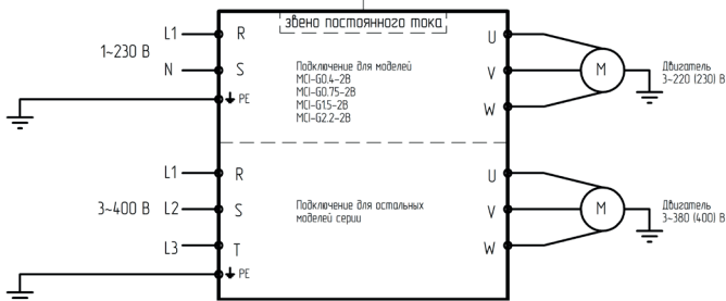
Рис. 2 – Подключение силовых клемм
