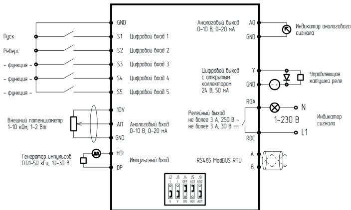
Рисунок 3 – Подключение управляющих клемм
