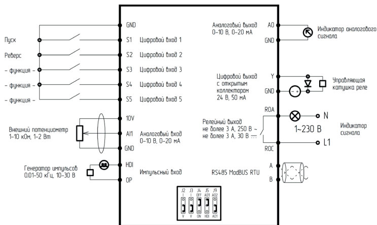
Рисунок 3 – Подключение управляющих клемм
