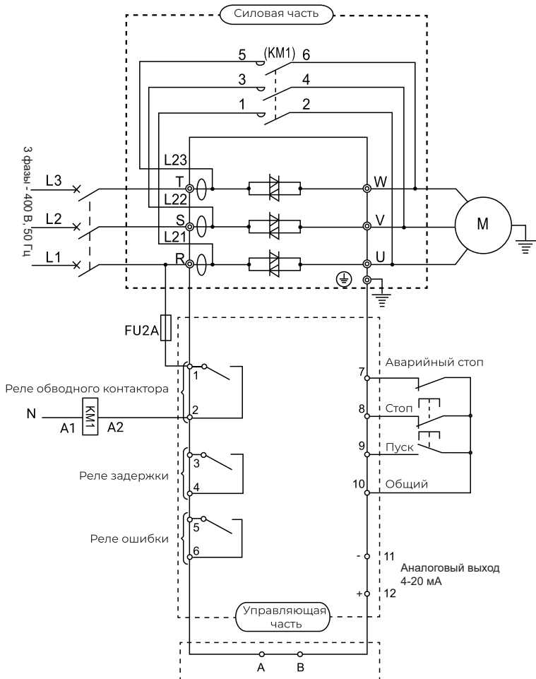
Рисунок 3 – Схема подключения клемм устройства плавного пуска серии SS1
