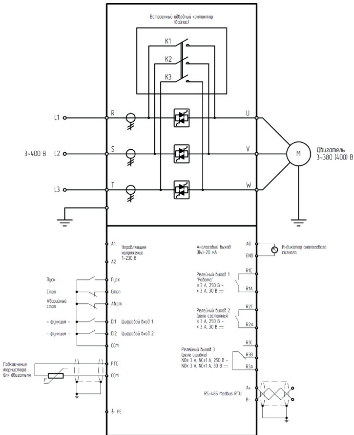
Рисунок 4 – Схема подключения клемм устройства плавного пуска серии SBIP
