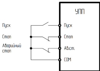
Рисунок 5 – Трехпроводная и двухпроводная схема управления
